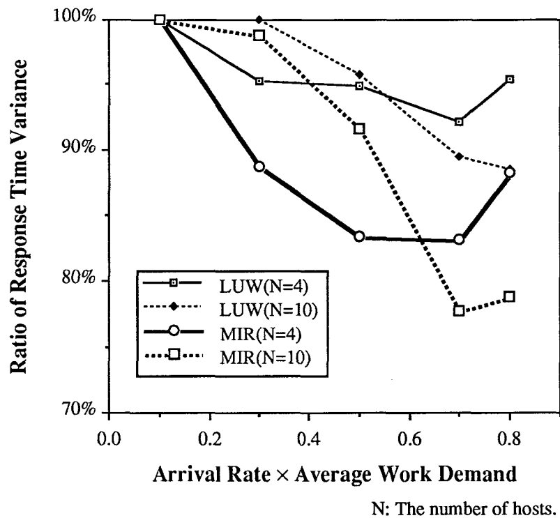
図 3.3: JSQ に対する他の尺度の応答時間の分散の比率
