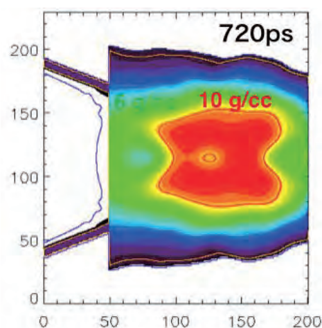
図 3 シミュレーション初期プラズマ密度。実験の最大圧縮時（爆縮レーザー照射後 720ps）の密度から設定。中心はおおよそ固体の 10 倍に圧縮されている。
