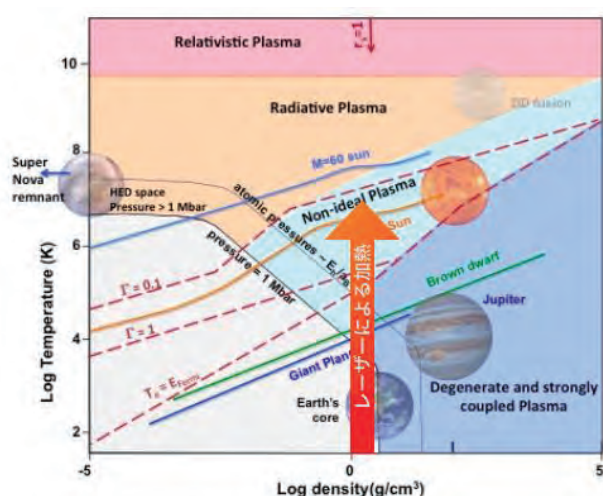
図1 密度と温度のマップ。固体( \sim 1 \text{ g/cm}^3 )を高強度レーザーで1000万度以上に瞬間的に加熱する。生成されたプラズマのエネルギー密度は太陽の内部状態と同じである。
