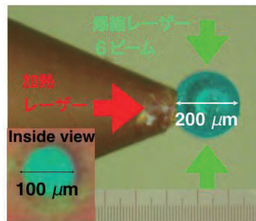
図 2 金コーンに取り付けられた球ターゲット。この球ターゲットを激光レーザー 6 ビームで爆縮する。その後、コーン内側から加熱ビームを照射し加熱する。
