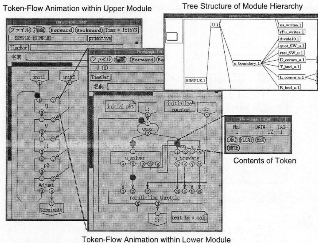
図 4.7 Qv-x の視覚的プログラミング支援環境の使用例
