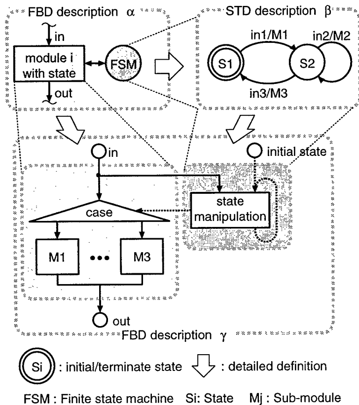
図 3.4 状態遷移処理の多面的図的仕様記述手法
