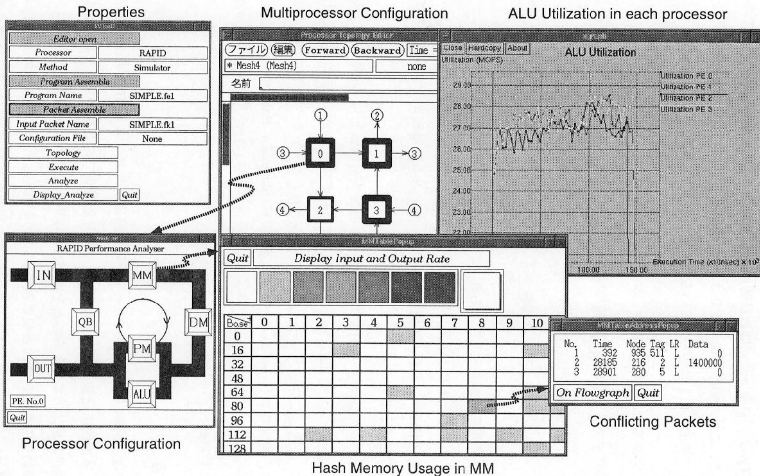
図 4.8 Qv-x マルチプロセッサの視覚的評価支援環境の使用例
