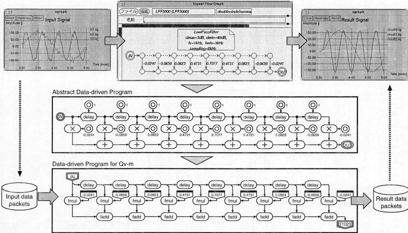
図 5.8 プロトタイプ環境の適用例
