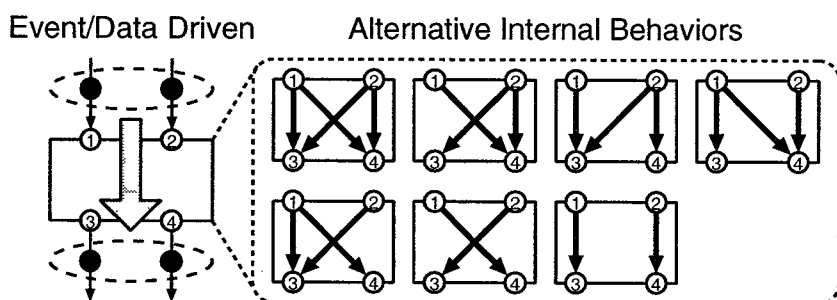
図 4.1 モジュールの振舞いの多様性
