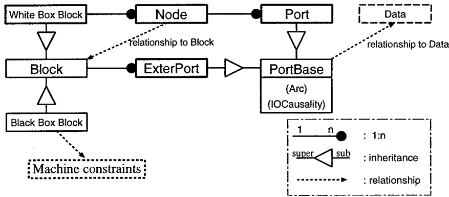
図 5.2 中間形式の機能構造情報
