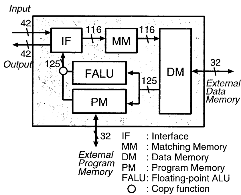
図 4.4 動的データ駆動型 VLSI プロセッサ Qv-m の基本構成
