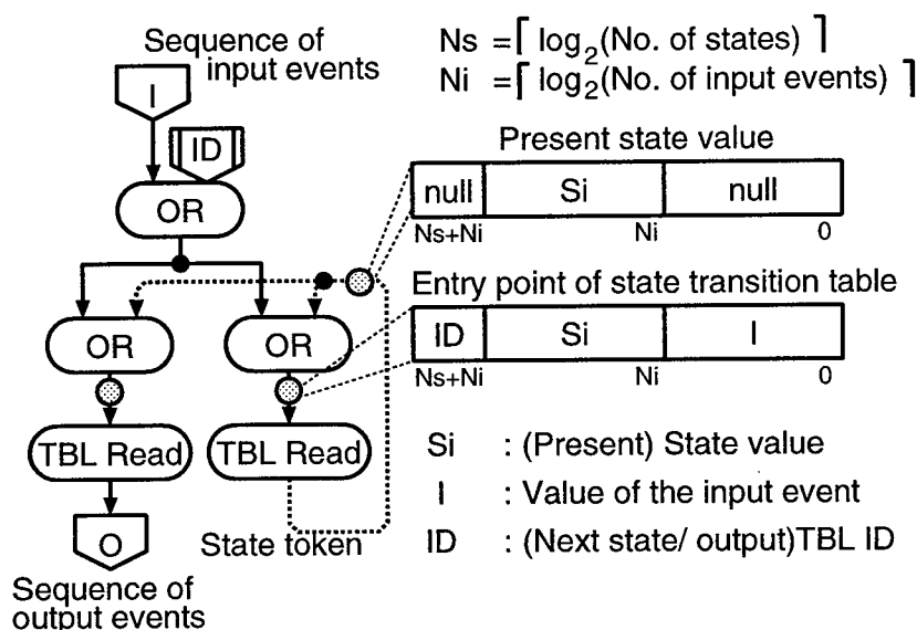
図 3.5 FSM の抽象データ駆動型プログラム構造
