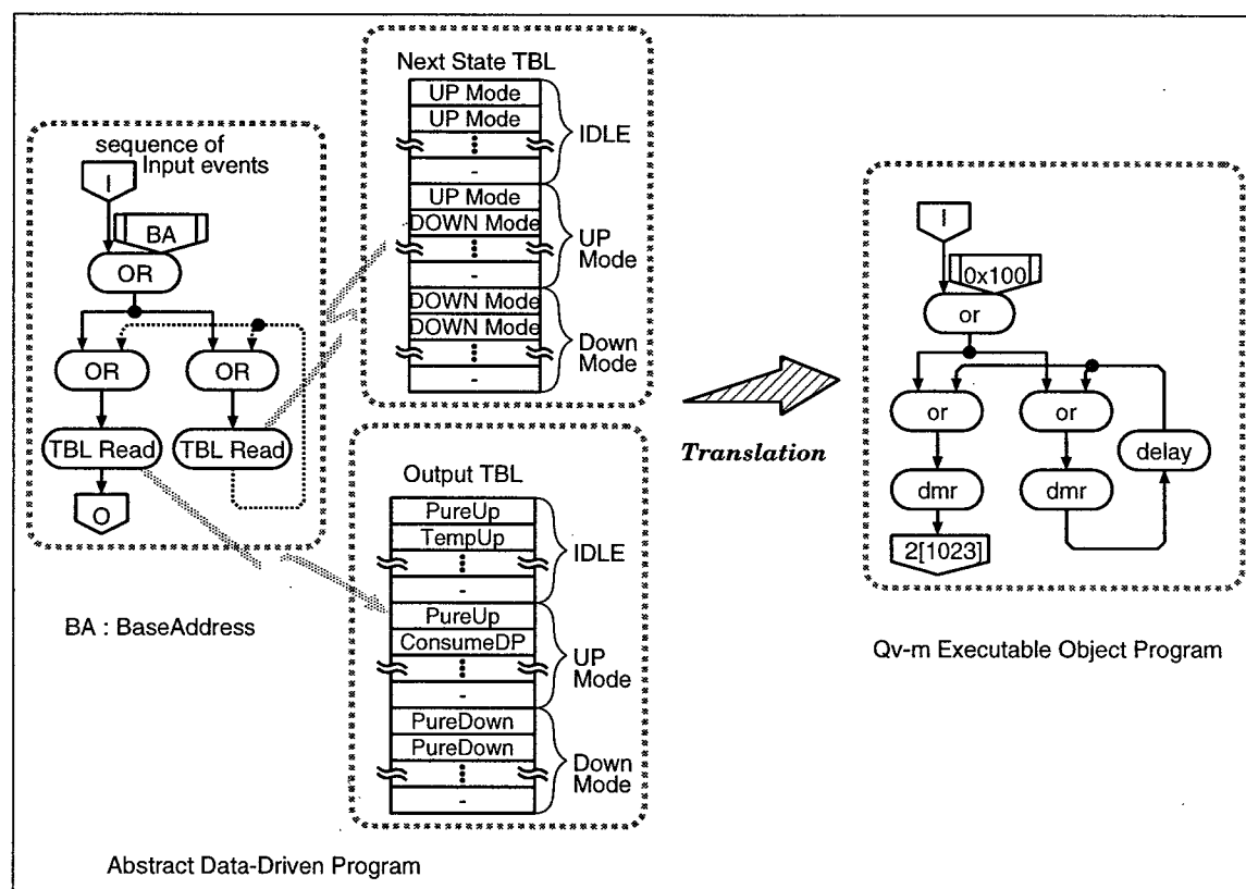
図 5.10 リフト制御問題における状態遷移動作の変換例
