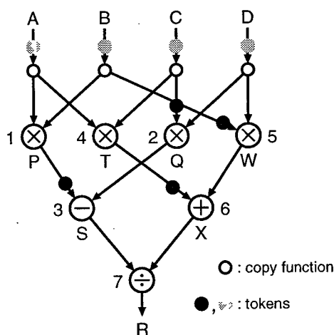
図 2.5 動的データ駆動型処理方式
