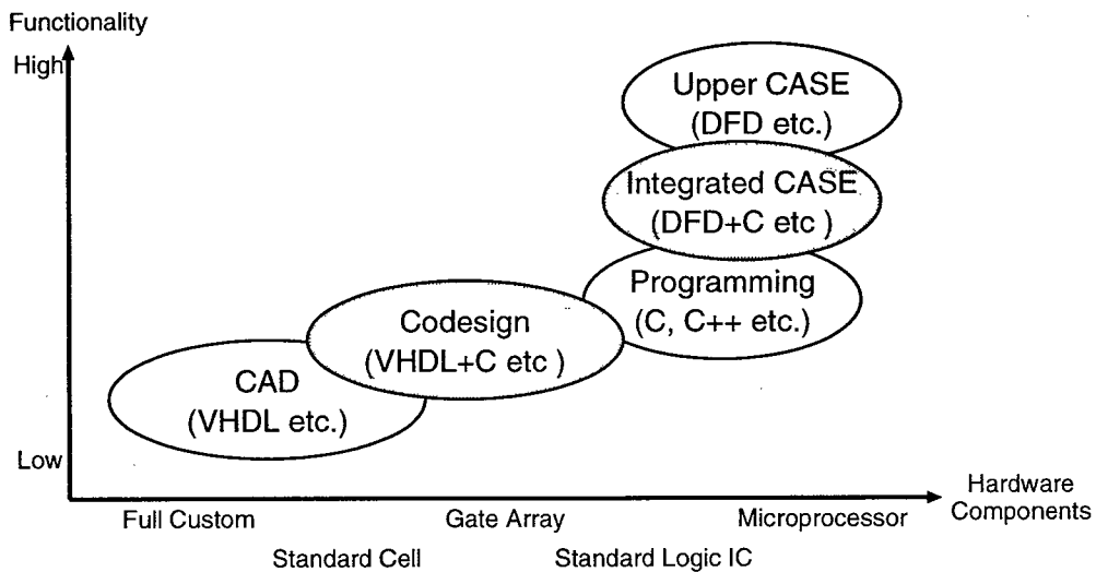
図 2.1 現状のシステム開発環境
