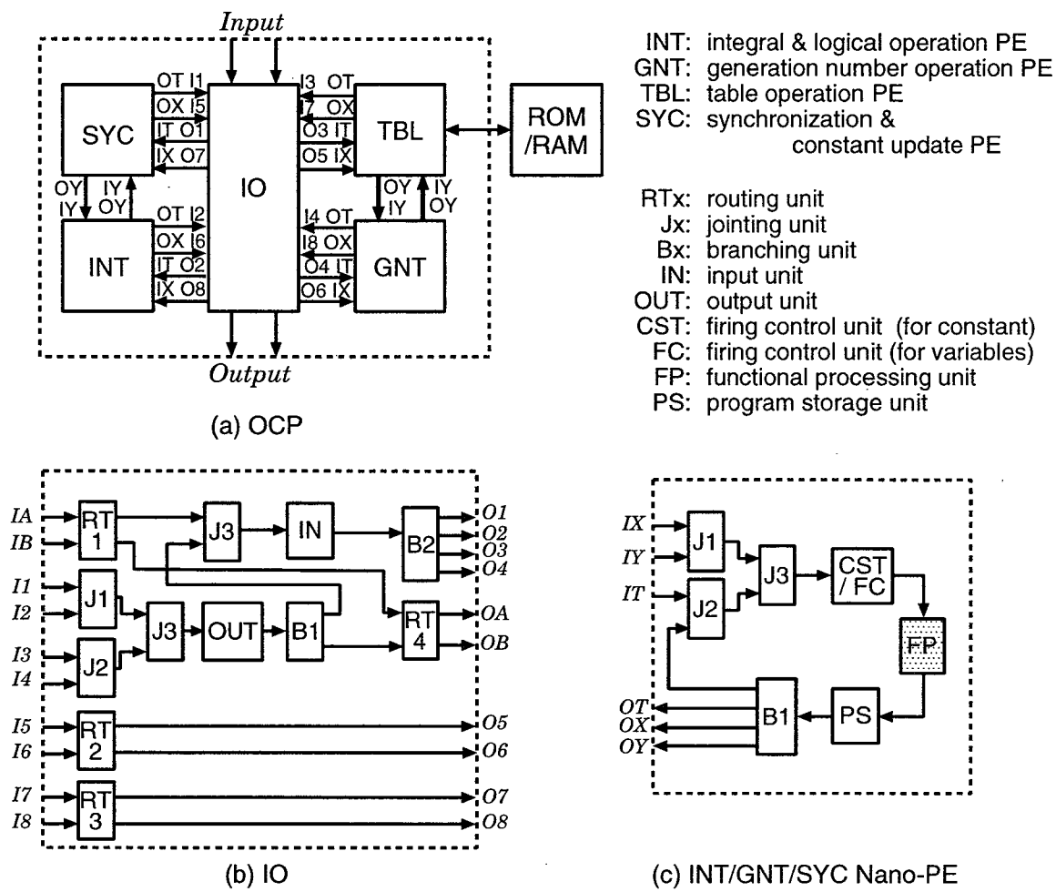
図 2.7 データ駆動型 VLSI プロセッサ Qv-s の構成
