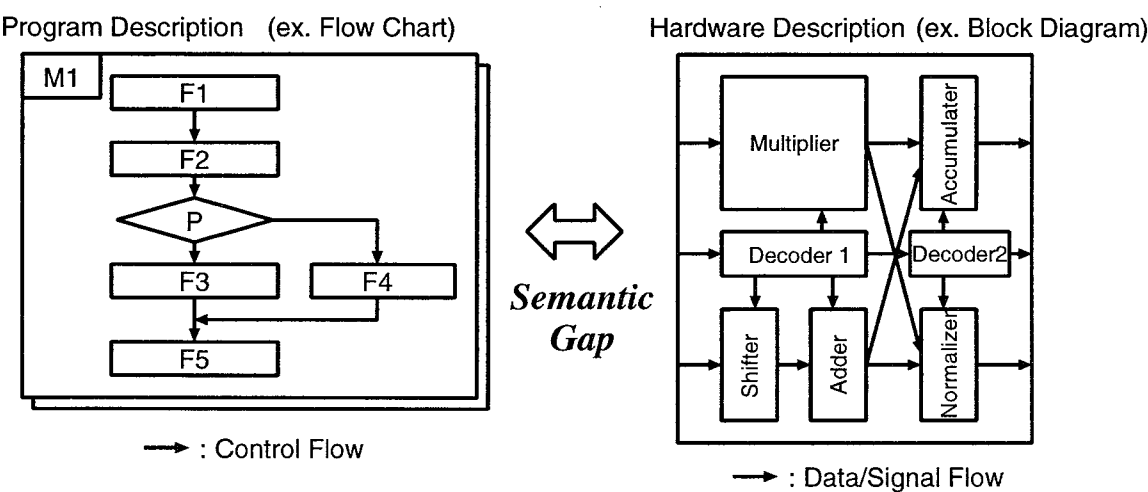
図 2.3 逐次代入型プログラム記述とハードウェア記述
