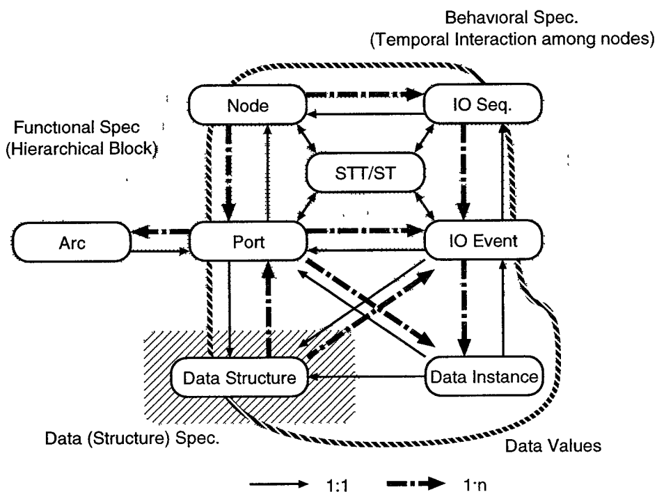
図 4.2 中間形式の各要素間の対応関係
