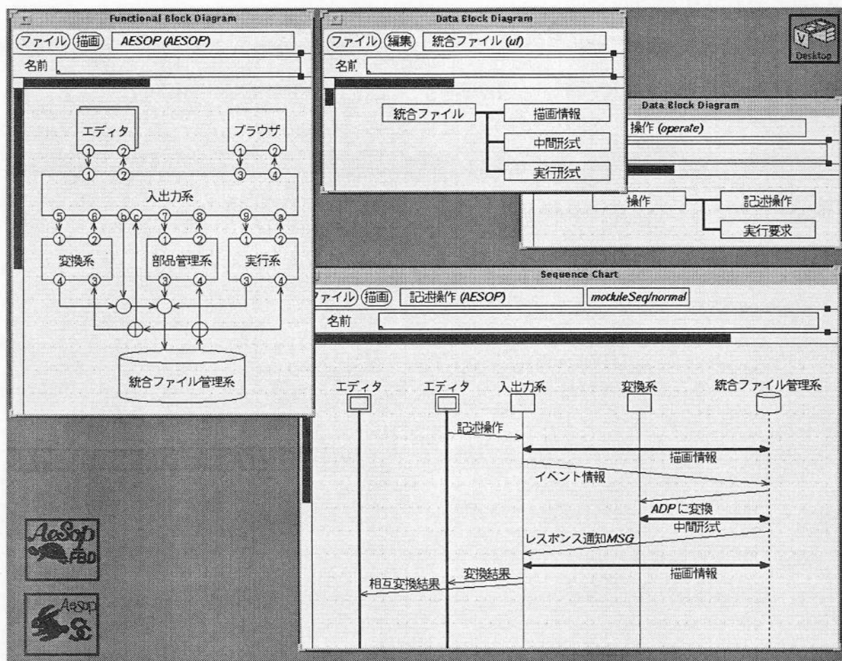
図 5.1 AESOP の機能構成
