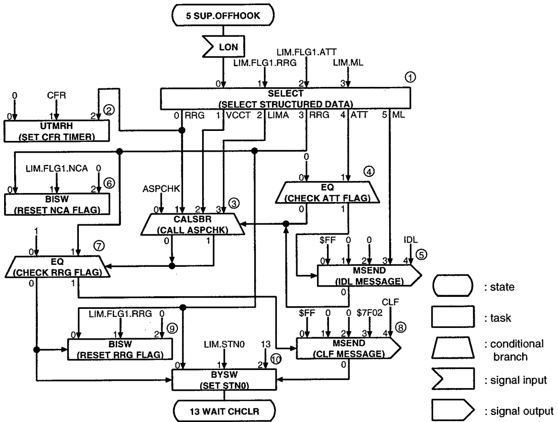
図 2.6 図的データ駆動言語 DDL による徹底した部品化例
