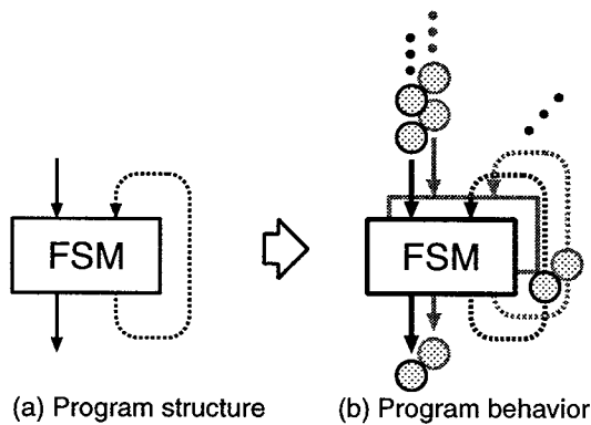
図 3.6 FSM 構造の動的データ駆動型多重実行
