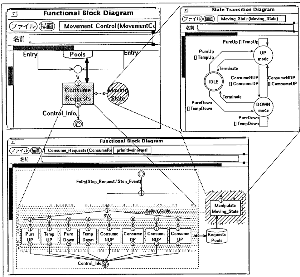
図 5.9 リフト制御問題の仕様記述例
