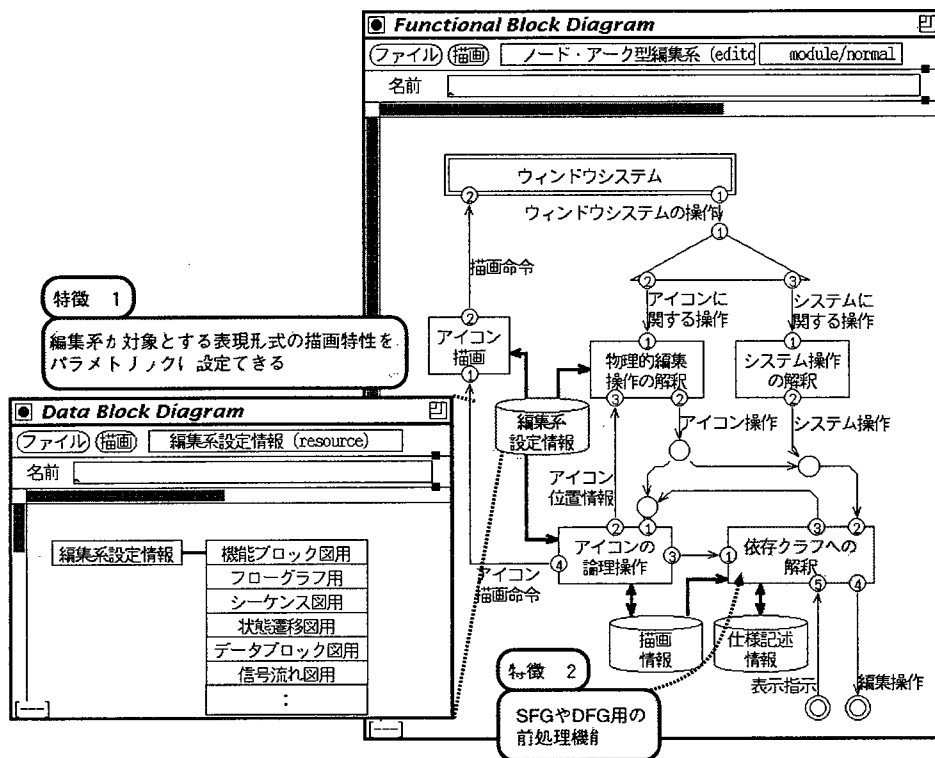
図 5.5 ノード・アーク系図的表現の編集系の構成
