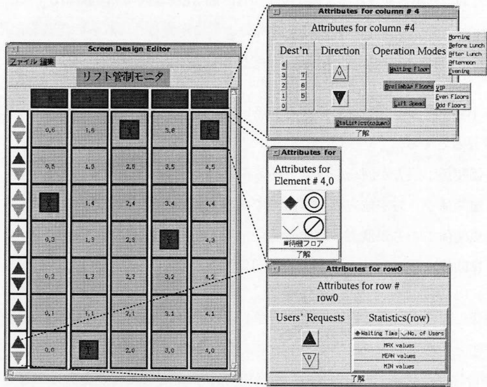
図 3.3 ユーザインタフェースの図的記述例
