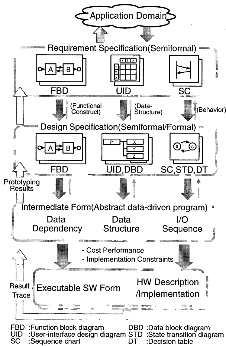
図 3.1 統合的システム記述体系 AESOP の概要
