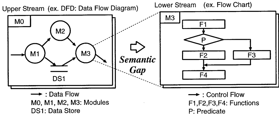
図 2.2 構造化分析・設計の流れ
