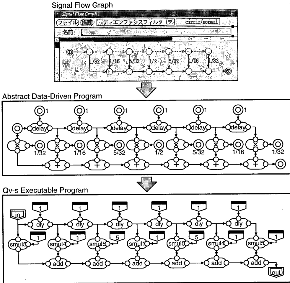
図 3.9 デイエンファシスフィルタの SFG 記述からのデータ駆動型プログラムの生成例
