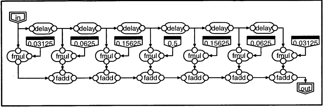
図 4.5 デイエンファシスフィルタの Qv-m プログラム
