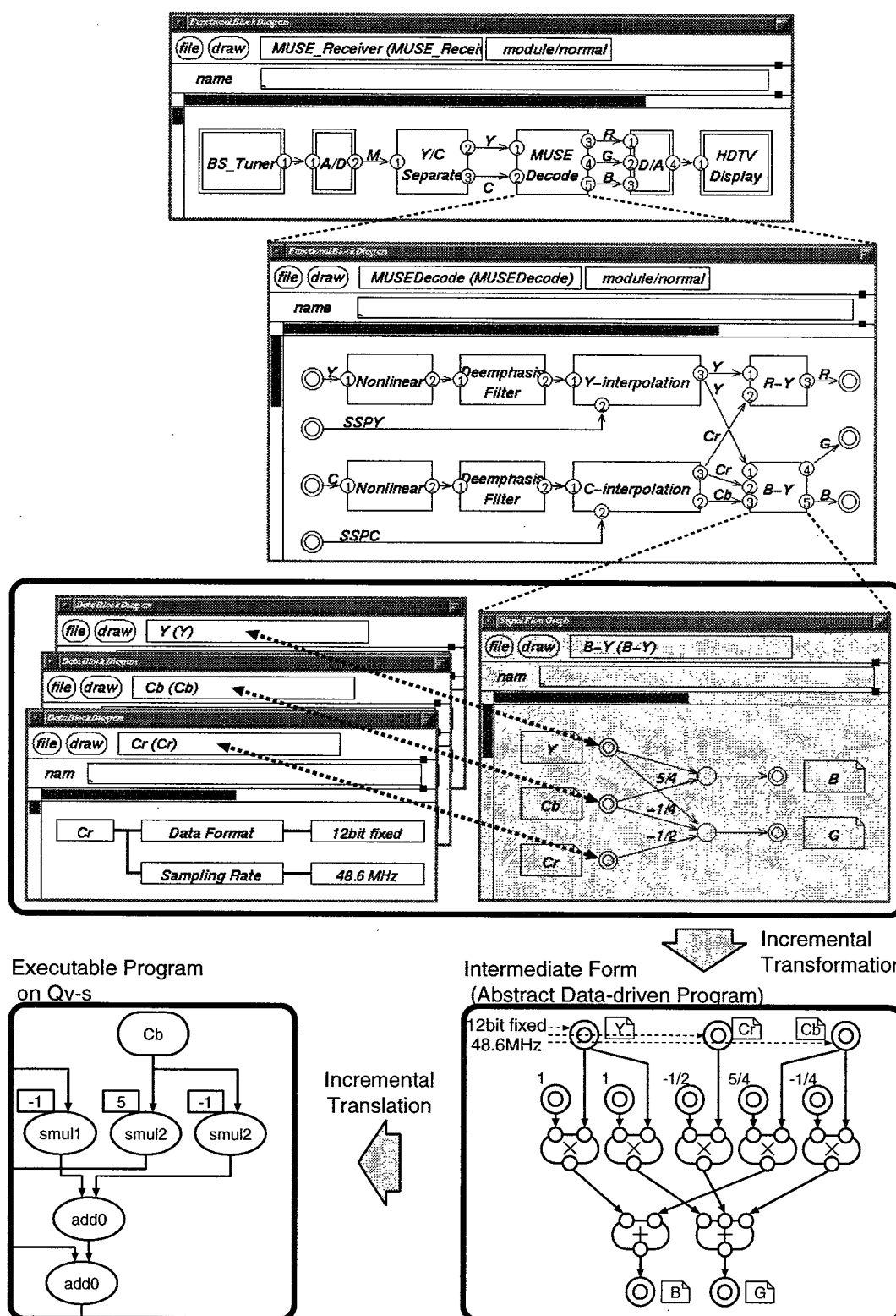
図 5.11 MUSE 信号デコーダの仕様記述例とそのデータ駆動型プログラムの生成例
