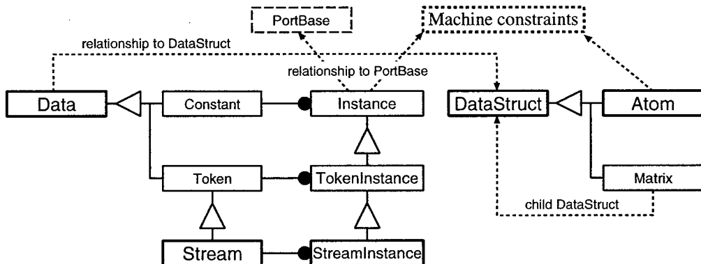
図 5.3 中間形式のデータ構造情報
