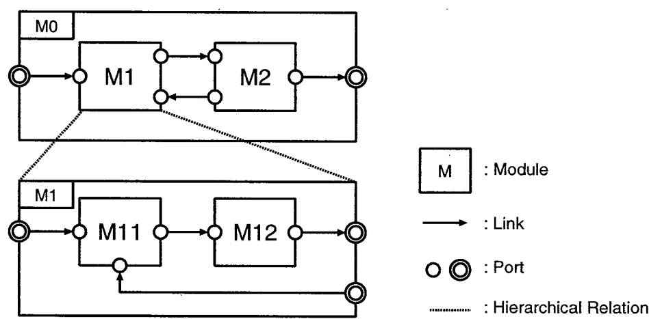
図 3.2 機能ブロック図の構成要素
