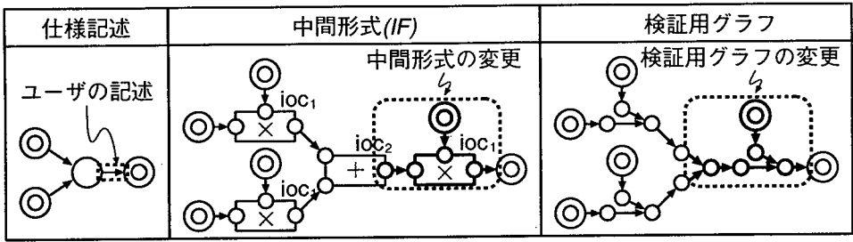
図 4.3 トークンフロー検証用グラフ
