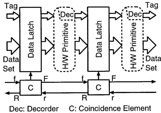
図 2.8 自己タイミング型パイプライン機構
