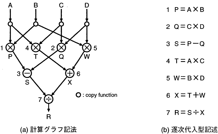
図 2.4 データ駆動型記述と逐次代入型記述
