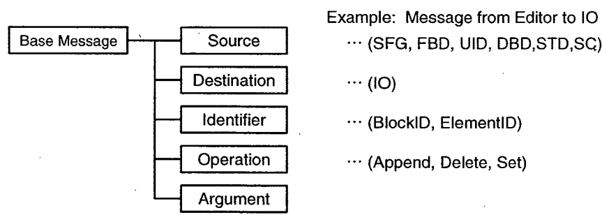
図 5.4 サブシステム間のメッセージ形式
