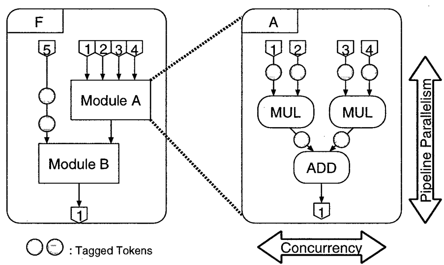
図 4.6 データ駆動型プログラムとその動作
