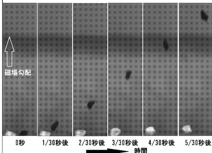
図 3 試料の運動（連続写真） 間隔は 1/30 s 右の黒い試料がグラファイト（磁化率文献値 \chi = -52 \times 10^{-7} \text{ emu/g} ）で、右の白い試料がセルロース（平均幅 1.0mm 文献値 \chi = -5.7 \times 10^{-7} \text{ emu/g} ） 5/30 秒後までに、グラファイトは 12mm、セルロースは 1mm 鉛直上向きに運動した。
