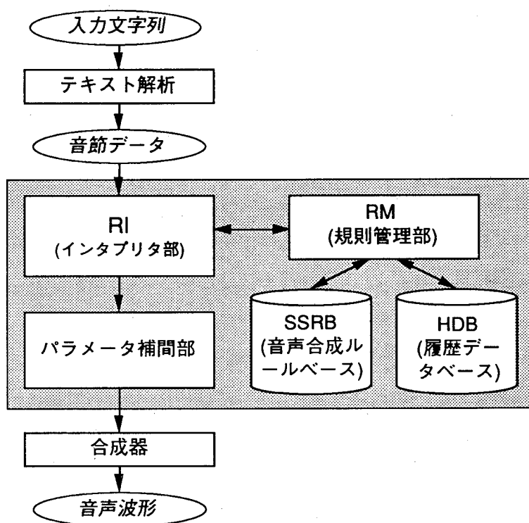
図3.16 SSRI の構成
