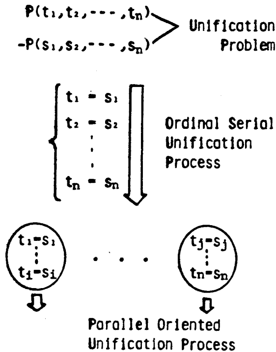
図 5 - 1 単一化計算の逐次処理と並列処理
