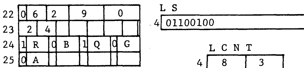
図 4 - 1 2 生成された導出形の内部表現
