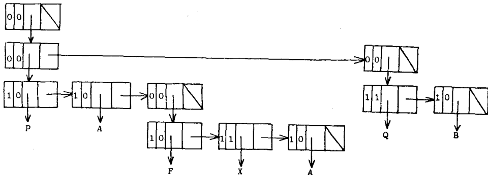
図 3 - 3 入力節の内部構造
