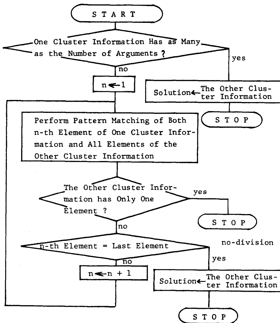
図5-8 クラス演算アルゴリズム
