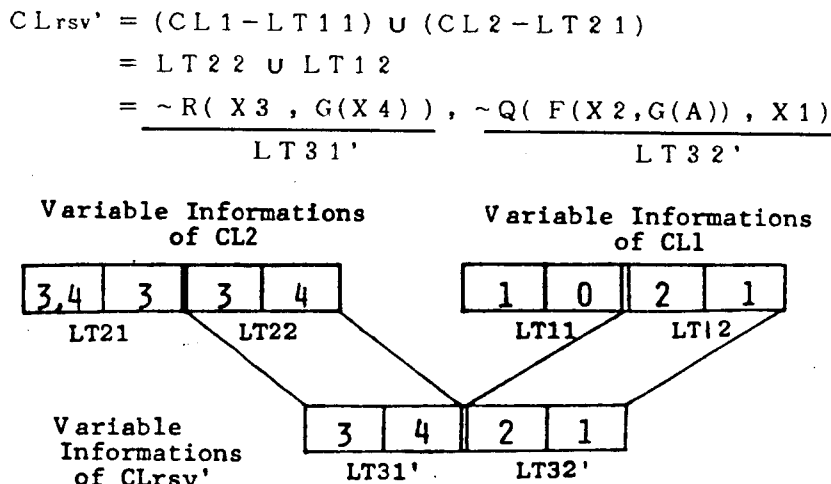
図5-12 フェーズ1の処理
