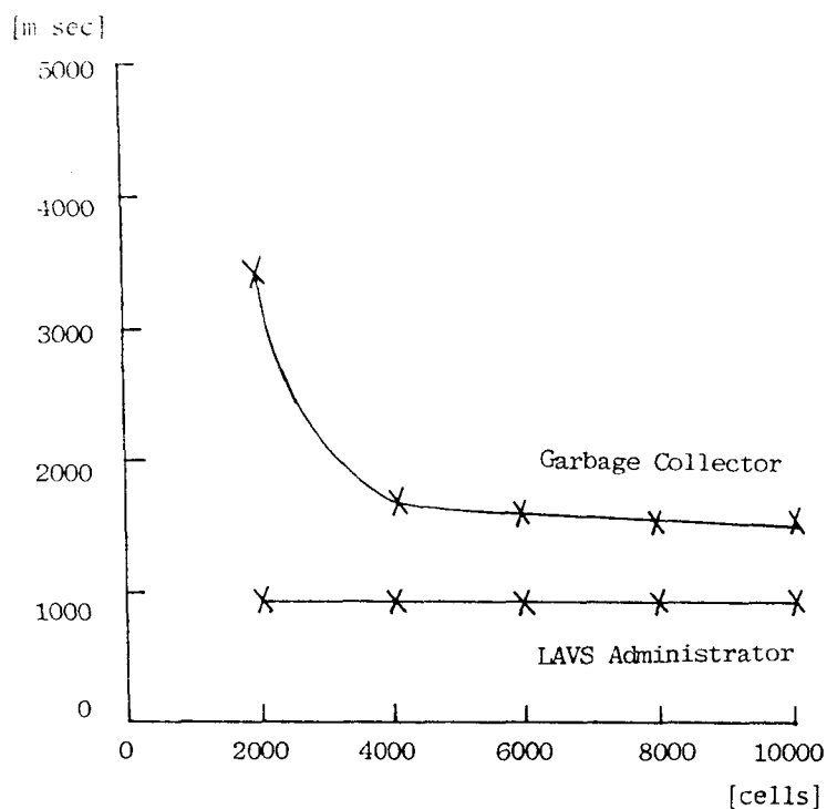
図3-16 Garbage Collector 及び LAVS Administrator を使用した時のTPUを実行する SENRI FORTRAN バージョンの効率比較
