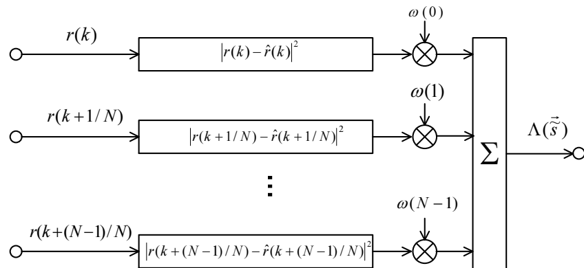
図 2-7 状態数を制限した場合のブランチメトリック演算回路
