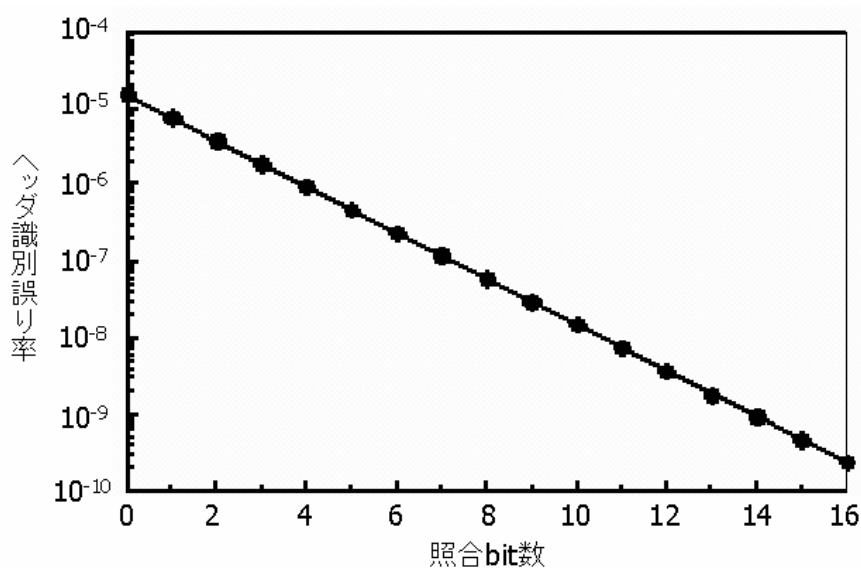
図 3-9 データグラム識別誤り率
