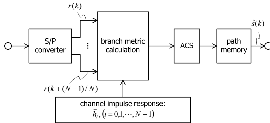
図 2-4 分数間隔サンプルを用いた MLSE 受信器
