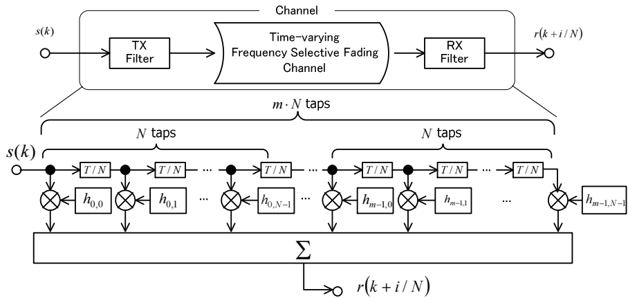
図 2-2 通信路モデル
