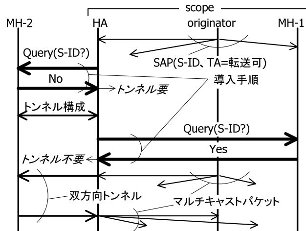
図 3-23 HA によるトンネルの構成手順
