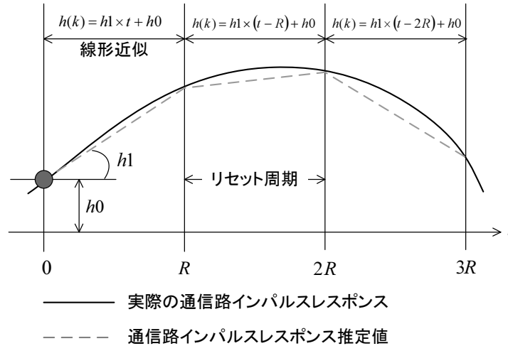
図 C-1 1 次 QT-LMS アルゴリズムによる推定コンセプト
