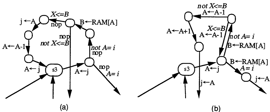
図9 提案する設計法で得られる遷移図と簡約化作業によって得られた遷移図（部分）
