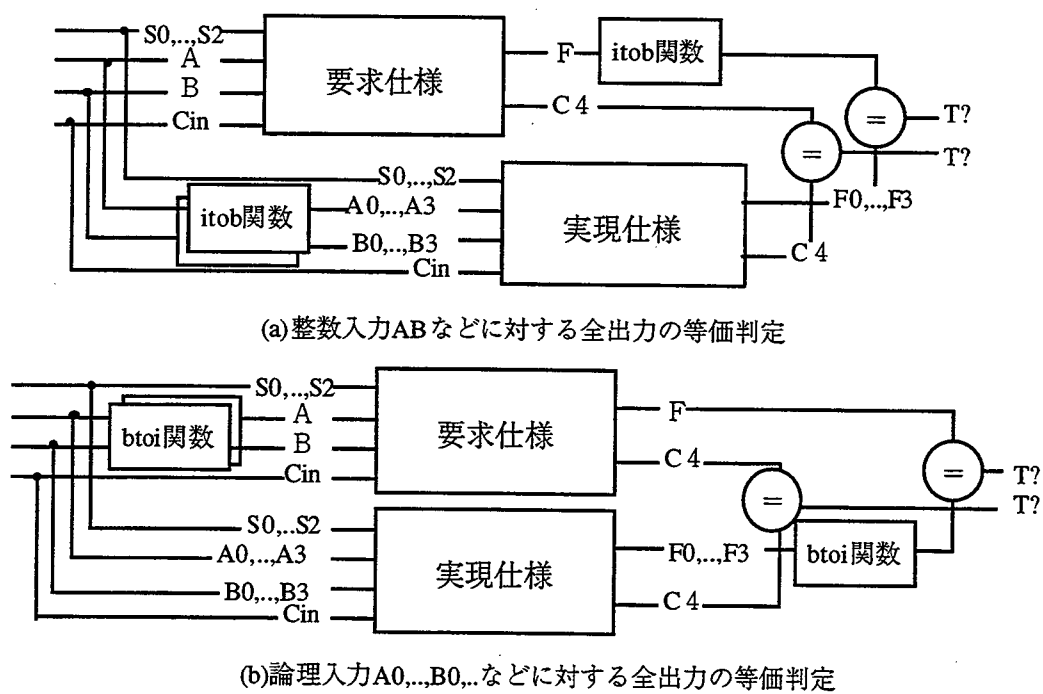
図 1 7 74382の検証の概要
