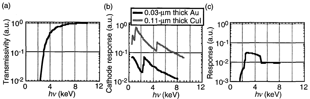
図3.3.18 フィルター／フォトカソードの組み合わせによって観測X線波長域が決まる。(a) BSPを考慮した5 \mu\text{m} 厚Ti金属薄膜フィルターの透過率。(b) 0.03 \mu\text{m} 厚のAuカソードと0.11 \mu\text{m} 厚のCuIカソードのレスポンス。(c) Tiフィルター／Auカソードの組み合わせに対する観測X線波長領域。
