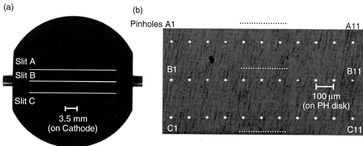
図3.5.3 McMIXS法で使用したカソード・ディスク (a) とピンホール・ディスク (b) の写真。
