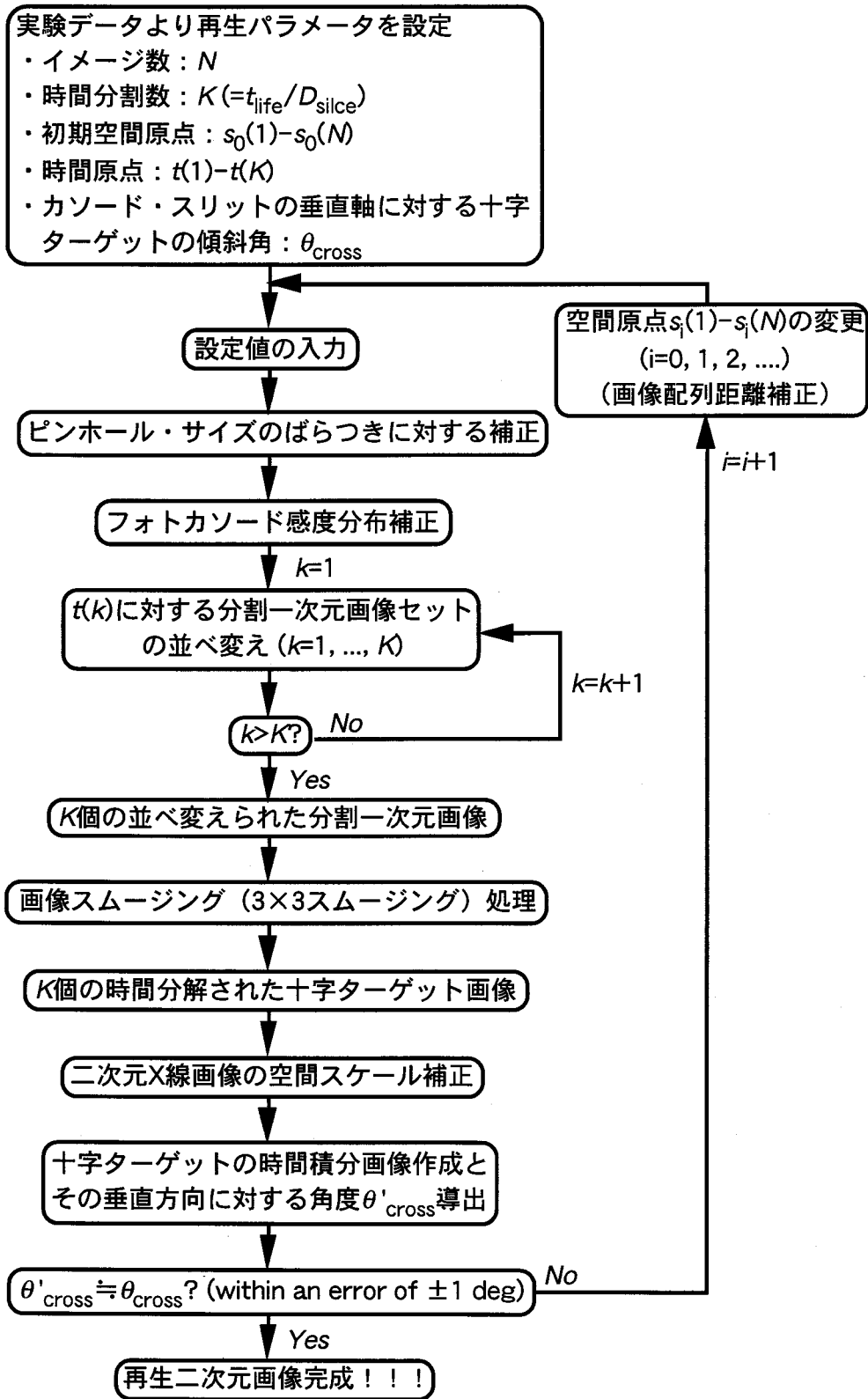
図3.3.12 十字ターゲットに対する二次元X線画像再構成のフロー・チャート。
