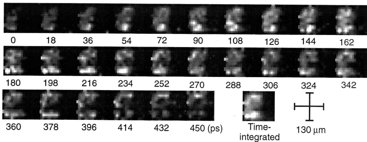
図3.6.5 2D-SIXS法で観測した金コート中実球の時間分解二次元X線画像。フレーム時間間隔は18 psである。
