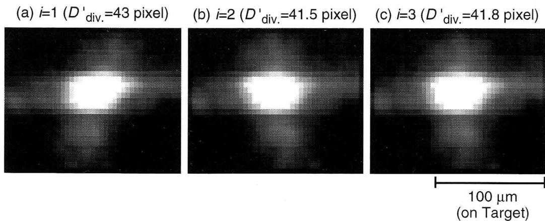
図3.3.16 D'_{div.}=43 (a), 41.5 (b), 41.8 (c) pixelに対する十字ターゲットの時間積分画像。それぞれの \theta'_{cross}=-18.4, 4.25, 0.767 degである。ここで、負符号は垂直軸に対して右に傾いていることを意味している。
