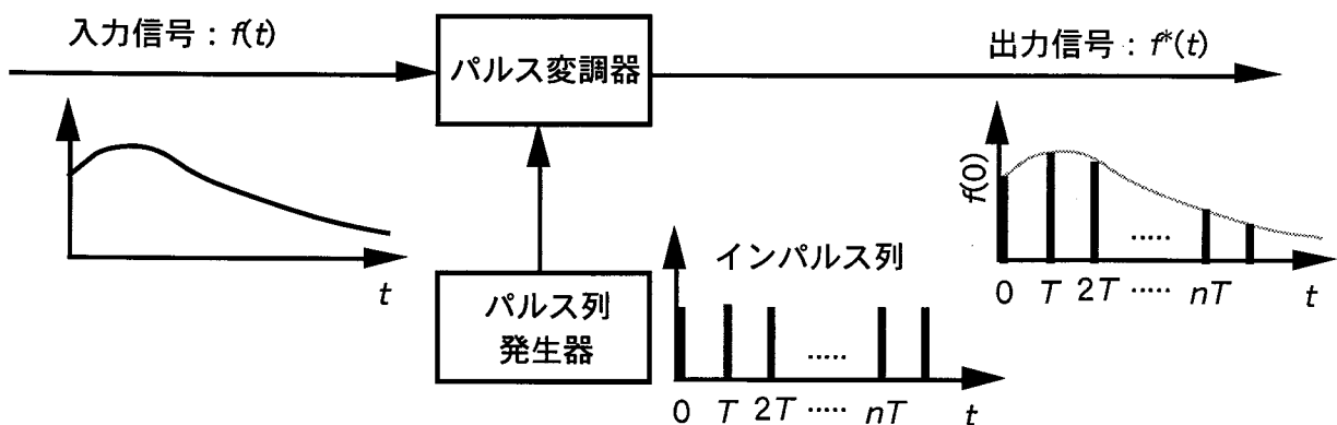
図3.2.3 時系列信号におけるサンプリング。
