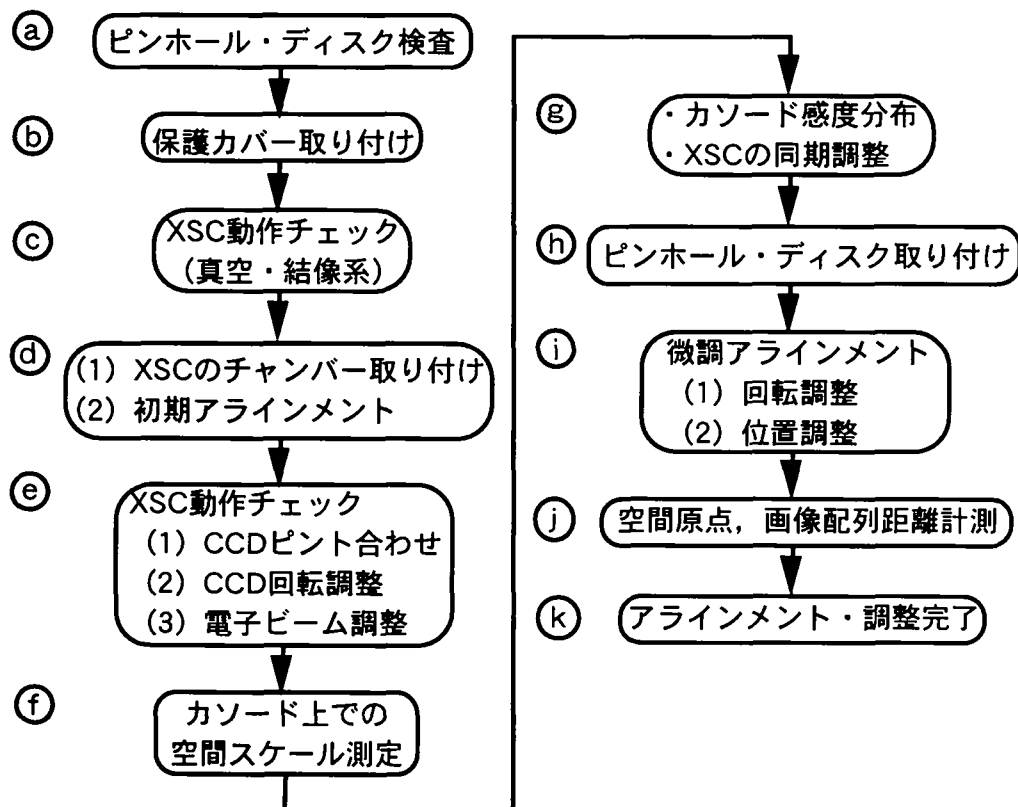
図B.1 MIXS法のアラインメント及び調整手順のフロー・チャート。
