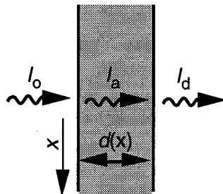
図3.3.7 フォトカソードの断面図。入射X線 (強度 I_0 ) は、フォトカソード内で吸収され光電子となるもの (強度 I_a ) と透過するもの (強度 I_d ) に分類できる。
