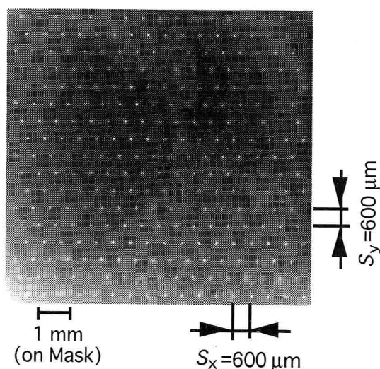
図3.6.2 サンプリング・マスクの光学顕微鏡写真。
