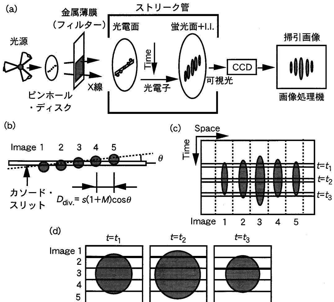
図3.3.1 MIXS法の原理図。(a) MIXS法のシステム全体の概要図。(b) ストリーク・カメラのカソード・スリット上に結像された光源像の画像列。(c) ストリーク管によって時間掃引された分割一次元画像。(d) 任意の時刻 t=t_1, t_2, t_3 の画像再構成された二次元画像。
