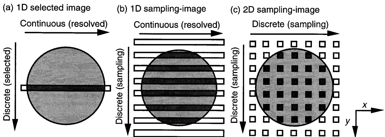
図3.2.2 X線ストリーク・カメラの光電面上での画像サンプリング．(a) 光源のある場所の一次元空間分解計測に限られる．(b) y 方向の一次元画像サンプリング，(c) x, y 方向の二次元画像サンプリングによって光源の二次元空間情報を得ることができる．
