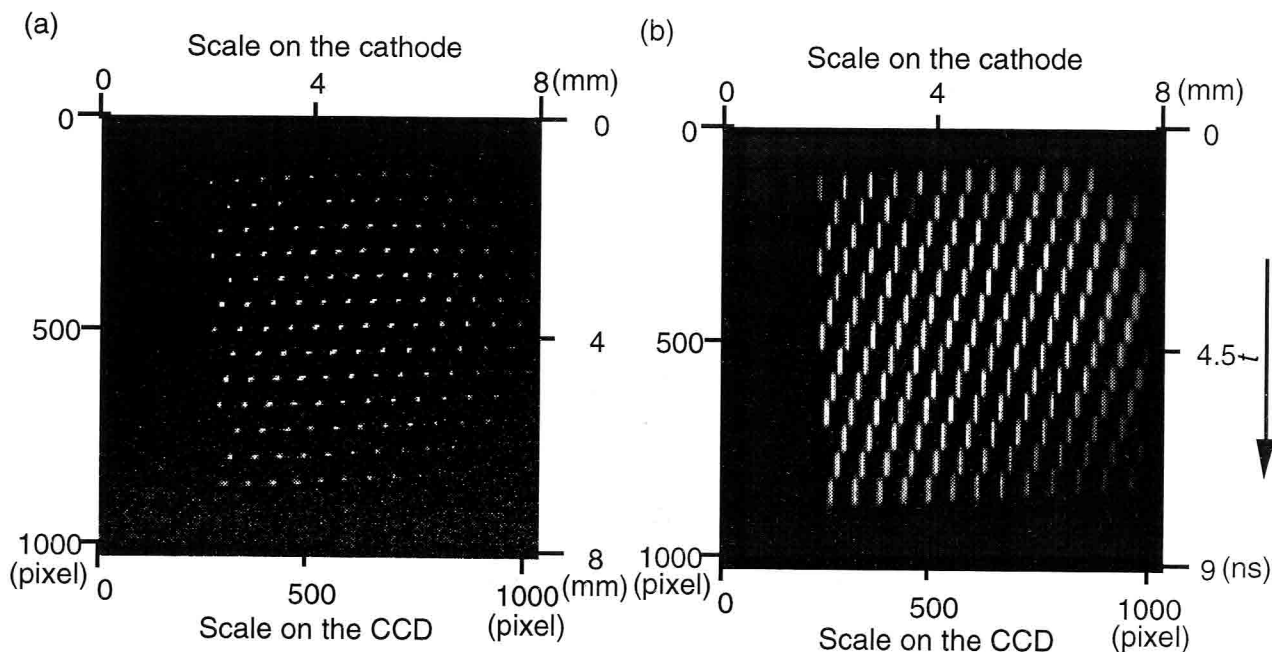
図3.6.3 2D-SIXS法によって観測されたサンプリング点全体の静止画像 (a) と時間掃引画像 (b)。
