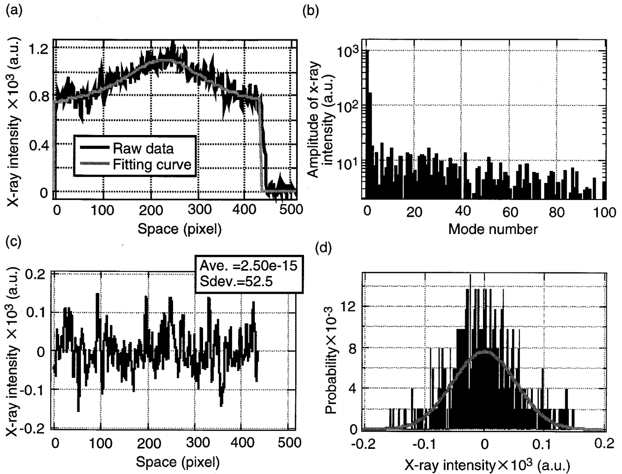
図3.3.6 フォトカソード感度分布補正に関する解析. (a) 厚さ 0.03 \mu\text{m} のAuカソード感度分布. 横軸はCCDカメラ上における水平方向の空間軸を示している. (b) X線発光強度の空間プロファイル (範囲 x=1-440 pixel) に関するモード展開. モード数は考慮した空間範囲内の空間周波数に相当する. モード0は直流成分, モード n は考慮した範囲内で n 個の凸凹があることを意味する. (c) モード2以上の発光強度の空間プロファイル. 平均値は 2.50e-15 , 標準偏差は52.5であった. (d) 同図(c)の確率度数分布. 実線はモード2以上の発光強度の平均値, 標準偏差で記述した正規分布曲線である.
