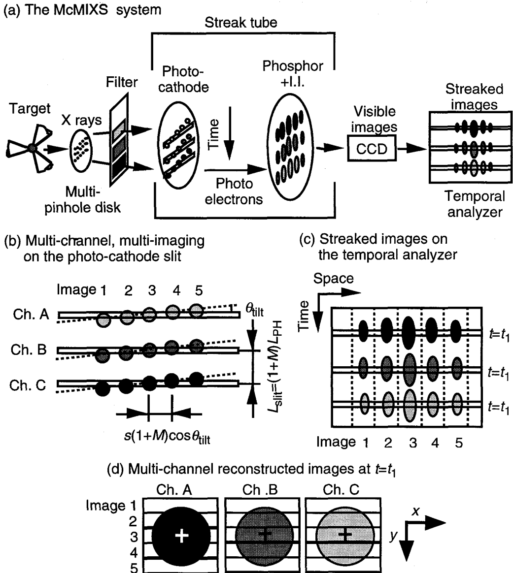
図3.5.1 McMIXS法の原理図. (a) McMIXSシステム全体の概略図. (b) 三つのカソード・スリットとピンホール列とフィルターの組み合わせにより、光電面上に3チャンネルの分割一次元画像のセットを結像する. (c) 3チャンネルの分割一次元画像セットの時間掃引画像. (d) t=t_1 での再構成された3チャンネルの二次元X線二次元画像.
