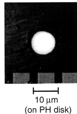
図3.3.2 Ta基板（厚さ 25\ \mu\text{m} ）にマイクロ放電加工により製作された直径約 10\ \mu\text{m} のピンホール．
