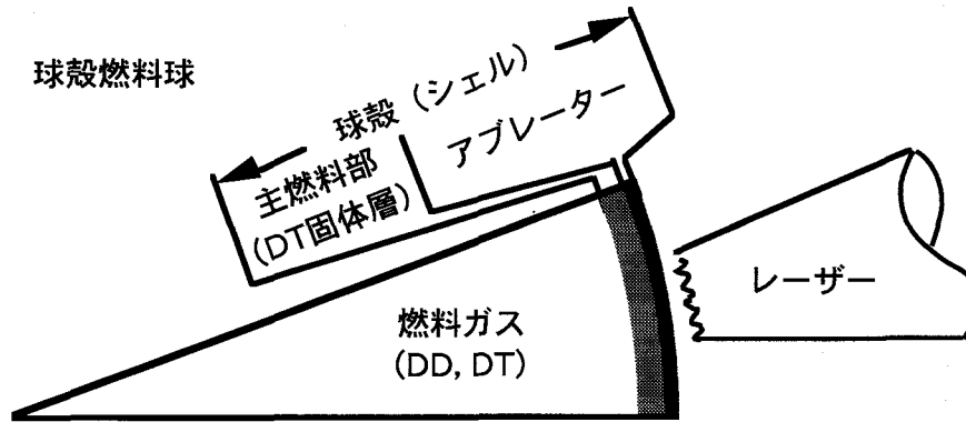
図1.2.1 高利得用レーザー核融合ターゲット。核融合点火源となる燃料ガス部の周りを主燃料部であるDT固体層が取り巻き、その外側をプラスチックのアブレター層が覆っている。
