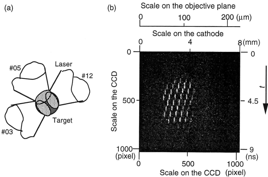
図3.6.4 計測器から見たレーザー照射系 (a) と金コート中実球のX線発光形状を二次元画像サンプリングした時間掃引画像 (b)。
