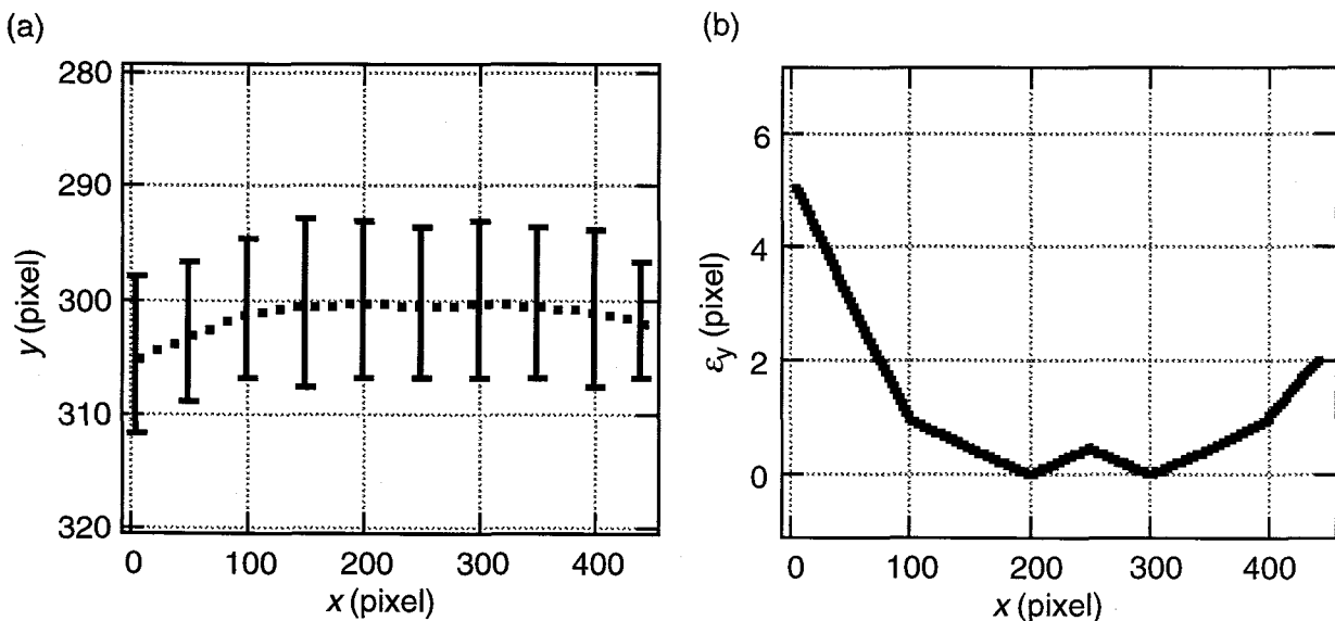
図3.3.10 掃引画像モードでの電子結像の画像歪みに対する評価。(a)時間掃引されたカソード・スリットは上に湾曲した弓形の構造を持つ。(b)画面中央( x=200-250 pixel)に対する画像歪み \varepsilon_y (pixel)。
