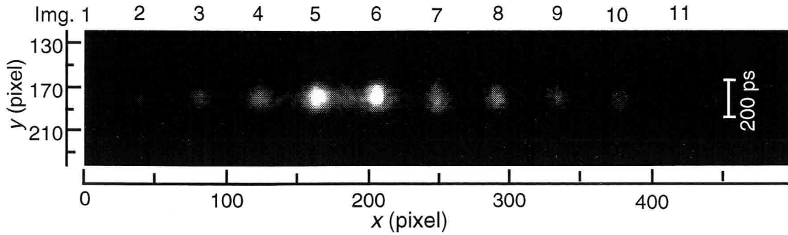
図3.3.15 MIXS法によって得られた十字ターゲットの時間掃引画像。イメージ1は画面端にかかっており，イメージ11はカソード・スリットの有効幅外にある。
