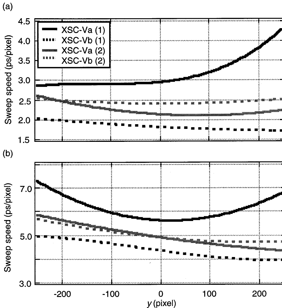
図3.3.11 第三、四章で使用したXSC-Va, Vbの2 ns (a), 5 ns (b) 掃引画像モードに対する掃引速度の時間軸に対する依存性. (1), (2) は掃引速度較正を行った時期が異なることを意味している. y 軸の0は画像処理機上の画面中央 y=250 pixel付近に相当する. 負符号は画像処理機画面上で上を意味している. 例えば, カソード・スリットの y 軸方向の位置が画面中央250 pixelにあるとすると, 0, 100, 200, 300, 400, 500 pixelでの時間掃引歪みは, それぞれ図中での-250, -150, -50, 50, 150, 250 pixelに対する数値に対応する.
