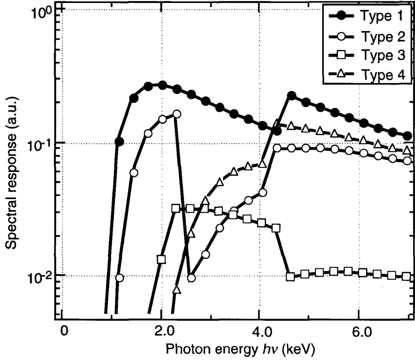
図3.3.19 MIXS, 1D+MIXS, McMIXS, 2D-SIXS法で使用するフィルター／カソードの組み合わせに対する観測X線スペクトル。Type 1はBSP/CuI, Type 2はBSP+35 μm厚CHCl/CuI, Type 3はBSP+5 μm厚Ti/Au, Type 4はBSP+500 μm厚Be/CuIの組み合わせである。ただし, 1D+MIXS法については3.4節と4章の設定が異なる。
