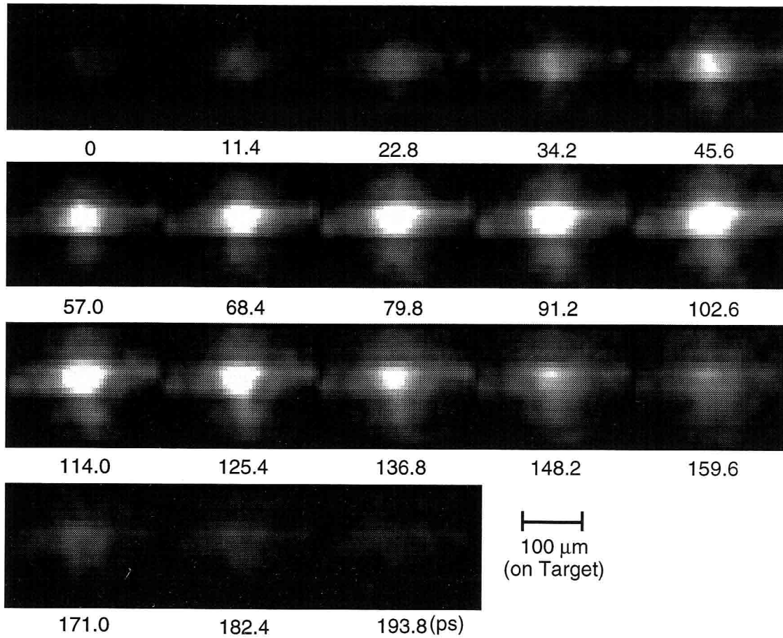
図3.3.17 D_{div.}=41.8 pixelに対する十字ターゲットの時間分解二次元X線画像. フレーム時間間隔は11.4 psである.
