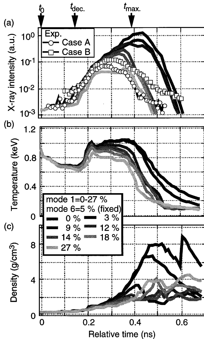
図4.3.5 NU_1=0-27\% , NU_6=0-20\% に対するX線発光強度 (a), 温度 (b), 密度 (c) の時間発展を示す。各時間プロファイルは図4.3.3と同じ手法で表示している。
