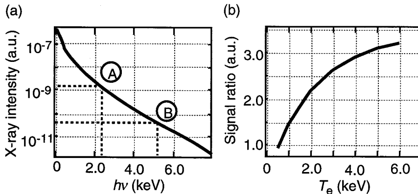
図3.5.2 電子温度導出原理。(a) 電子温度 kT_e=1.5 keVに対する束縛-自由、自由-自由遷移によるX線スペクトル。(b) McMIXS法での電子温度-信号強度比 (Ch. C/Ch. B) 曲線。
