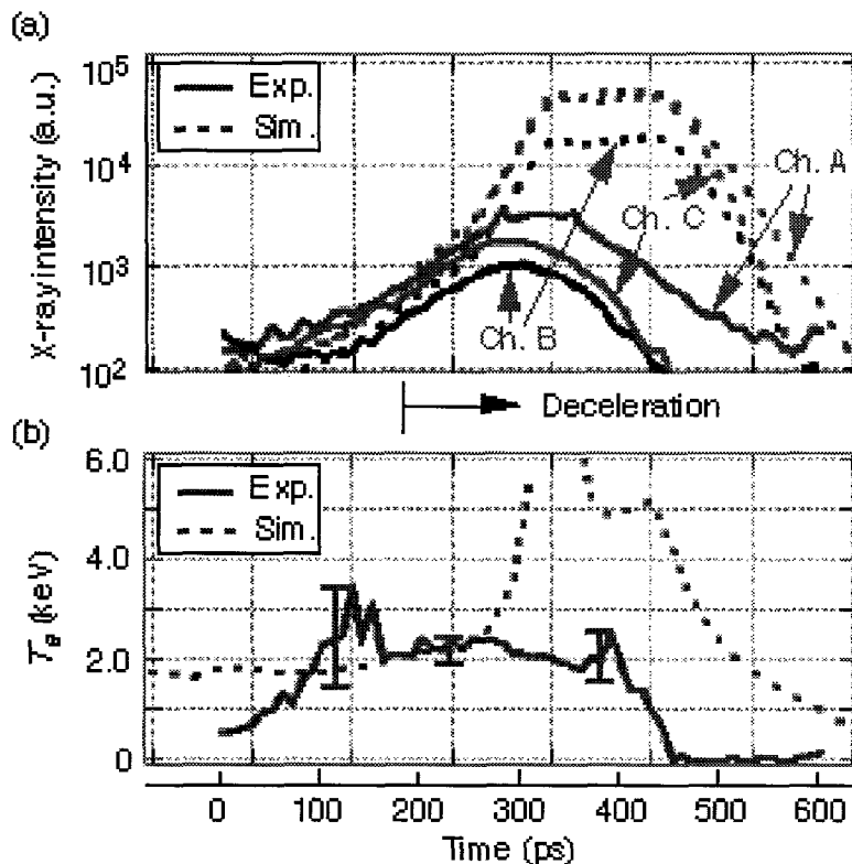
図3.5.6 実験結果と一次元シミュレーション結果との時間プロフィール比較。時刻は図3.5.4の一次元シミュレーションの時刻に対応している。(a) コア中心での各チャンネルのX線発光強度の比較。縦軸のスケールは発光初期 ( t<200 ps) で実験とシミュレーション結果を一致させた。(b) コア中心部の電子温度の比較。図中のエラー・バーは雑音レベルの信号による誤差を示す。
