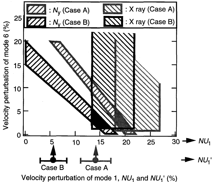
図4.3.9 NU_1, NU_6 のパラメータ領域におけるX線及び中性子の実験結果と二次元シミュレーション結果との比較のまとめ。XPCの爆縮コア変位から求めたCase A, Bに対するモード1の速度非一様性 NU_1' も示す。
