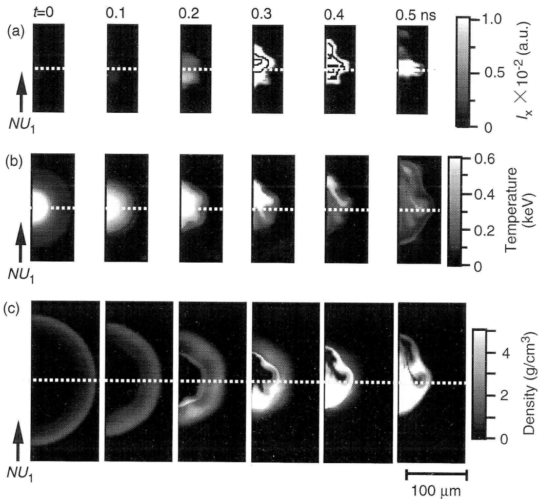
図4.3.4 二次元シミュレーションによる NU_1=18\% 、 NU_6=5\% に対する二次元X線画像 (a)、温度分布 (b) 及び密度分布 (c)。二次元X線画像の等高線は発光強度0.04 a.u.の間隔で表示している。
