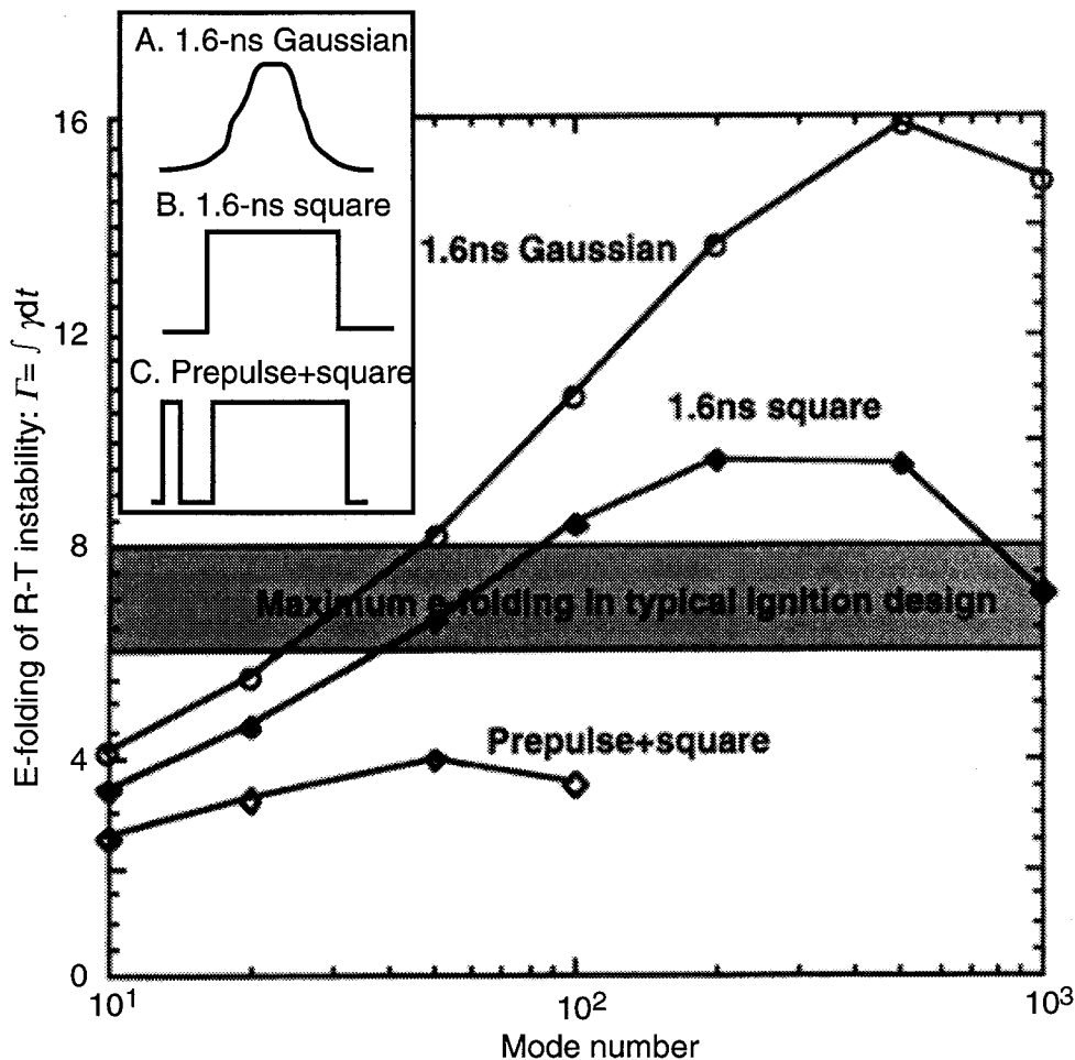
図2.3.3 1.6 nsガウス型, 1.6 ns矩形波, プレパルス+矩形波に対するR-T不安定性のe-folding: \Gamma = \int \gamma dt . 一般的な点火ターゲットは \Gamma = 6-8 で設計される。
