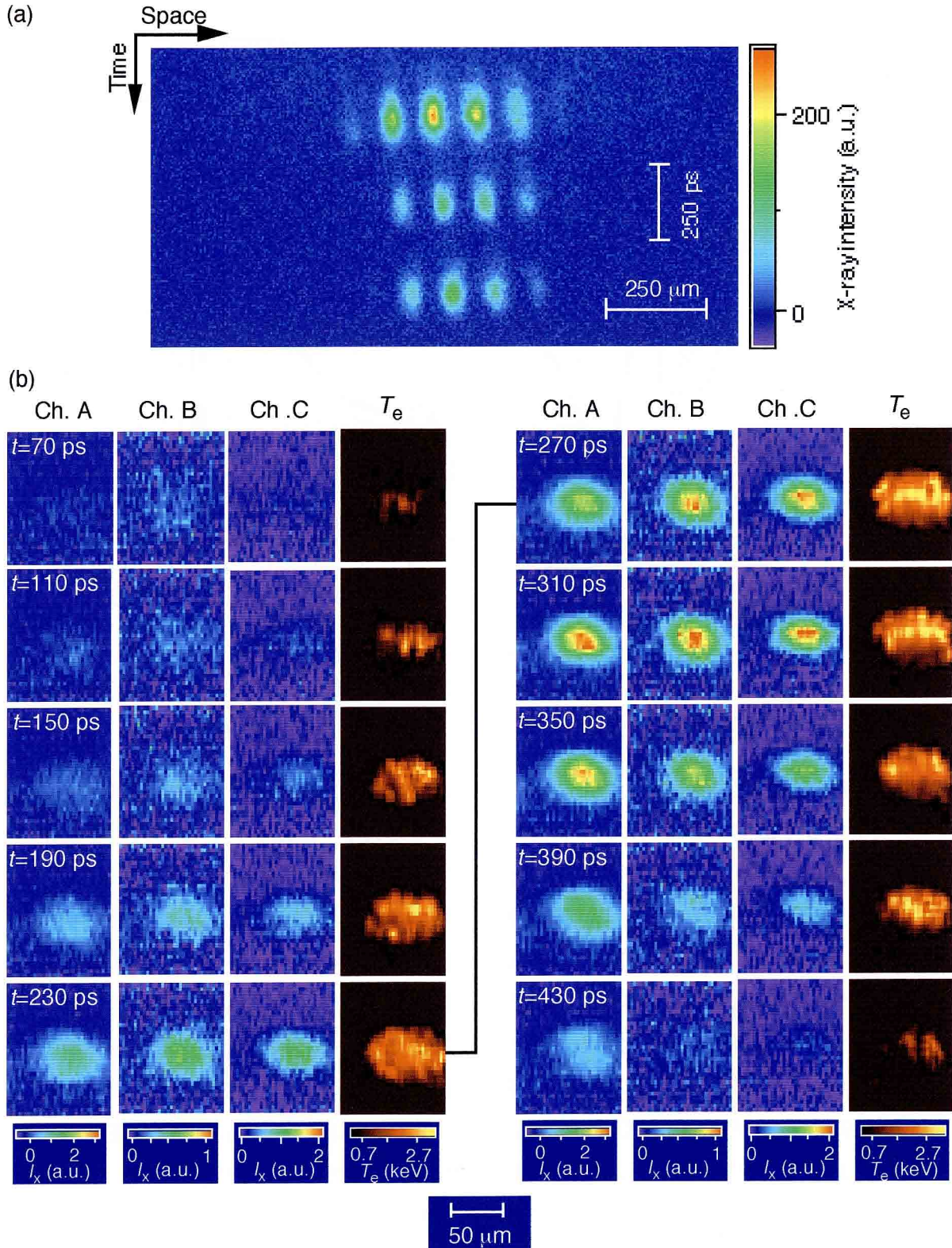
図3.5.5 McMIXS法による爆縮コア・プラズマ・ダイナミクス診断. (a)各チャンネルの分割一次元画像セットの時間掃引画像. (b)再構成したCh. A, B, Cの二次元X線画像と T_e の二次元空間分布. それぞれ異なるカラー・バーで色表示した. また, 得られる二次元画像はフレーム時間間隔10 psであるが, 便宜上40 psおきに表示した.
