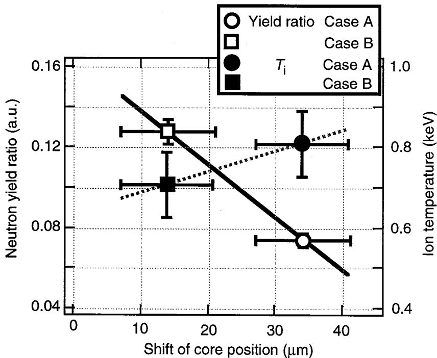
図4.2.9 中性子イールド及びイオン温度の爆縮コア変位に対する依存性。
