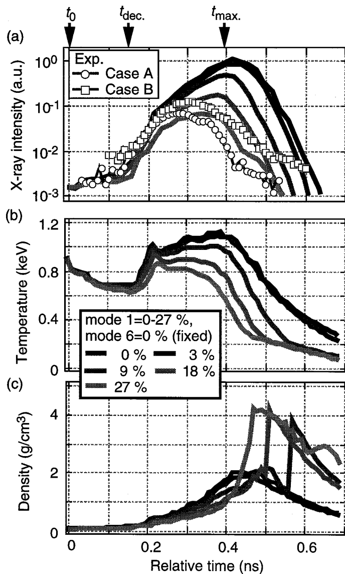
図4.3.3 NU_1=0-27\% , NU_6=0 に対するガス燃料内の垂直軸上にある最大温度位置でのX線発光強度 (a), 温度 (b), 密度 (c) の時間発展を示す。図4.2.8 (c) に示した爆縮コア中心での時間発展の実験結果を同図 (a) に示す。
