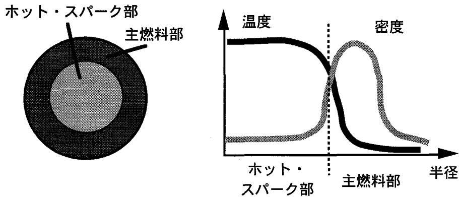
図1.2.2 高利得実現には爆縮最終段階でホット・スパーク構造を安定に形成する必要がある。
