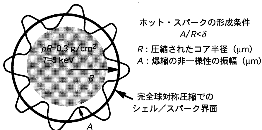
図2.3.1 ホット・スパーク形成条件。スパーク／主燃料間に流体混合があると点火に寄与する領域が小さくなる。擾乱を受けていない領域が点火条件を満たさなければならないと考える。
