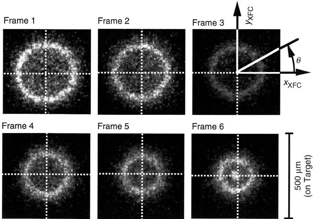
図4.2.3 XFCによって観測されたCase Aの時間分解，二次元空間分解データ．フレーム時間間隔は100 psである． \theta は円周方向の角度を示している．また，XFCの観測平面の座標を (x_{XFC}, y_{XFC}) によって示す．白い点線の交点がチャンバー中心を示している．
