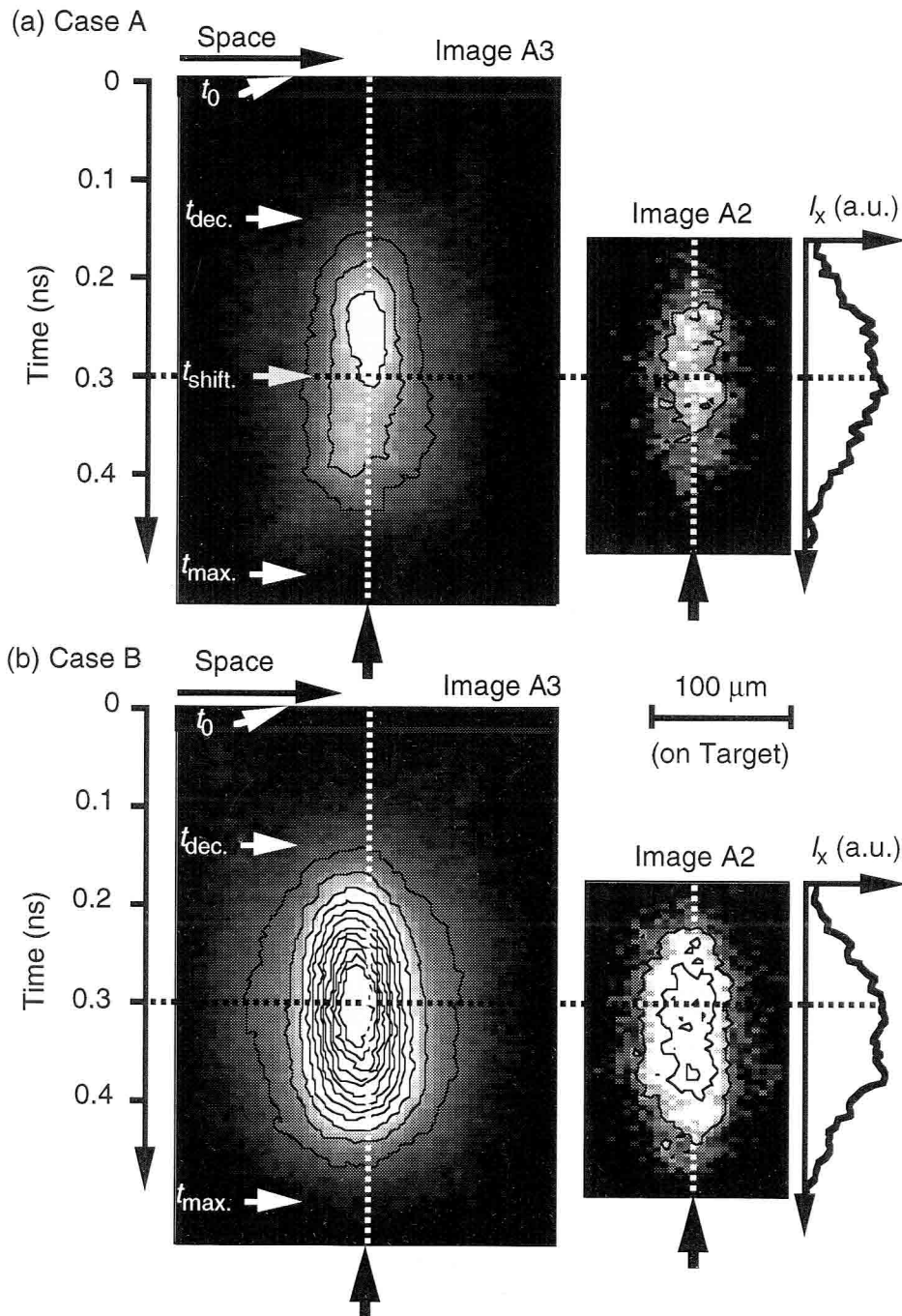
図4.2.7 減速相におけるチャンネルA2(コア), チャンネルA3(コア周辺のシェル) の時間掃引画像. イメージA2の空間積分した時間プロファイルを示す. 相対時間は図4.2.4に示した一次元シミュレーションでの絶対時間に対応している. また, t_0 , t_{\text{dec}} , t_{\text{max}} も図4.2.4で定義したものである. 白い点線はチャンバ中心を示している. イメージA2, A3の等高線はそれぞれX線強度において60, 200カウントの間隔で表示している. また, この観測平面に投影したXPCの爆縮コア位置を太い矢印によって示している.
