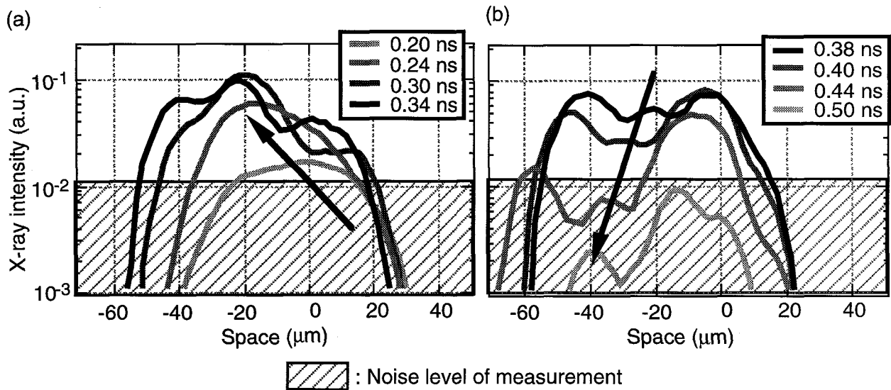
図4.3.6 NU_1=18\% , NU_6=5\% に対する図4.3.4 (a) の垂直軸上のX線発光強度における発光初期 (a), 後期 (b) の空間プロファイル。図中の矢印はプロファイルの中心位置が時間とともに負の方向（二次元コード平面の下から上）へ移動する様子を表している。
