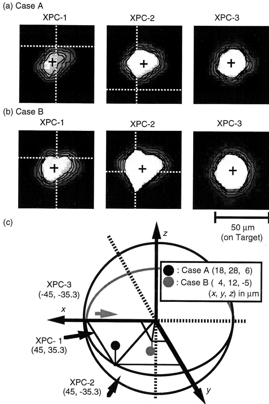
図4.2.2 Case A (a), Case B (b) のXPC-1, 2, 3で観測したコアの時間積分二次元X線画像。コア中央部の画像は飽和している。白い点線の交点がチャンバー中心を、黒い十字の交点がコア中心を示している。XPC-3はチャンバー中心位置計測に失敗したため、チャンバー中心位置を画像内に示していない。(c) (x, y, z) 座標によって表示した三次元的な爆縮コアの中心位置。
