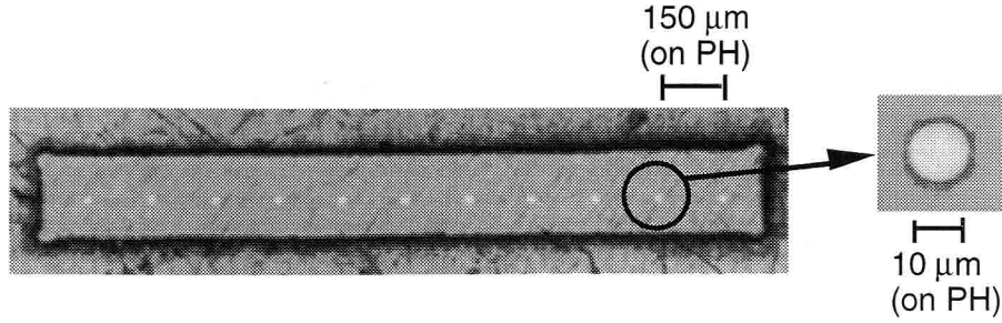
図3.3.14 マルチピンホール・ディスクの光学顕微鏡写真。枠はピンホール・ディスク（Taディスク：径7.5 mm，厚さ25 μm）の上に貼り付けられたピンホール・ディスクと同じ材質の保護カバーの計測用窓である。
