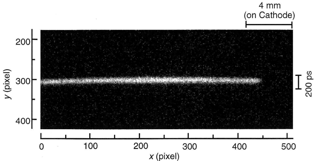
図3.3.5 厚さ0.03 \mu\text{m} のAuカソード・スリットの感度分布．カソード上の空間スケールを示した．
