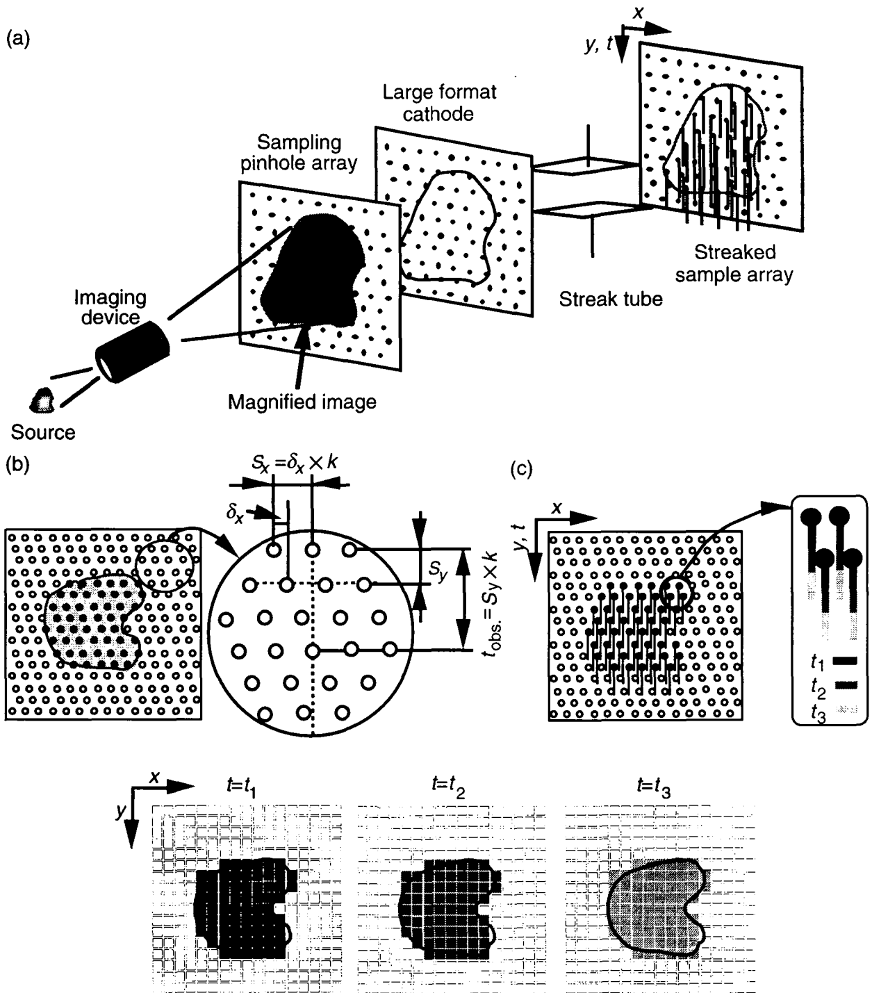
図3.6.1 2D-SIXS法の原理図。(a) 2D-SIXSシステム全体の概略図。(b) 高倍率で光電面上に結像された光源像をサンプリング・マスクによって二次元画像サンプリングを行う。(c) 各サンプリング画像をストリーク管によって時間掃引する。(d) 各サンプリング点における時間掃引画像から、任意の時刻での元の光源の二次元画像を再構成する。
