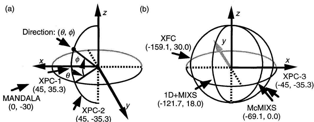
図4.2.1 ある方向から見た計測器配置図 (a) と反対側から見た配置図 (b)．各計測器の観測方向を (\theta(\text{deg}), \phi(\text{deg})) 座標で示す．
