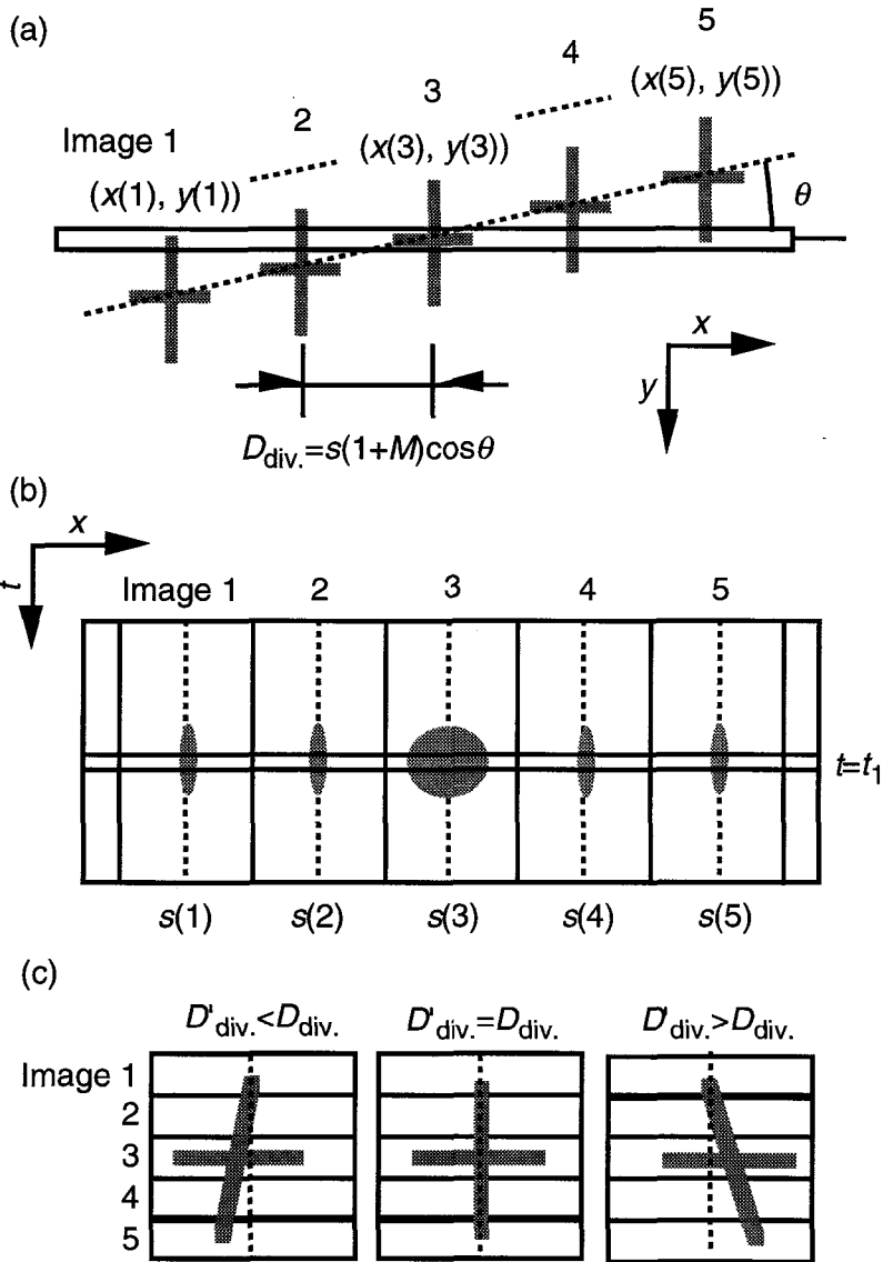
図3.3.3 十字ターゲットを用いた水平方向の画像配列距離に対する補正. (a) 光電面上に結像された十字ターゲット像. それぞれの十字ターゲットの交点を (x, y) 座標で表示した. (b) 同図 (a) の時間掃引像. 各画像1-5の空間原点を s(1) - s(5) で示した. (c) 三通りの画像配列距離による時刻 t=t_1 での再構成二次元画像.
