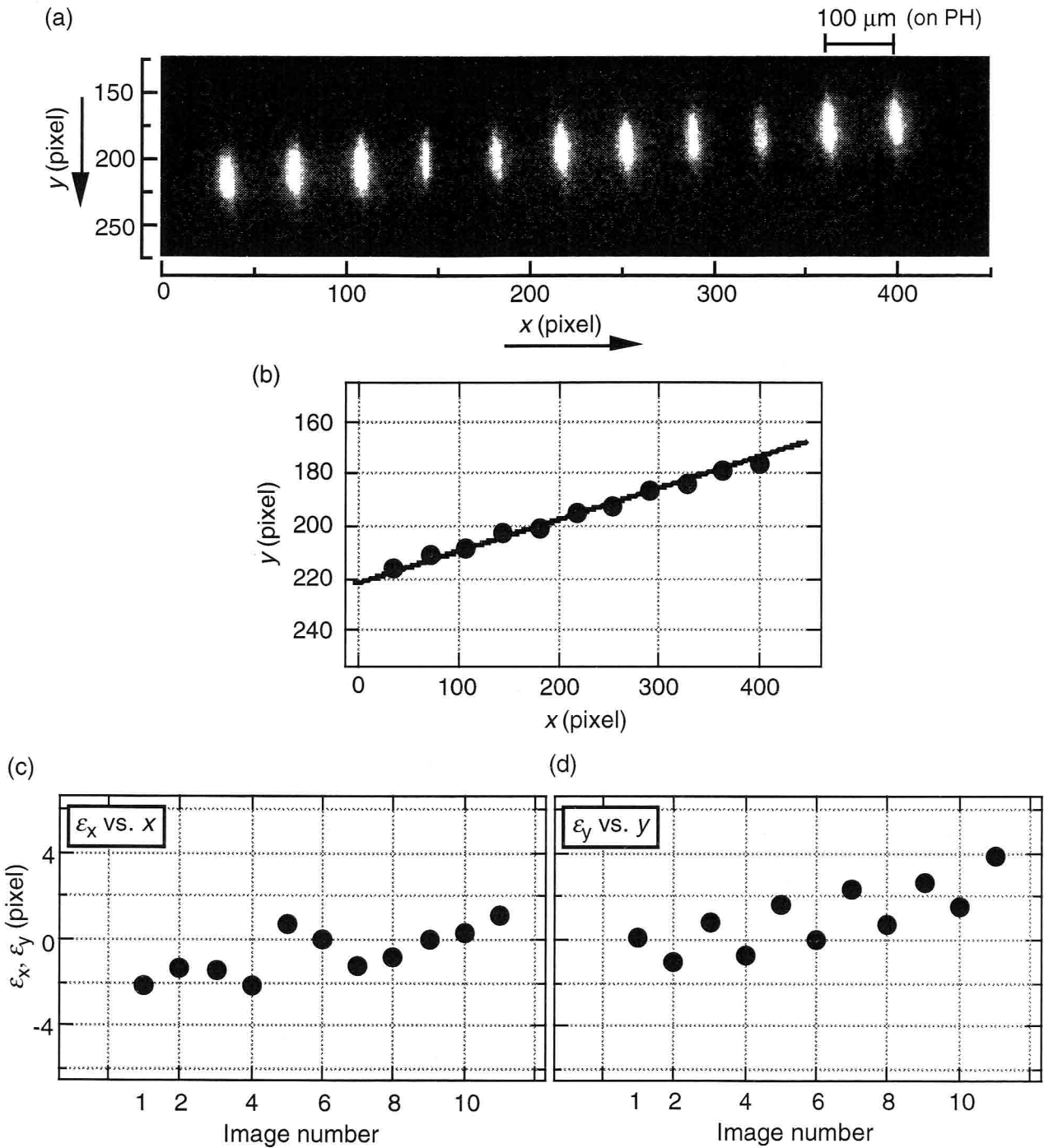
図3.3.9 Auコートしたカーボン・ファイバーを用いた静止画像モードでの電子結像画像歪み評価。(a) Auファイバーの静止画像。図中の空間スケールはピンホール・ディスク上のものである。(b) 各ファイバー画像に対する空間プロファイルの中心位置とイメージ6を基準とした画像歪みがない場合の画像配列直線。(c),(d)に各ファイバー画像に対する x, y 方向の画像歪み \epsilon_x, \epsilon_y を示す。
