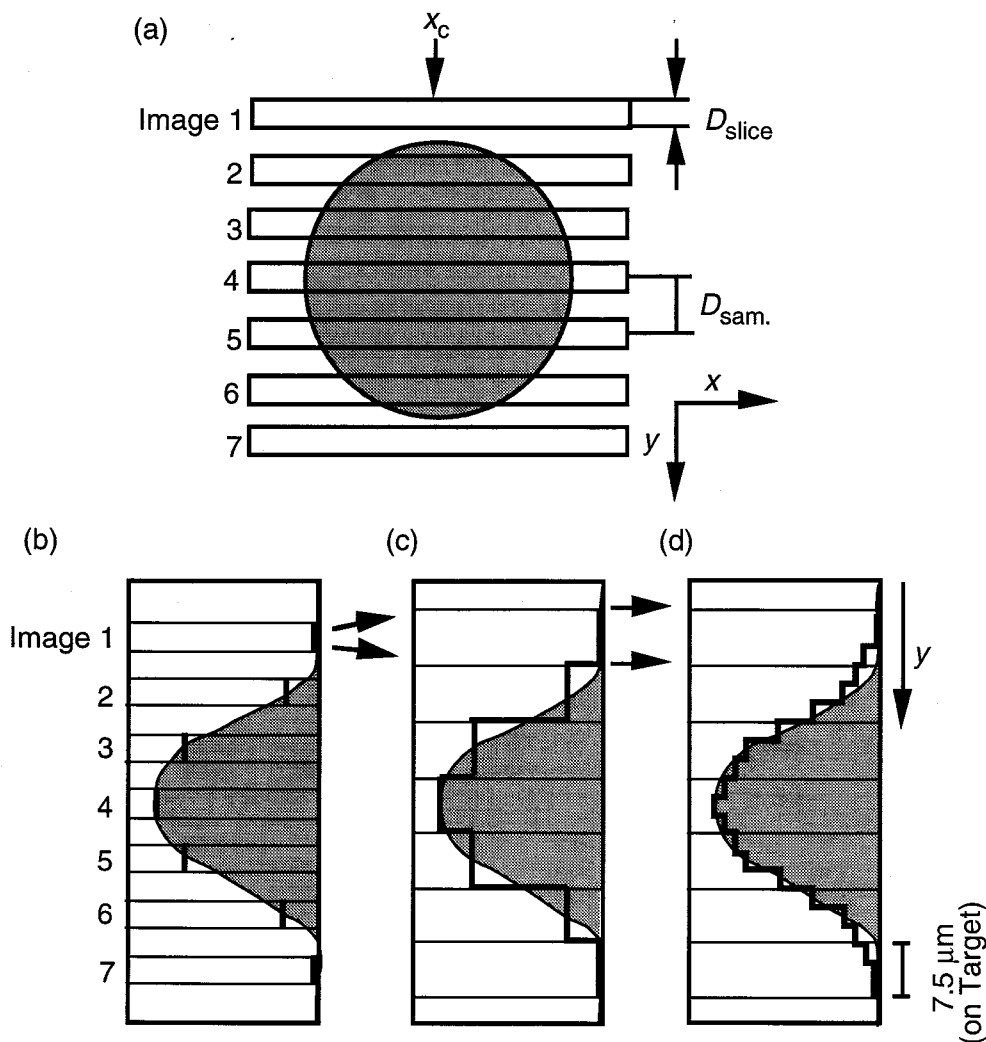
図3.3.4 光源の空間プロファイルにガウス型を仮定した画像スムージング（ 3 \times 3 スムージング）処理の一例。(a) MIXS法によりスライス幅 D_{\text{slice}} 、画像サンプリング間隔 D_{\text{sam.}} で画像サンプリングされた光源像。(b) x 座標 x_c における y 方向の光源の空間プロファイル。サンプリング値を濃い縦線で示す。(c) 計測されていない領域は周辺のサンプリング値で補われる。(d) 画像スムージング処理を施すことにより、光源の空間分布に近づく。
