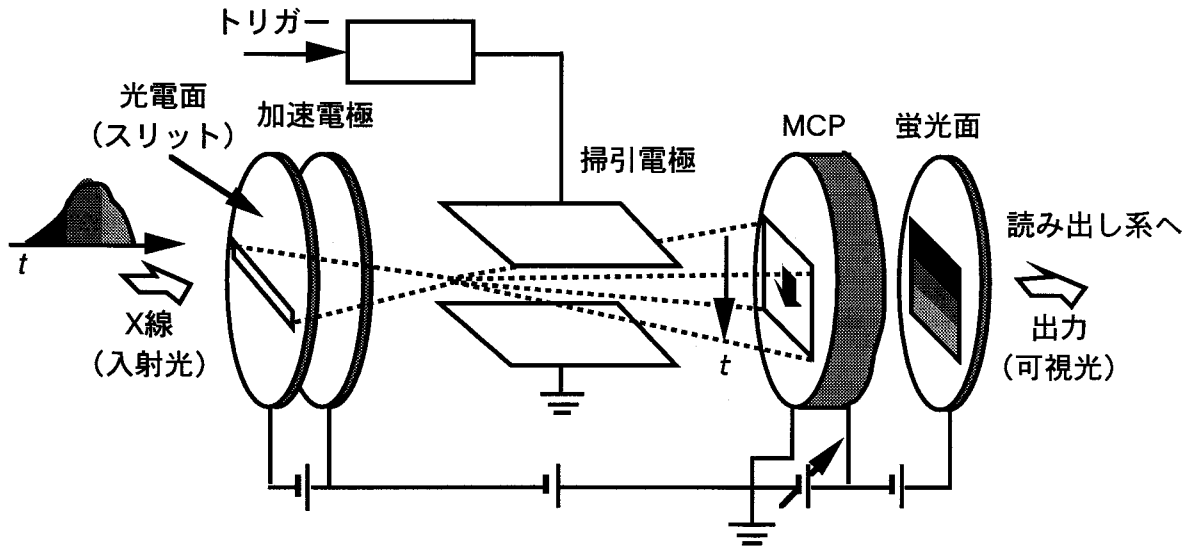
図3.2.1 X線ストリーク・カメラの動作原理図。
