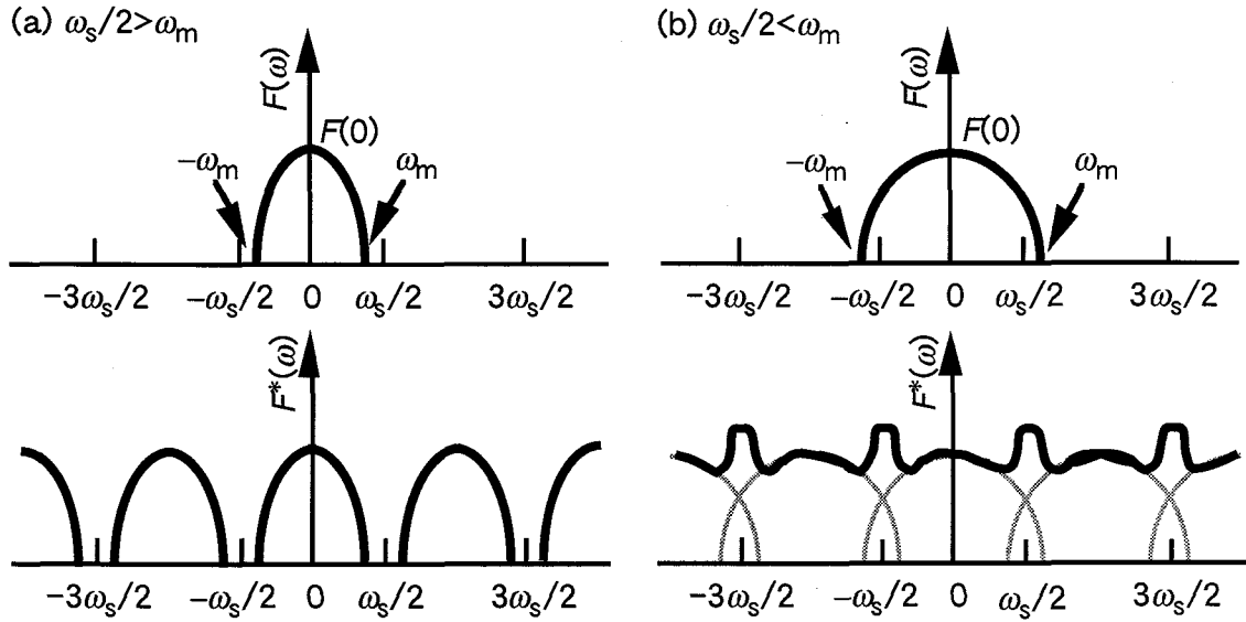
図3.2.4 入出力信号の周波数スペクトラム。
