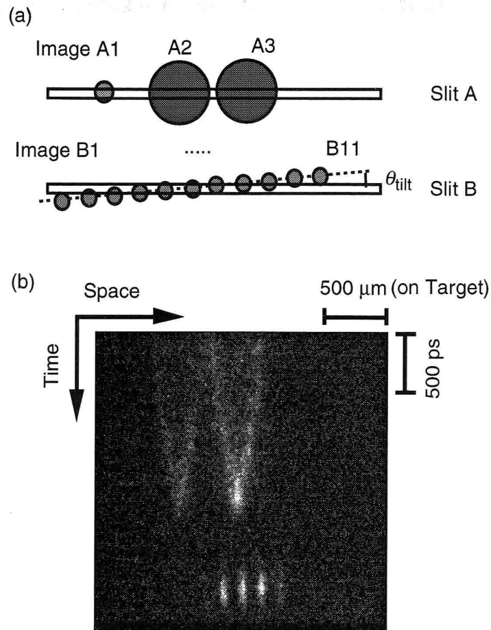
図3.4.1 一次元及びMIXS結像の原理. (a) イメージA1-A3はスリットA上に、イメージB1-B11はスリットB上に角度 \theta_{\text{tilt}} だけ傾けて結像する. (b) 1D+MIXS法で得られた時間掃引画像.
