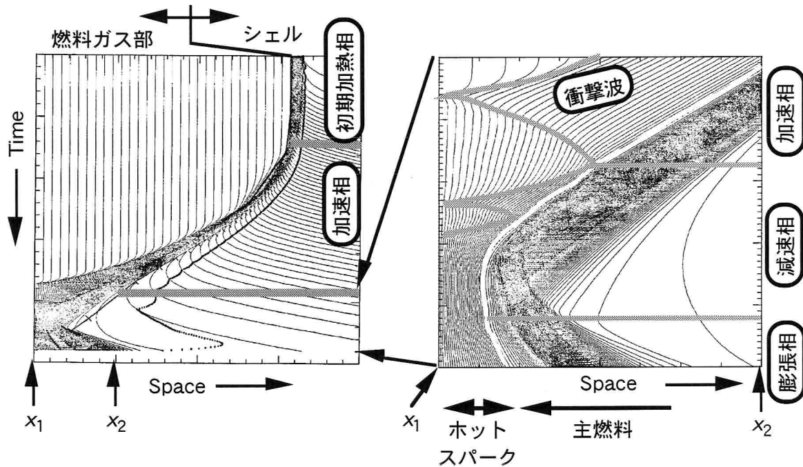
図2.2.1 一次元流体コード” ILESTA_1D” による爆縮過程全体のダイナミクス(a)と爆縮最終段階の拡大図(b).
