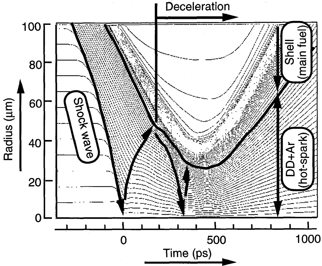
図3.5.4 一次元シミュレーション・コードによる爆縮最終段階の流線図。衝撃波がターゲット中心で衝突する時刻を t=0 とした。シェルが減速開始時刻は t=180 ps付近である。
