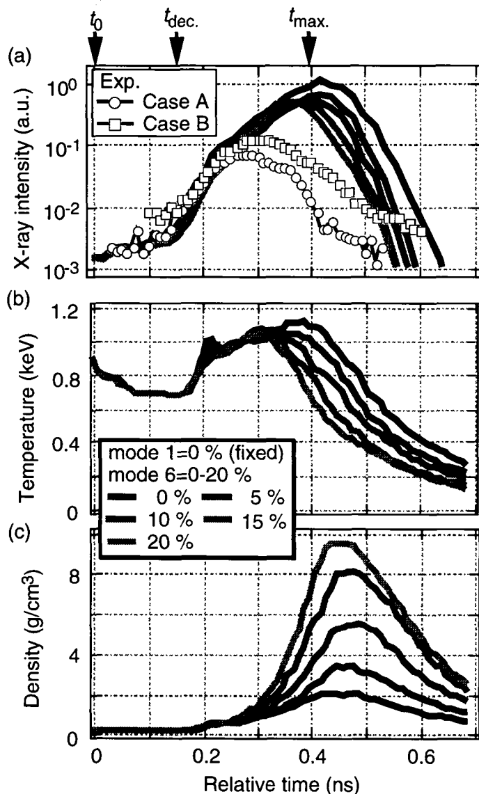
図4.3.8 NU_1=0, NU_6=0-20\% に対するX線発光強度 (a), 温度 (b), 密度 (c) の時間発展を示す。各時間プロファイルは図4.3.3と同じ手法で表示している。
