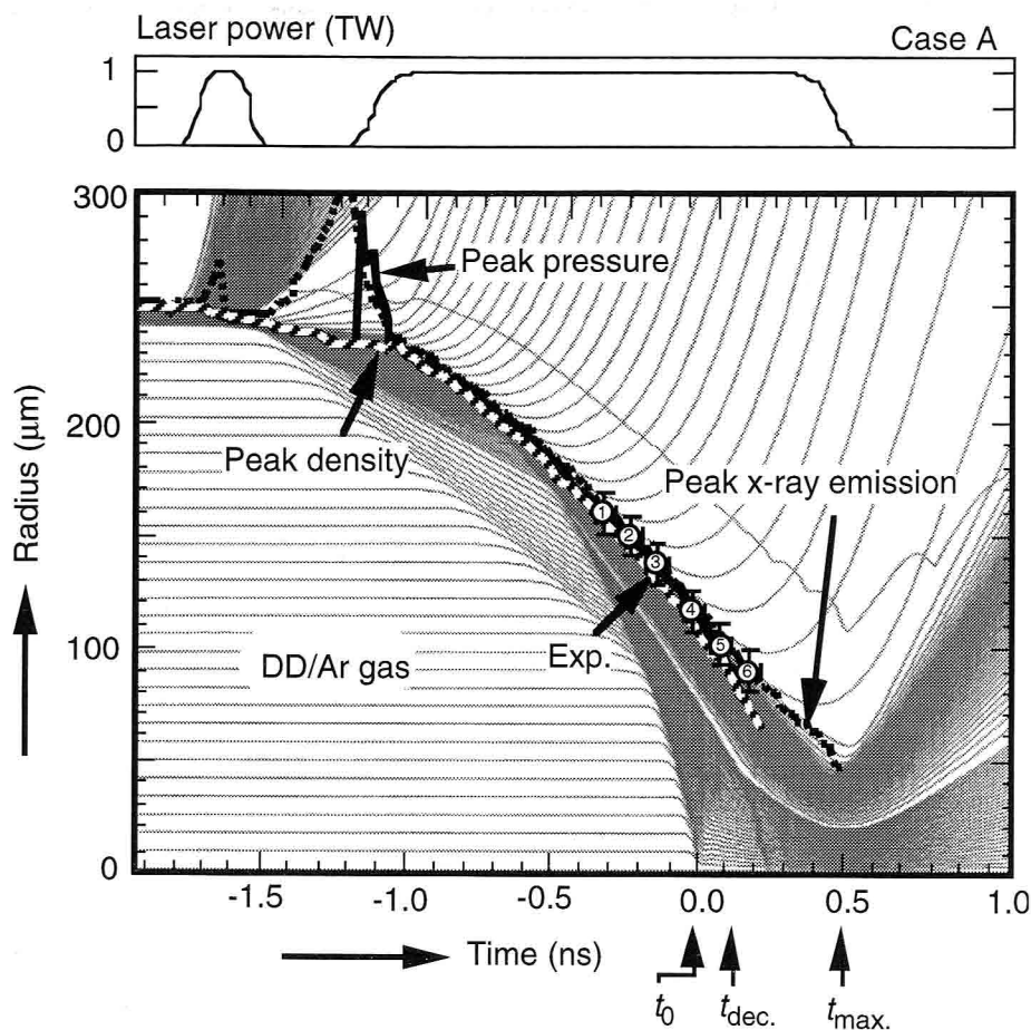
図4.2.4 ILESTA_1DによるCase Aに対する流線図。また、最大X線発光位置、最大圧力位置、最大密度位置のシミュレーション結果と最大X線発光位置の実験結果の時間軌跡を示す。衝撃波が中心で初めて衝突する時刻を t=t_0 ( =0 ns)、減速開始時刻を t=t_{dec} 、最大圧縮時刻を t=t_{max} として表示する。
