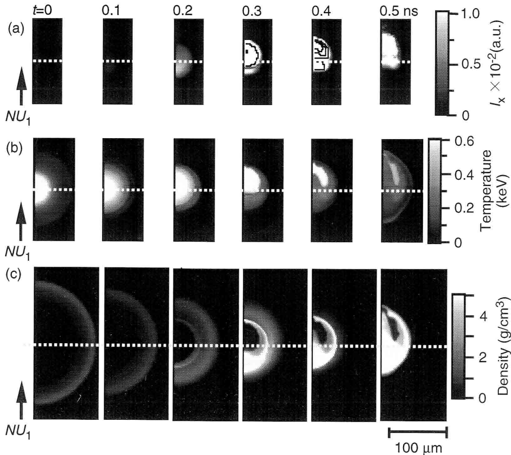
図4.3.2 二次元シミュレーションによる NU_1=18\% , NU_6=0 に対する二次元X線画像 (a), 温度分布 (b) 及び密度分布 (c). 二次元X線画像の等高線は発光強度0.04 a.u.の間隔で表示している.
