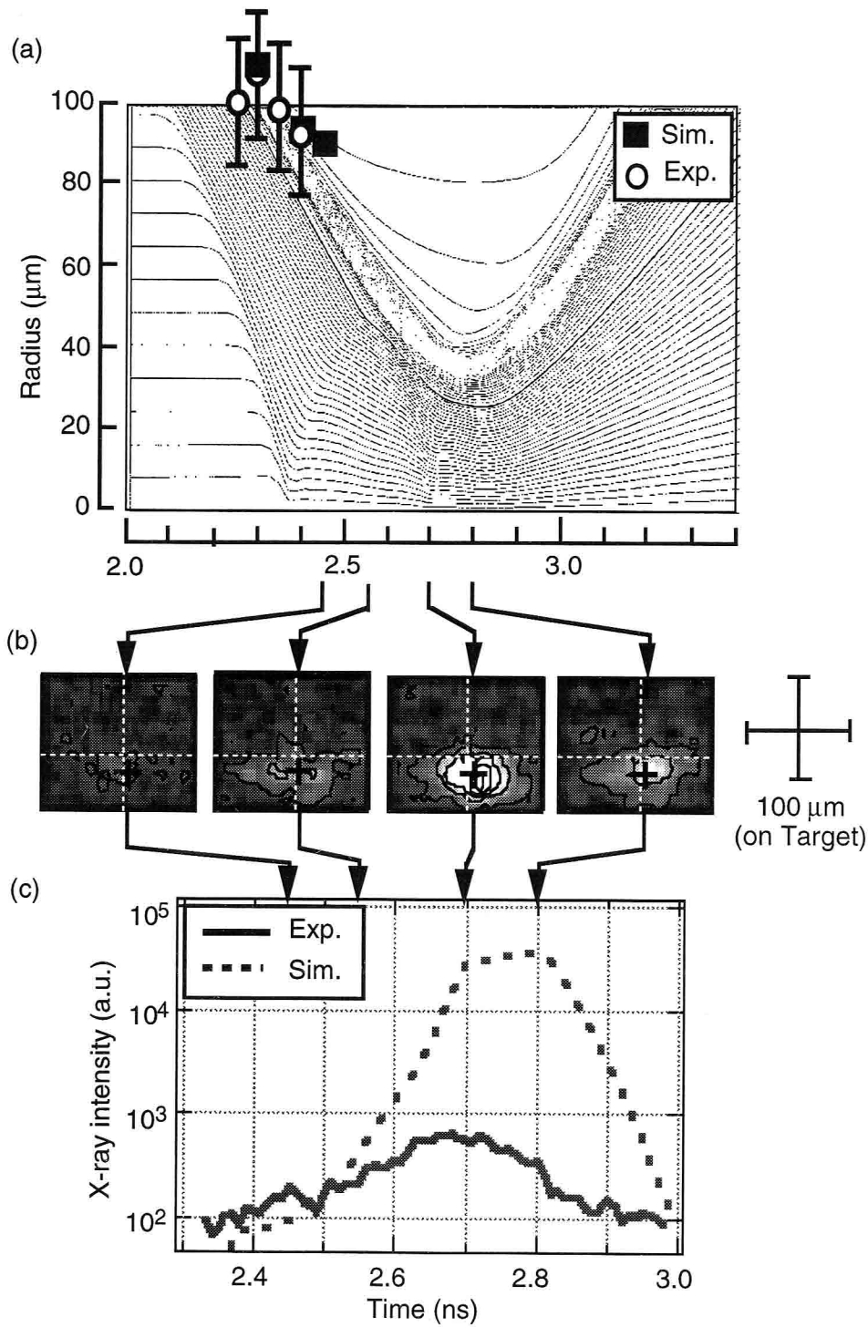
図3.4.3 1D+MIXS法で得られた実験結果と一次元シミュレーション予測との比較. (a) 一次元シミュレーション・コードによる爆縮最終段階での流線図. シェルのX線発光ピーク位置において, 実験結果とシミュレーション結果を一致させた. (b) t=2.45, 2.55, 2.70, 2.80 nsでの再構成された二次元X線画像. 白い点線の交点はチャンバー中心を, 実線はコア中心を示している. (c) コア中心でのX線発光強度の時間プロファイル比較.
