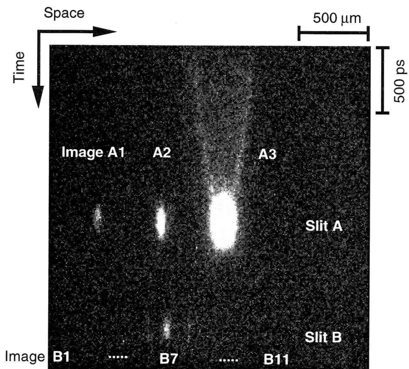
図4.2.6 1D+MIXS法で得られたCase Bに対する時間掃引データ。図中のImage A1-A3, B1-B11, Slit A, Bは図3.4.1 (a)で示したものに対応している。
