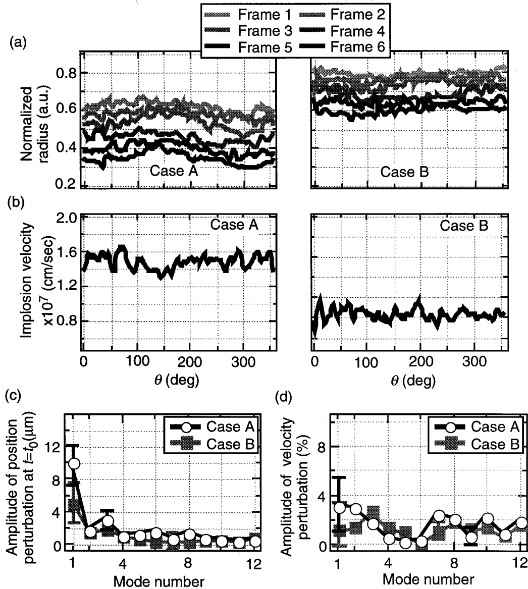
図4.2.5 爆縮途上のシェルの低次モード非一様性のモード解析結果. (a) 規格化した最大X線発光位置の円周方向プロファイル. (b) 爆縮速度の円周方向分布. (c) 時刻 t=t_0 での発光位置のモード展開結果. (d) 爆縮速度のモード展開結果.
