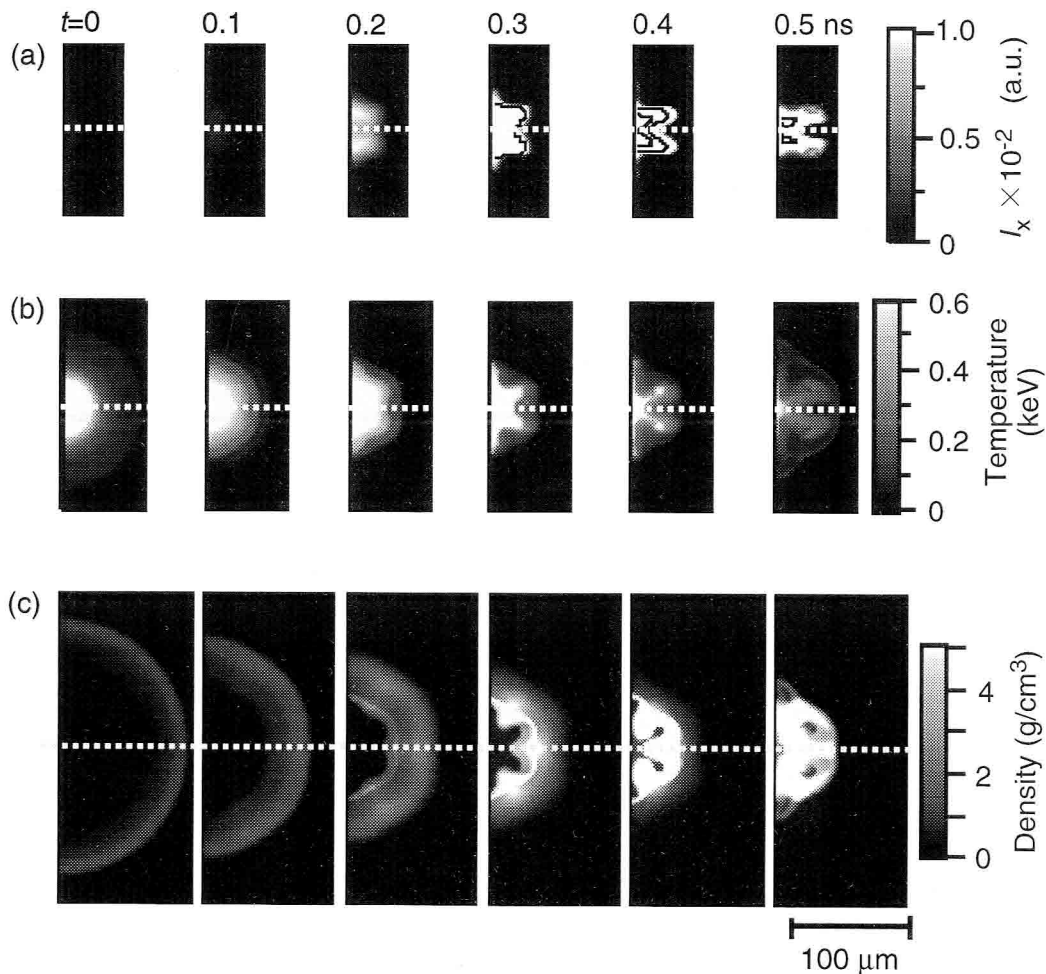
図4.3.7 二次元シミュレーションによる NU_1=0, NU_6=5\% に対する二次元X線画像 (a)、温度分布 (b) 及び密度分布 (c)。二次元X線画像の等高線は発光強度0.25 a.u.の間隔で表示している。
