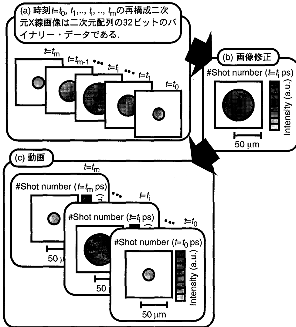
図3.7.1 時間的に連続する多数枚の二次元画像を順次コンピューター画面上に表示させ、動画化を行う。(a) 二次元画像は各時刻ごとにバイナリー・データ形式で保存される。(b) 各時刻の二次元画像に対し画像修正等を行いPICTファイルとして保存する。(c) 任意の動画速度(各コマ間隔時間)での二次元画像の動画をQuickTime形式で作成する。
