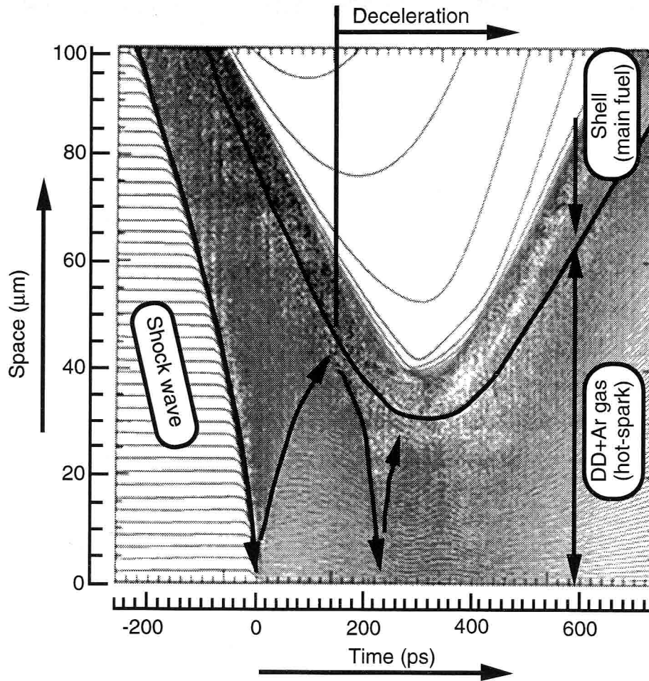
図3.3.20 ILESTA_1Dによる d/R=4 に対する爆縮の最大圧縮近傍の様子（流線図）。 t=0 は内向きに伝播する衝撃波がターゲット中心で衝突する時刻を示している。
