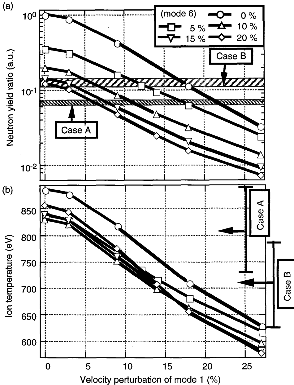
図4.3.1 二次元シミュレーションによる NU_1 及び NU_6 に対する中性子イールド (a) とイオン温度 (b) の依存性. Case A, Bの実験結果も示す.
