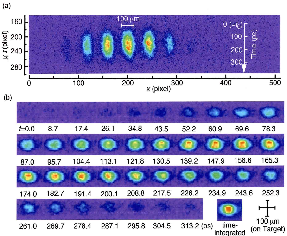
図3.3.21 MIXS法による爆縮コア・プラズマ・ダイナミクス診断。(a)時間掃引データ。時刻は図3.3.20での一次元シミュレーションによるものであり、 t=0 は衝撃波がターゲット中心で衝突する時刻を示している。(b)再構成された爆縮コア・プラズマの時間分解された二次元画像。フレーム時間間隔は8.7 psである。
