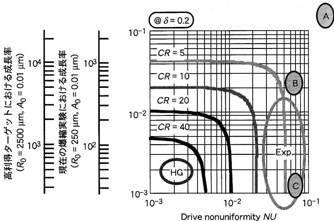
図2.3.2 規格化したR-T不安定性の成長率 GF_0 、レーザー照射強度非一様性 NU 、半径圧縮率 CR によって記述したスパーク形成条件 ( \delta=0.2 )。HG, Expはそれぞれ高利得ターゲット、現在の爆縮実験に対するパラメータ領域を示している。また、A, B, Cはそれぞれ3.3.4節、3.4及び3.5節、4章で述べる爆縮実験に対するパラメータ領域を示している。
