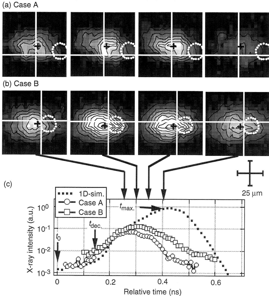
図4.2.8 McMIXS法によって観測されたCase A, Bでの実験結果. Case A, Bの爆縮コアの時間分解二次元X線画像をそれぞれ(a), (b)に示す. 白い線の交点がチャンバー中心を, 黒い十字の交点がコア中心を示している. McMIXS観測平面に投影したXPCのコア位置を破線の円によって \pm 15 \mu\text{m} 程度の精度で示す. 図中の等高線表示は192カウントの発光強度の間隔で表示している. (c) 爆縮コア中心でのX線発光強度の時間発展比較. 表示した時刻は図4.2.4の一次元シミュレーションの時刻に対応している. 球心衝撃波が中心で初めて衝突する時刻を t=t_0 ( =0 \text{ ns} ), 減速開始時刻を t=t_{\text{dec}} , 最大圧縮時刻を t=t_{\text{max}} でそれぞれ示す.
