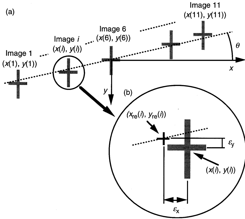
図3.3.8 静止画像モードの画像歪み評価手法。(a) マルチピンホール結像による11個の十字ターゲット全体の時間積分画像。(b) i 番目の画像の拡大図。
