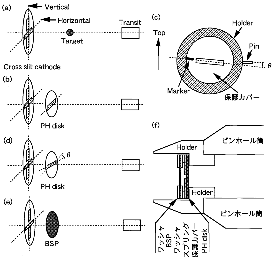
図B.2 ピンホール先端部の初期アラインメント. (a) 十字カソードの中心、チャンバーの中心、レチクルの中心を同一軸に持ってくる. (b) ピンホール列を水平方向のスリットに平行にする. (c) ピンホール・ディスク正面図. ピンホール列をピンに対して \theta だけ時計回りに回転させる. (d) ピンホール・ディスク中心をレチクル中心に合わせる. (e) BSPを取り付ける. (f) ピンホール先端部の断面図.
