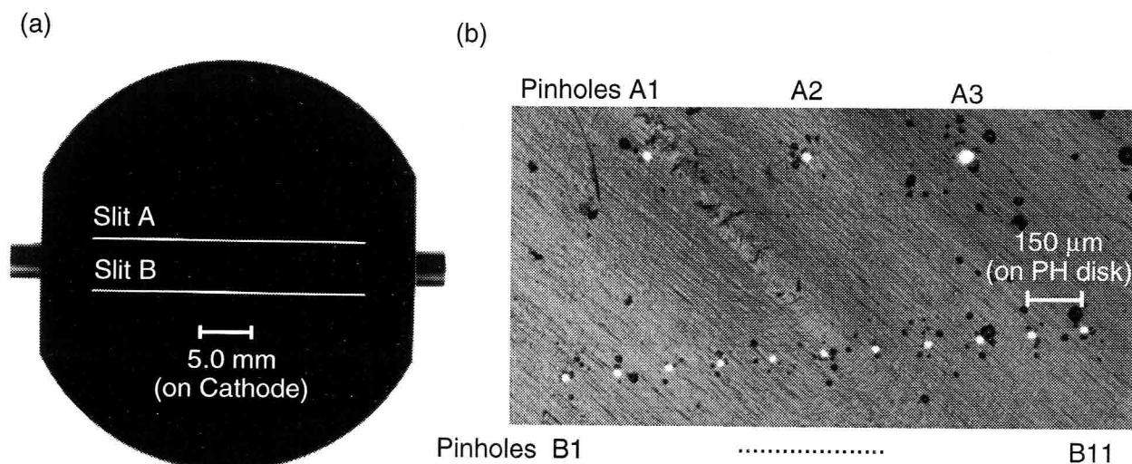
図3.4.2 1D+MIXS法で用いたカソード・ディスク (a) とピンホール・ディスク (b) の写真。
