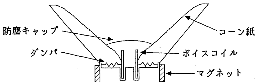
図2.2.1 コーン型スピーカの構造
