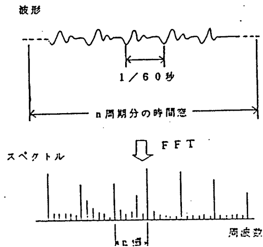
図2.3.9 ブレードとびの周波数領域的検出法
