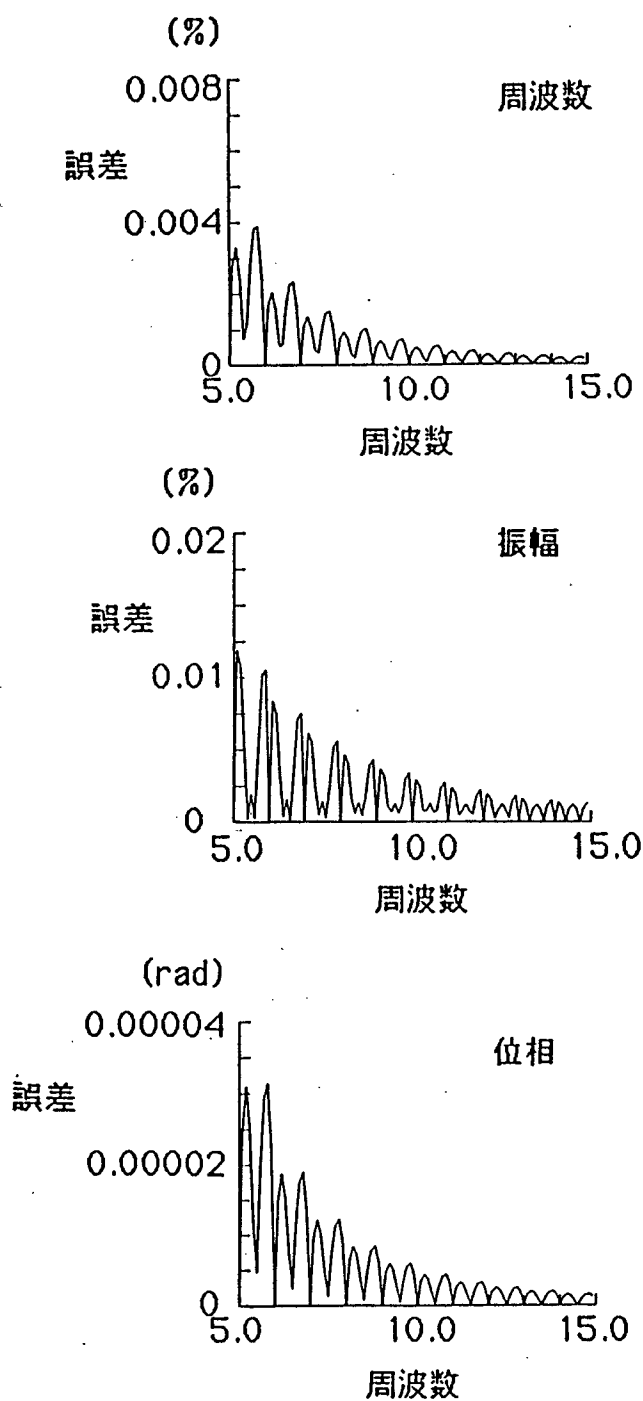
図1.5.3 推定スペクトル除去法による干渉除去後の単一周波数成分の同定精度
