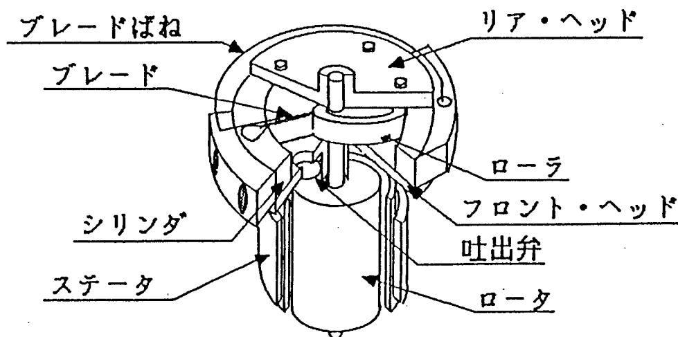
図2.3.1 冷房用ロータリ型圧縮機の構造
