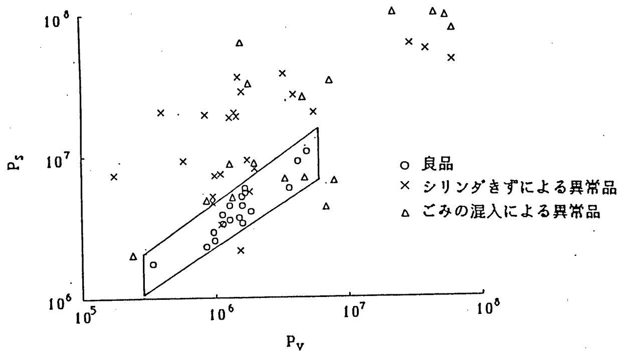
図2.3.12 シリンダきず，ごみの混入による異常品の検査結果
