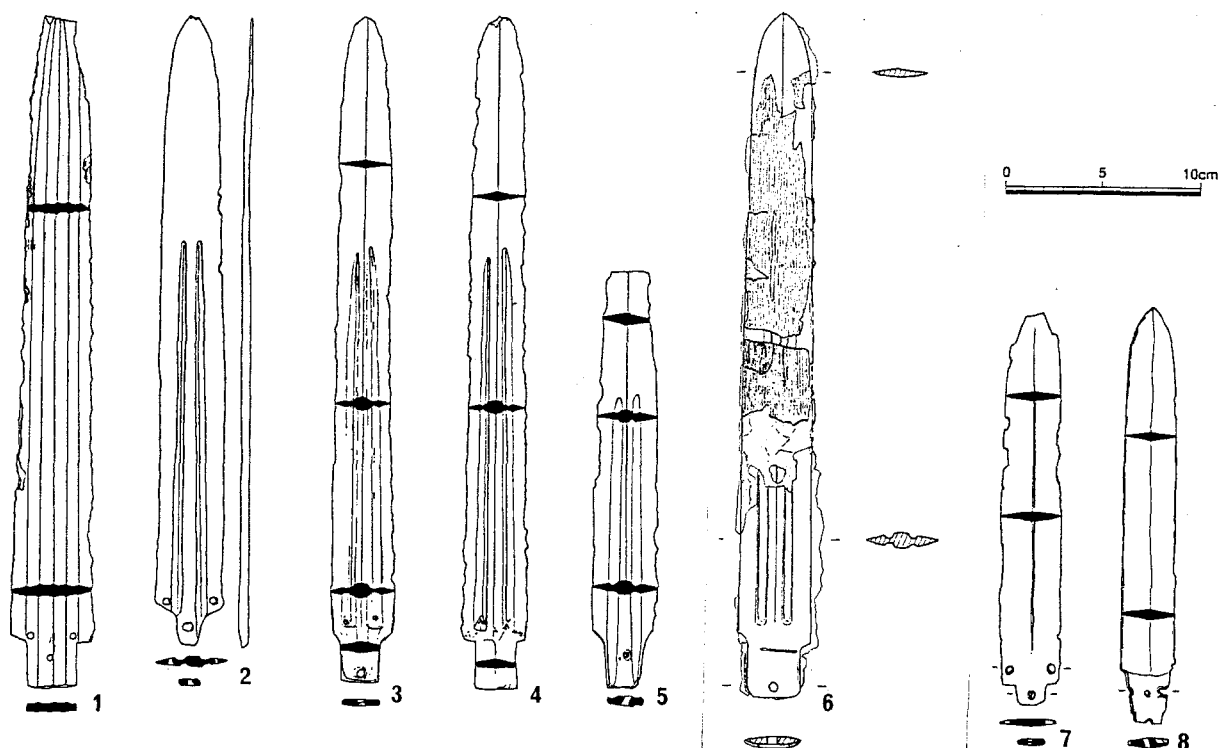
図31 弥生時代後期(併行期)以降における細身薄型銅剣( S = 1/4 )
