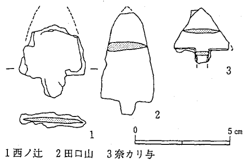
図20 近畿地方の有茎式鉄鋤 (S = 1/2)
