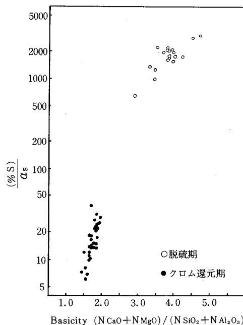
図 3-28 硫黄分配比におよぼす塩基度の関係 46) 47)
