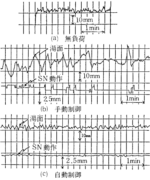
図5－8 115mm角の鑄片の鑄造時における鑄型内の溶鋼の湯面制御例 70) 71)
