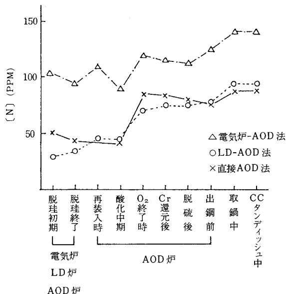
図 3-16 各種操業法における溶鋼中の窒素の挙動 33)
