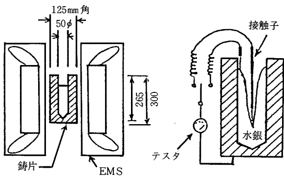
図 5－11 水銀を用いた攪拌実験装置および測定法 69)75)
