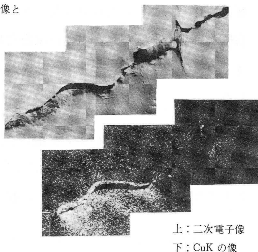
写真 5-7 SUS 310 の割れ発生部 における銅の析出状況 ( \times 165 ) 68) 69)
