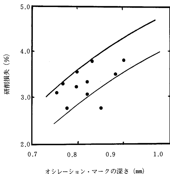
図5-1 オシレーション・マークの深さと研削損失の関係 59)
