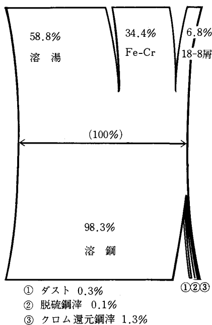
図4-2 30トンアルゴン・酸素脱炭炉における ステンレス鋼製造時のクロムの物質精算 図 60)
