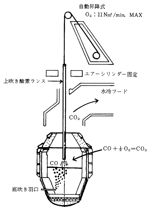
図3-8 30トンアルゴン・酸素脱炭炉の上吹き酸素設備の概要図
