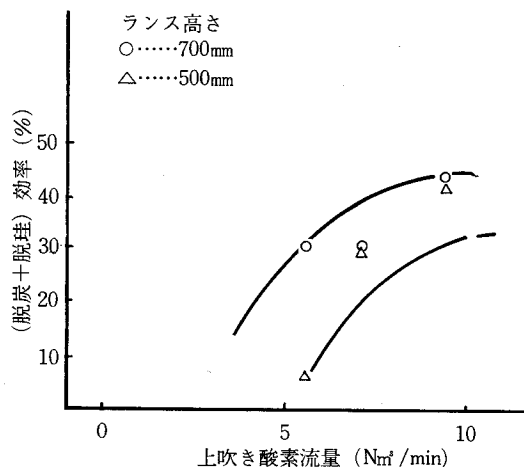
図 3-11 上吹き酸素流量と(脱炭+脱珪)効率の関係 33)
