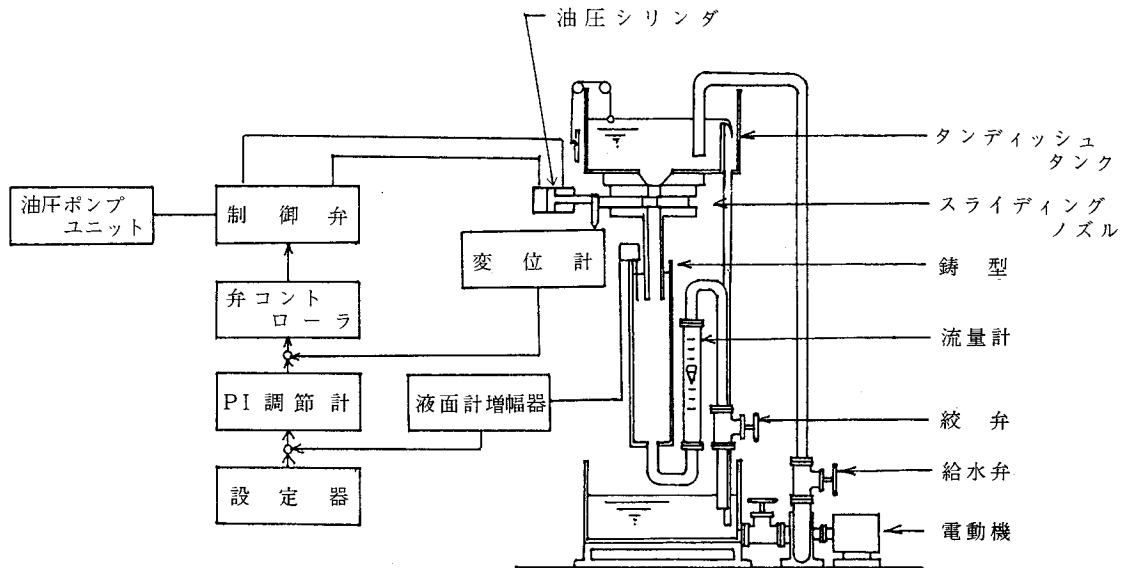
図5-5 鑄型内の溶鋼の湯面の自動制御系を開発するための実験装置の概略図 67)
