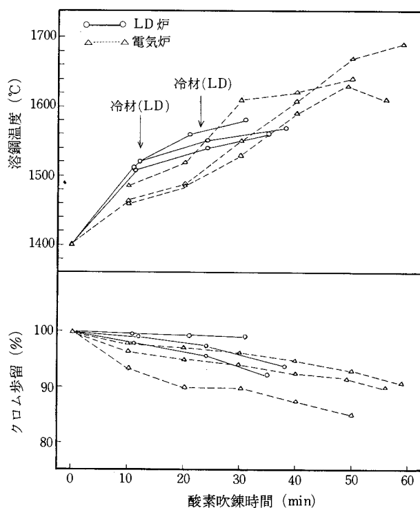
図3-7 酸素吹錬中の溶鋼温度およびクロム歩留の変化 46)
