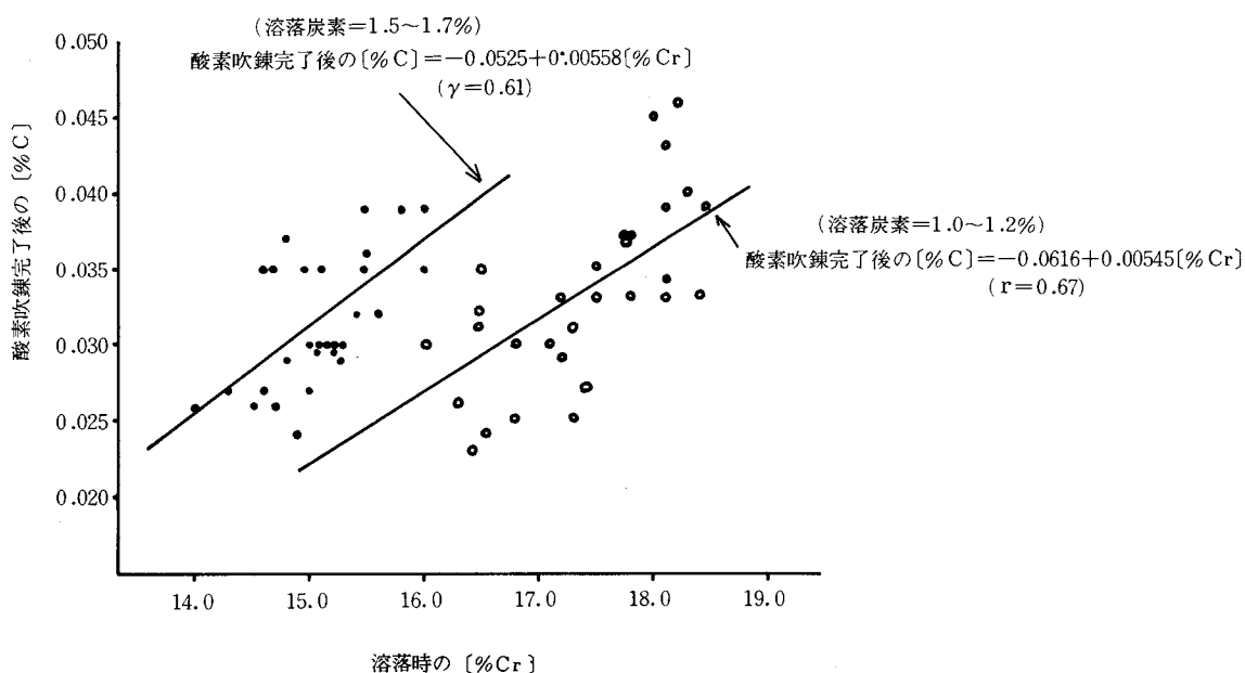
図2-3 酸素吹錬完了後の炭素含有量、溶落時の炭素含有量およびクロム含有量の関係 (20トン電気炉)
