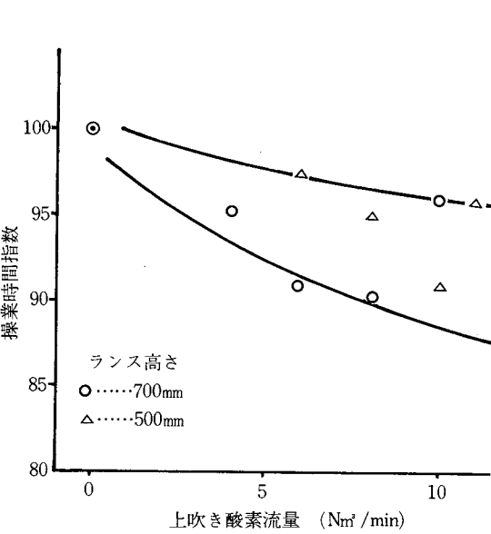
図3-12 上吹き酸素流量と操業時間の関係
