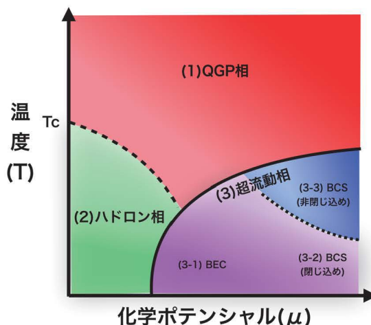
図 1:有限温度・密度 2 カラーQCD の相構造予想図
