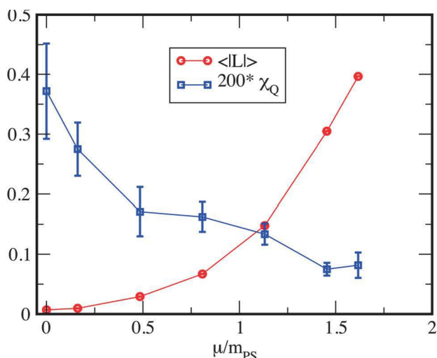
図 5: T=0.87T_c でのポリヤコフープ(赤)とトポロジカル感受率(青)の密度依存性
