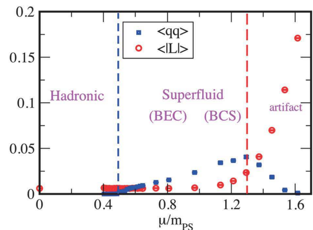
図2: T=0.43T_c におけるポリヤコフープ(赤)とダイクォーク凝縮(青)の化学ポテンシャル依存性
