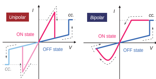
単一電圧極性で駆動可能な抵抗変化メモリ（左・ユニポーラ型）と駆動に両電圧極性を必要とする抵抗変化メモリ（右・バイポーラ型）
