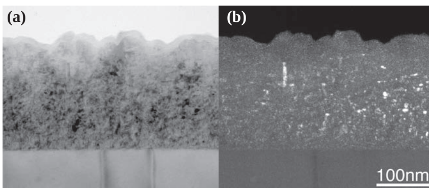
図 2. 低 Ga 分子線供給下で Gd を添加した GaN 薄膜の断面 TEM。(a) 明視野像。(b) 暗視野像 (GaN 以外の回折斑点から得た)。数 nm サイズのクラスターが GaN 中に析出している。
