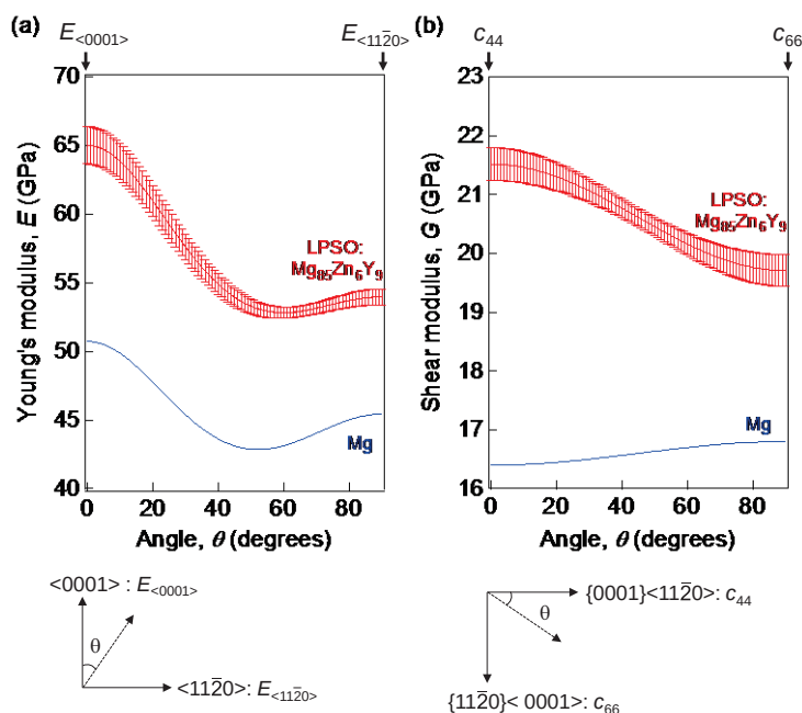
図 1 LPSO 構造を有する Mg 85 Zn 6 Y 9 合金と純 Mg の弾性率の結晶方位依存性: (a) ヤング率および (b) セン断弾性率。
