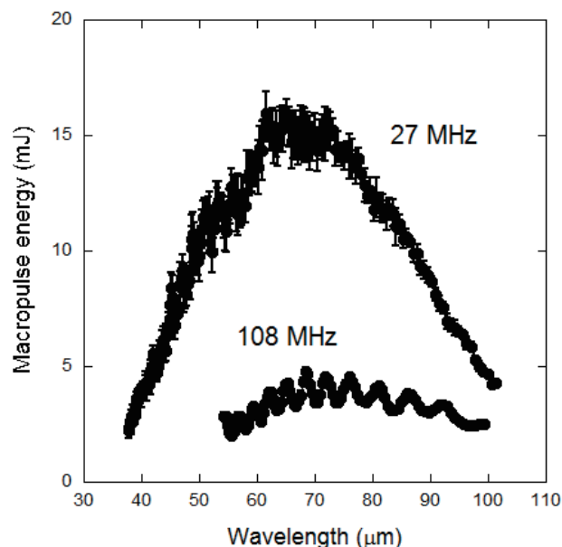
図2 27 MHz グリッドパルサーを用いた FEL 発振により得られたマクロパルスあたりの出力エネルギーの波長依存性。最大強度は現在のグリッドパルサーを用いた 108 MHz 繰り返しの場合と比べて約 4 倍に増加している。
