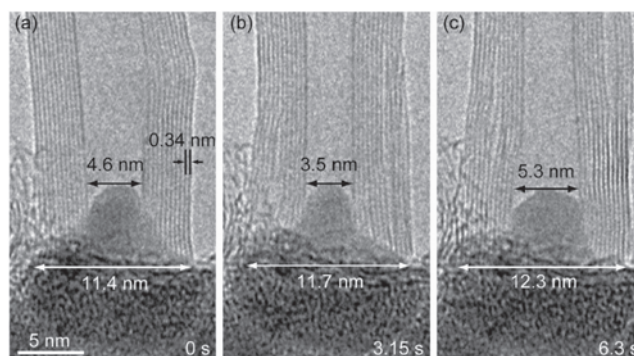
図 5 カーボンナノチューブ成長中の層間の変化
