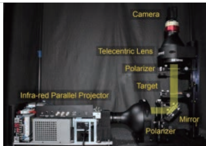
図2 計測装置
