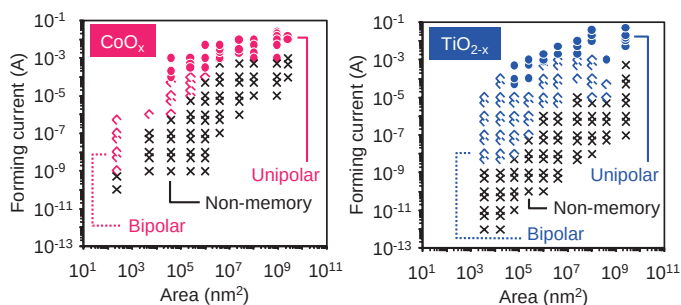
メモリ駆動方式の素子サイズ依存性（左・コバルト酸化物、右・チタン酸化物）
