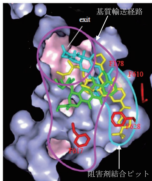
図 1 阻害剤結合部位の拡大図
