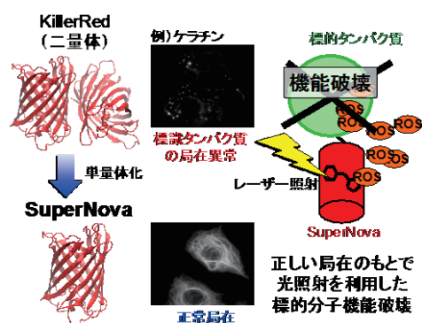
図 1 光増感蛍光タンパク質 SuperNova
