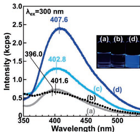
図3 エタノールに分散したシリコンナノ粒子のフォトルミネッセンススペクトル。(a) ビーズミル粉碎後に濾過したシリコンナノ粒子。(b) 42時間暗所でフッ化水素酸水溶液に浸漬して作製したシリコンナノ粒子のエタノール分散液の濾液。(c) 6時間および(d) 42時間、光照射しながらフッ化水素酸水溶液に浸漬して作製したシリコンナノ粒子のエタノール分散液の濾液。
