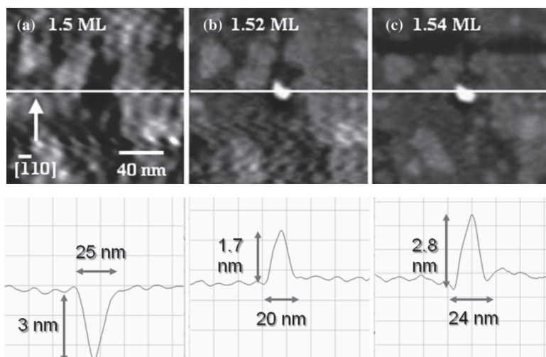
図 2 位置制御単一量子ドット作製：InAs 成長量と断面形状
