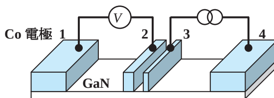
図 3. 作製した 4 端子非局所電気伝導測定素子の概略図。
