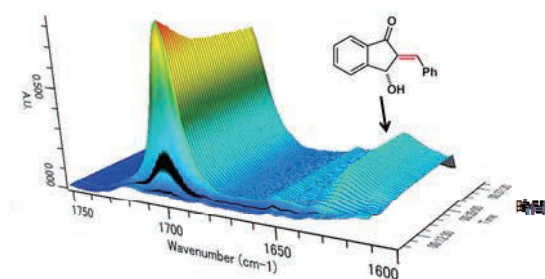
イリジウム錯体を用いるタンデム型不斉触媒反応
