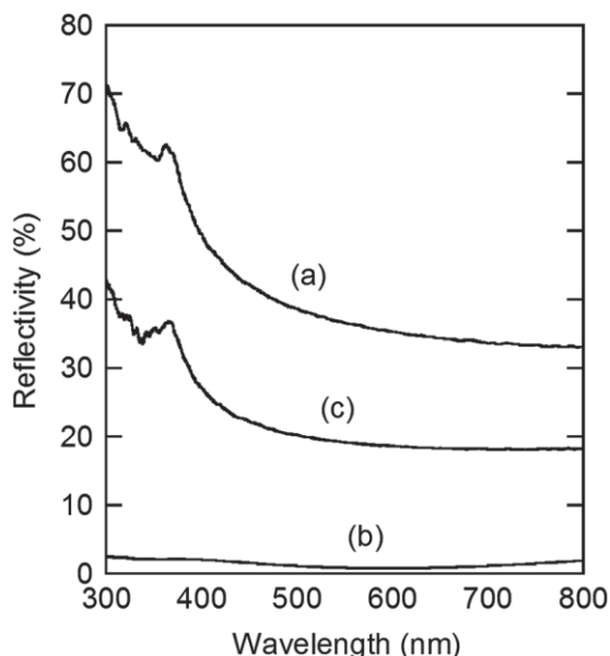
図1 SSCT法によりシリコンナノクリスタル層を形成する前(a)と後(b)のシリコン基板表面の反射率。(c)は、多結晶シリコン太陽電池で一般的に用いられている酸エッチングによるテクスチャー構造をもつシリコン表面の反射率。
