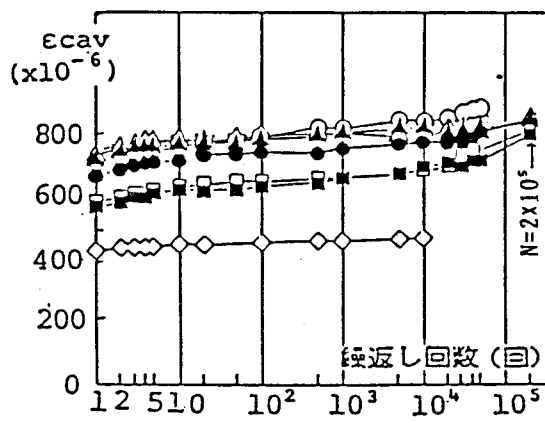
(c) 圧縮縁コンクリートひずみ \epsilon_{cav}
