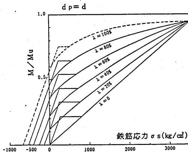
図2-27 曲げモーメント－鉄筋応力関係 ( M_u :一定, d p = d )
