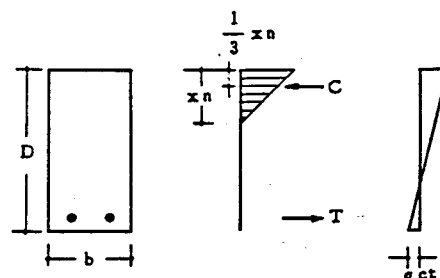
図4-5 ひずみ分布
