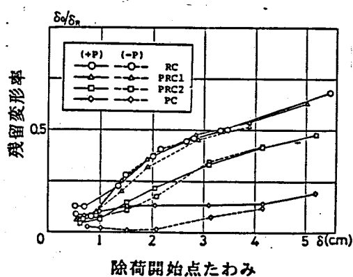
図2-21 残留変形率
