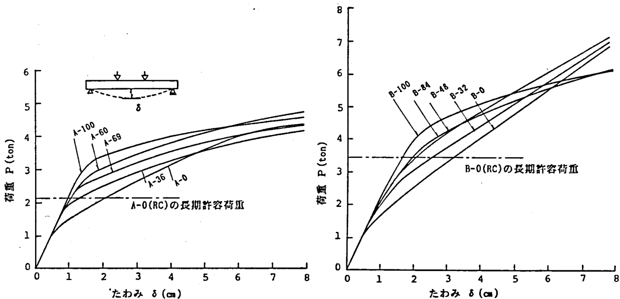
図2-3 荷重P－たわみ \delta 関係
