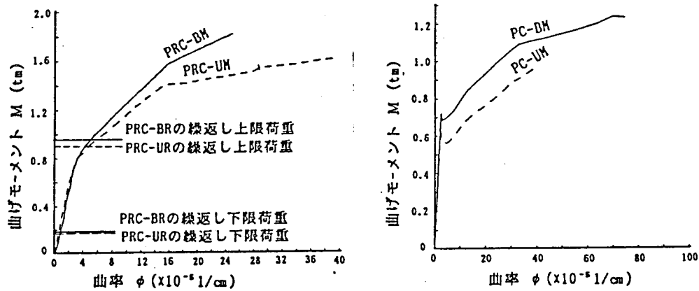
図 5-30 PRC 単調載荷試験体の M- \phi 関係
