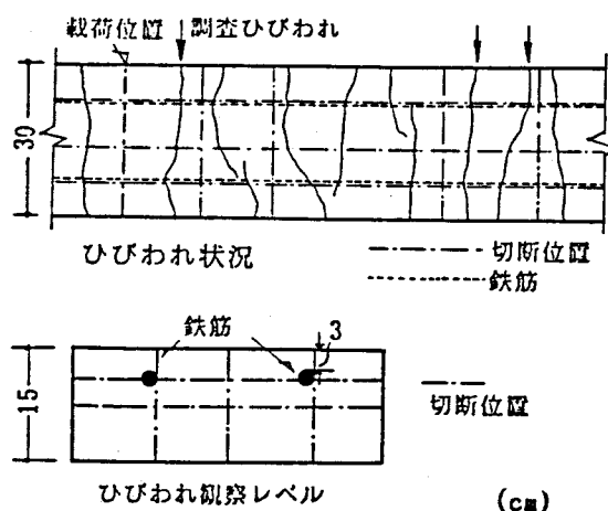
図4-24 コンクリート内部でのひびわれ形状を測定した試験体の形状、表面ひびわれ状況および切断位置
