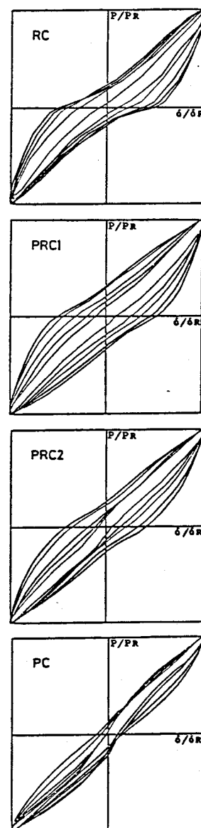
図2-19 履歴ループ形状
