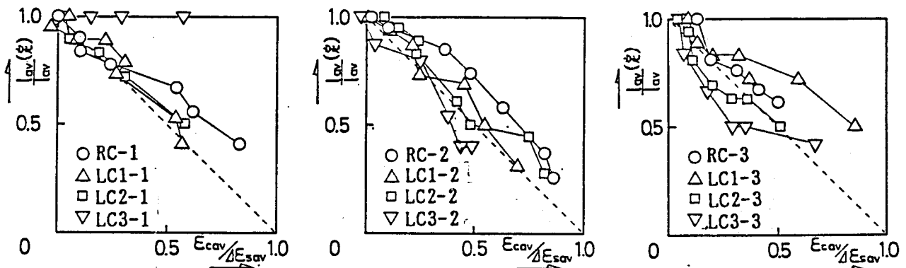
図 3-25 ひびわれ非定常状態における l_{av}(\epsilon)/l_{av} と \epsilon_{c.av}/\Delta \epsilon_{s.av} との関係
