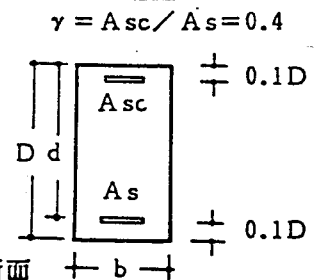
図7-18 はり断面
