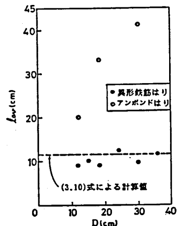
図4-3 平均ひびわれ間隔 l_{av} とはりせい D の関係
