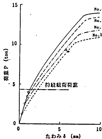
図6-40 単調荷試験体の荷重Pとたわみ \delta の関係
