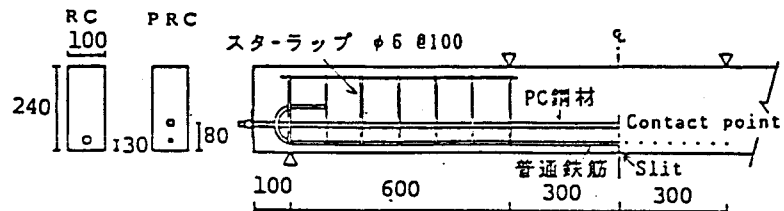
図5-28 はり試験体の形状
