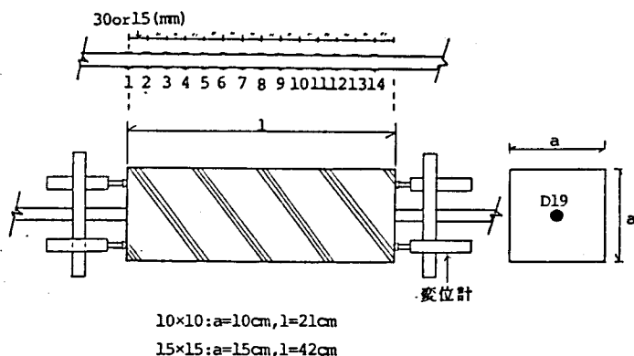
図5-5 試験体形状およびW.S.G貼付位置
