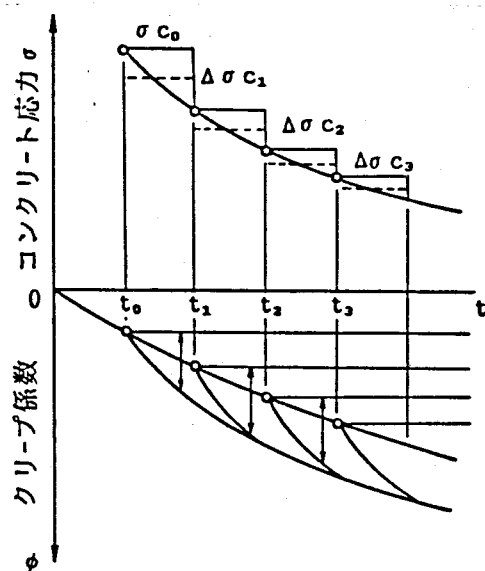
図6-25 応力、クリープ係数-時間の関係
