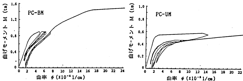
図 5-31 PC 繰返し載荷試験体の M- \phi 関係
