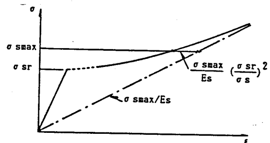
図3-17 CEB-FIP Code(1978)の平均鉄筋ひずみの算出法
