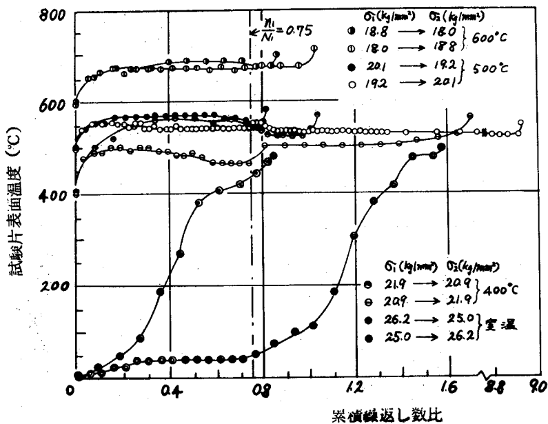
図1-2-9 二段二重複繰返し応力疲労過程中的試験片表面温度の変化
