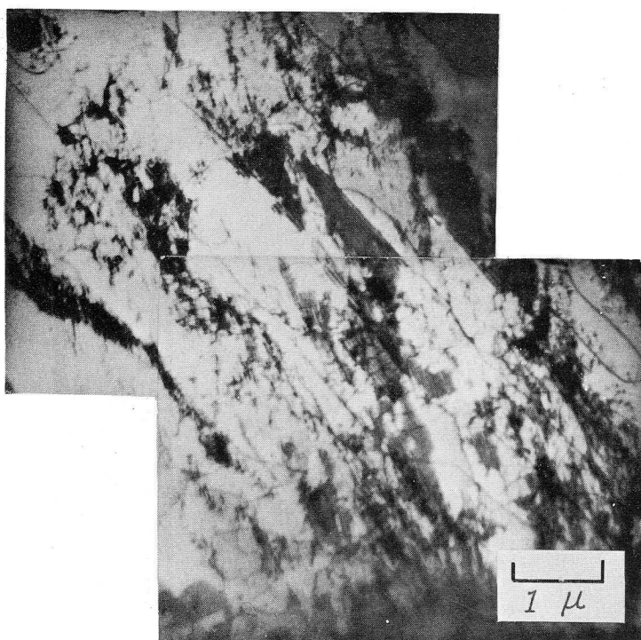
図 3-2-17 低応力疲労過程中的転位組織 \sigma = 2.4 \text{ kg/mm}^2 , N = 10^6
