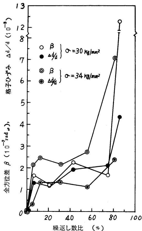
図2-2-6 疲労過程中的全方位差 ( \beta ) と格子ひずみ ( \Delta d/d ) の変化
