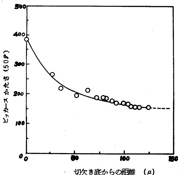
図 1-3-2 切欠き底部の硬度変化
