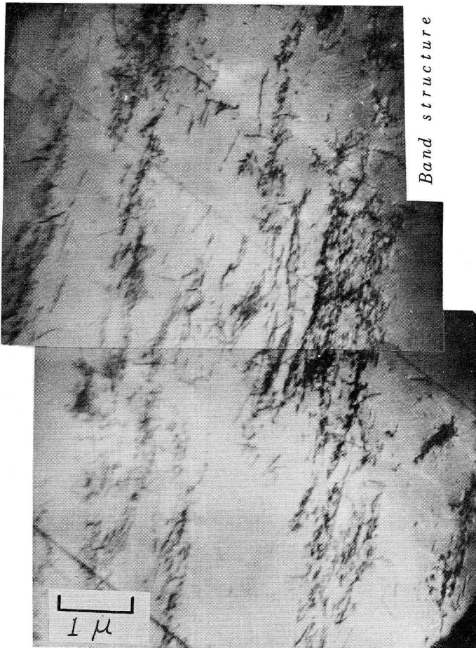
図3-2-9 低応力疲労過程中的転位組織
