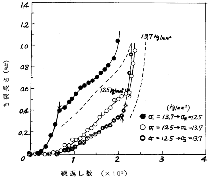
図 1-3-7 600℃における二段二重重複疲労過程中的き裂進展曲線
