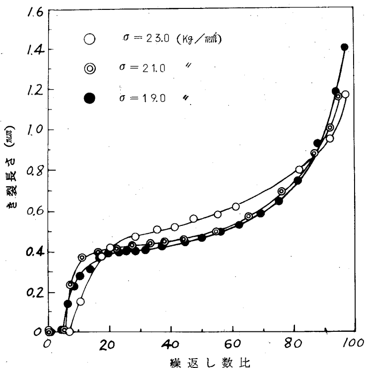
図1-3-13 き裂長さとの関係
