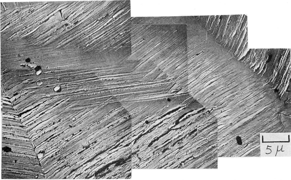
図2-4-13 すべり線中の析出物
