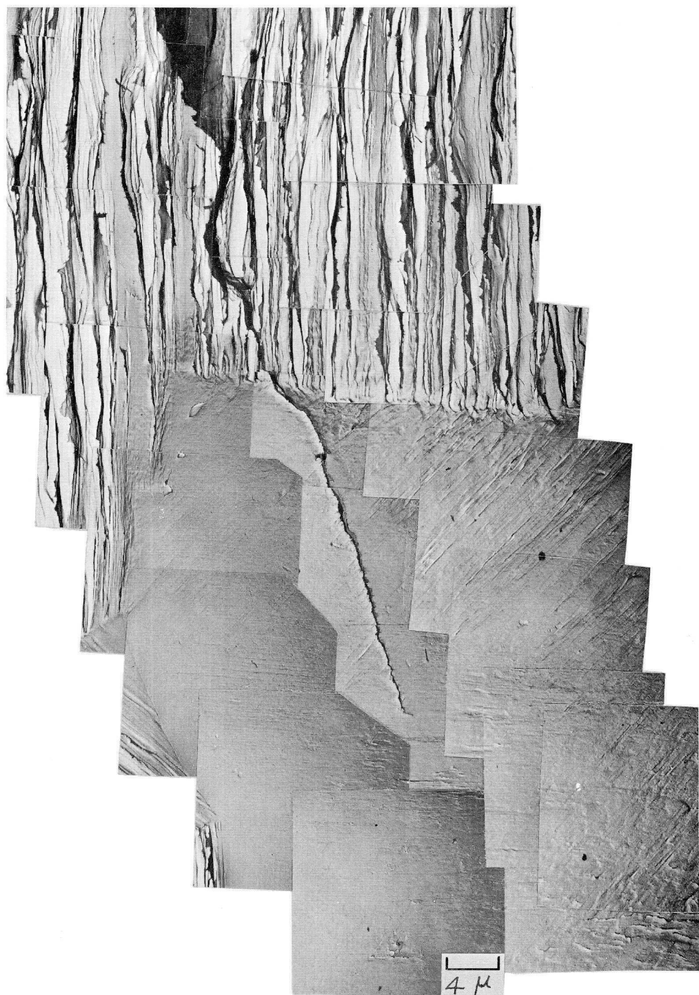
図2-4-7 Intrusion における疲労き裂の発生
