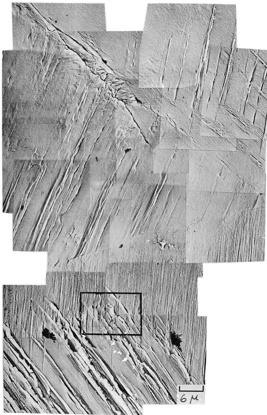
図2-4-9 結晶粒界近傍におけるき裂の発生
