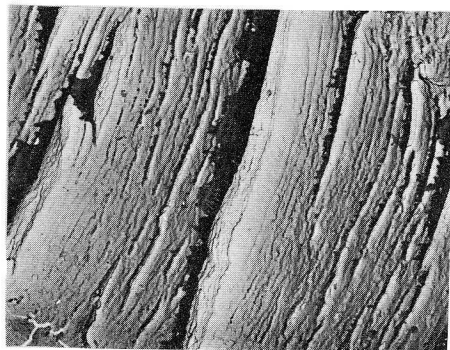
(d) T = 600^\circ\text{C} \sigma = 13.7 \text{ kg/mm}^2
