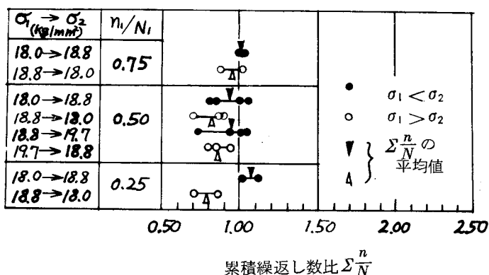
図1-2-7 二段二重重複疲労試験における累積繰返し数比
