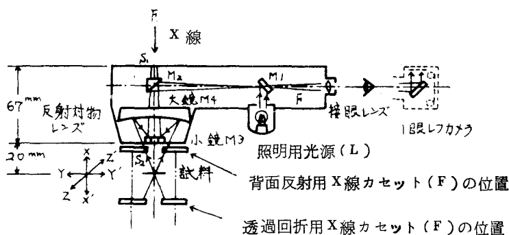
図 2-3-2 直視型マイクロビームカメラ構造図
