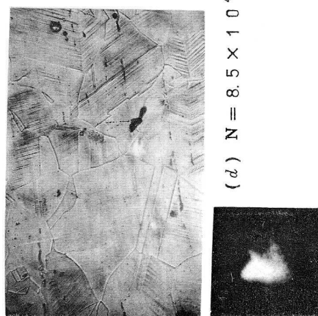
図 2-2-5 疲労過程における表面組織と X 線回折像の変化
