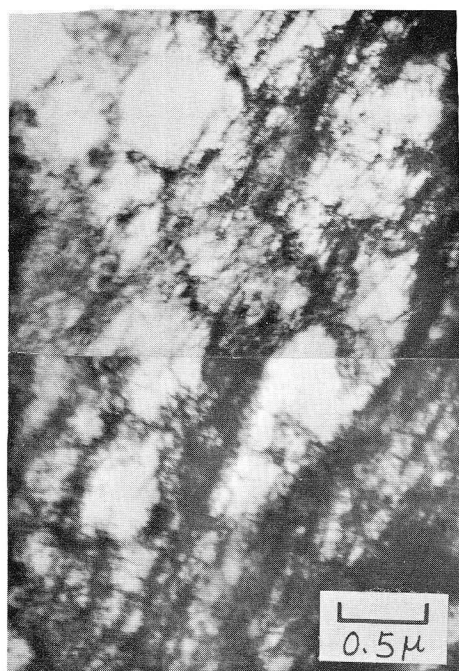
図 3-2-36 引張変形によって生じた Cell structure
