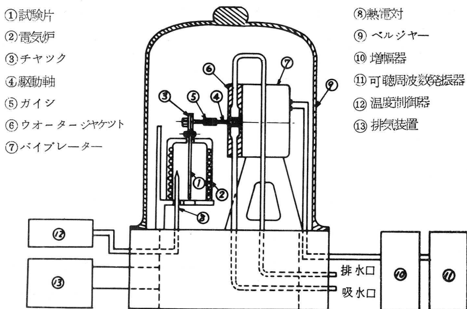
図 2-4-3 真空中高温用疲労試験機の概略図
