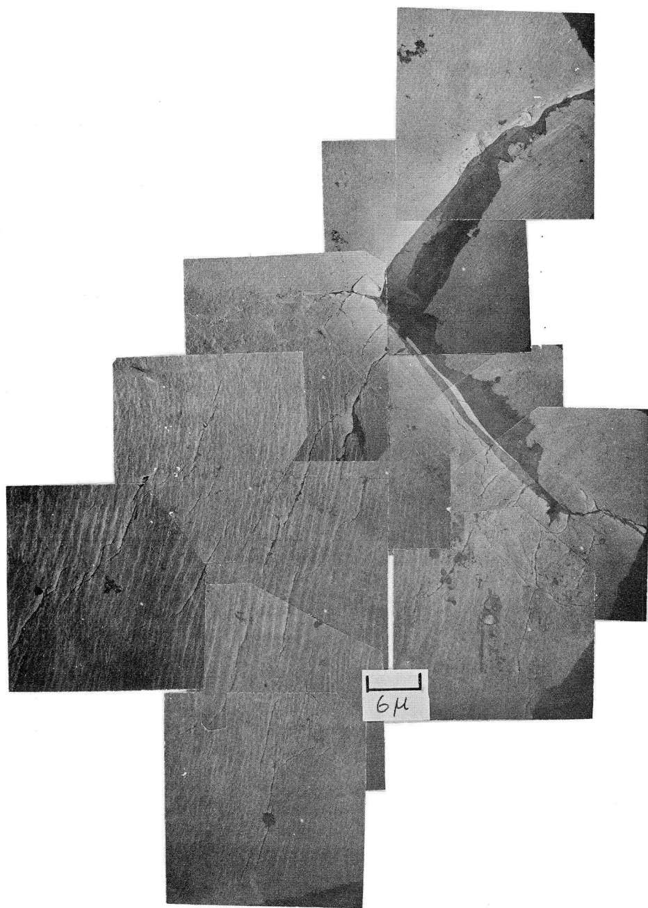
図 2-4-16 アルミニウムの疲労き裂近傍の変形組織
