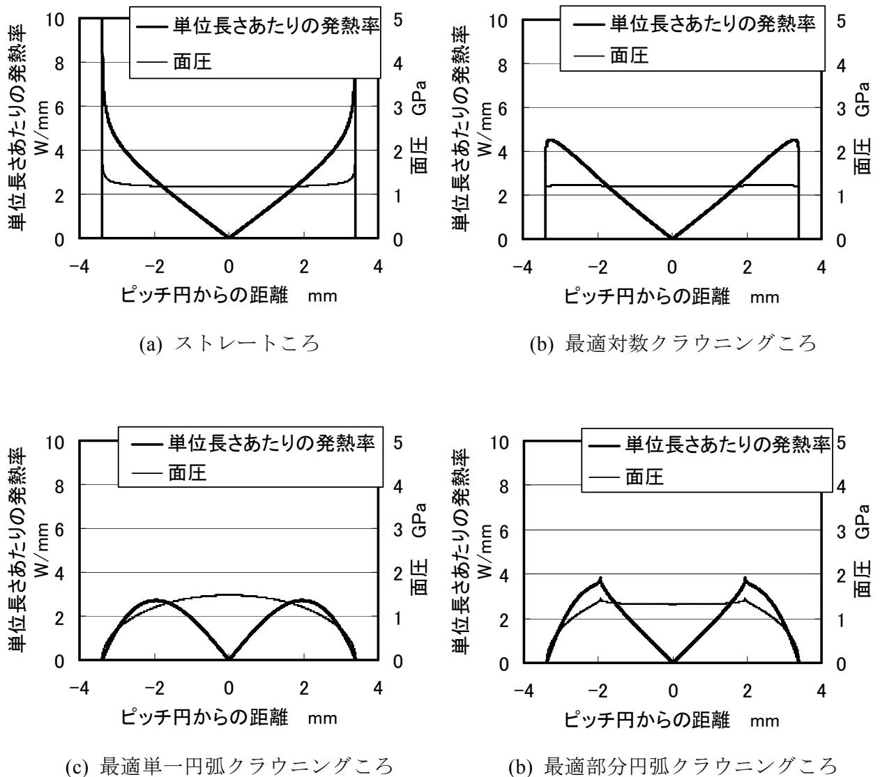
図 7-13 面圧と、スピンによる発熱の分布
