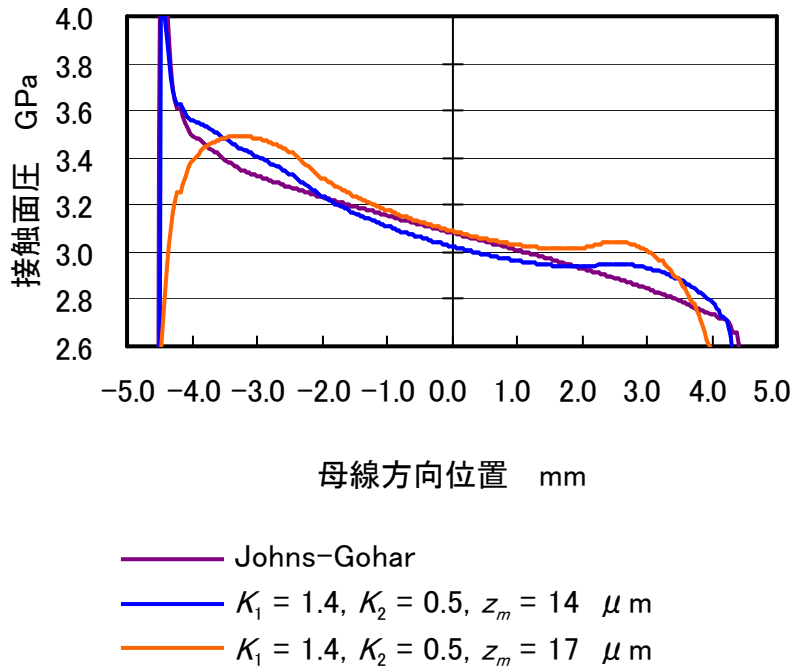
図 3-6 ころチルト角 0.001 rad のときの接触面圧
