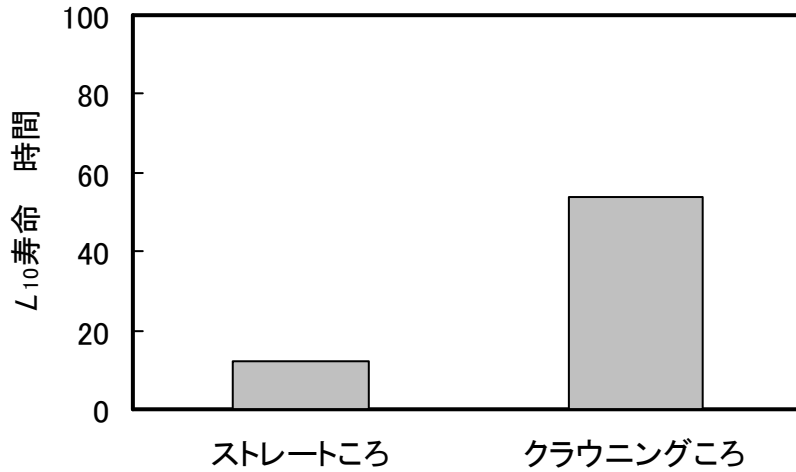
図 7-14 ストレートころとクラウニングころの寿命の比較
