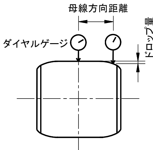
図 5-5 量産ラインにおけるドロップ量の測定方法
