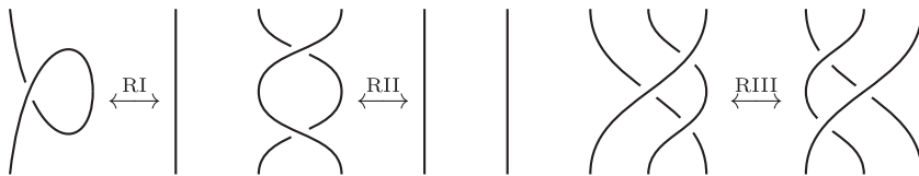
Fig. 2. Reidemeister moves
