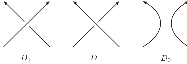
Fig.3. A skein triple
