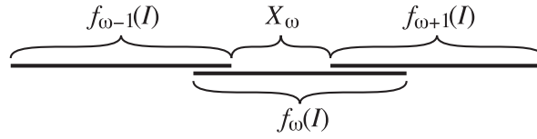
Fig.3. X_\omega
