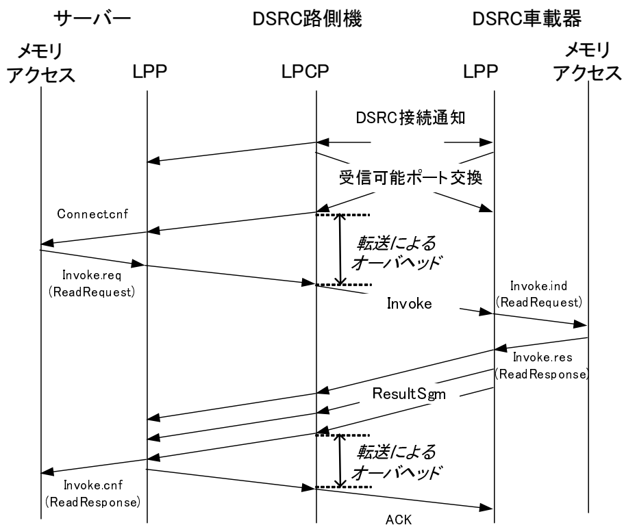
(b) メモリアクセスアプリケーションにおける通信シーケンス
