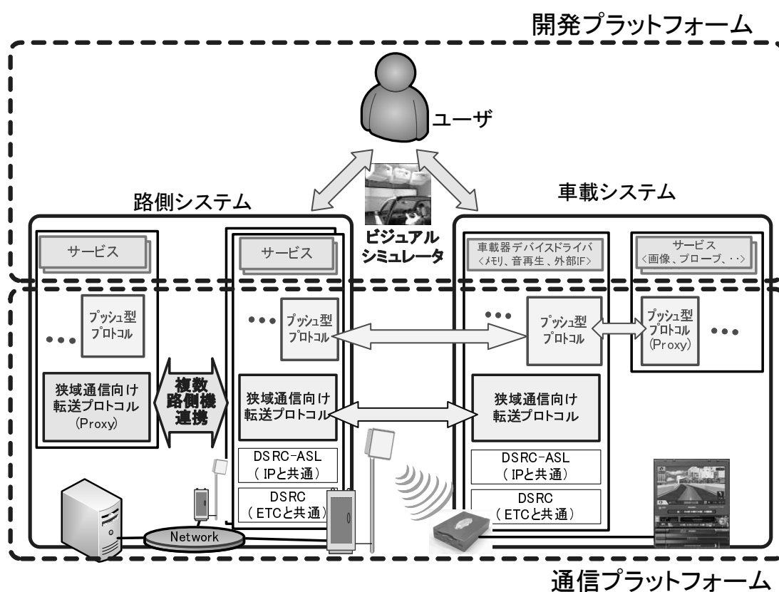
図 1.1: 路車協調システムのための通信プラットフォームの全体像
