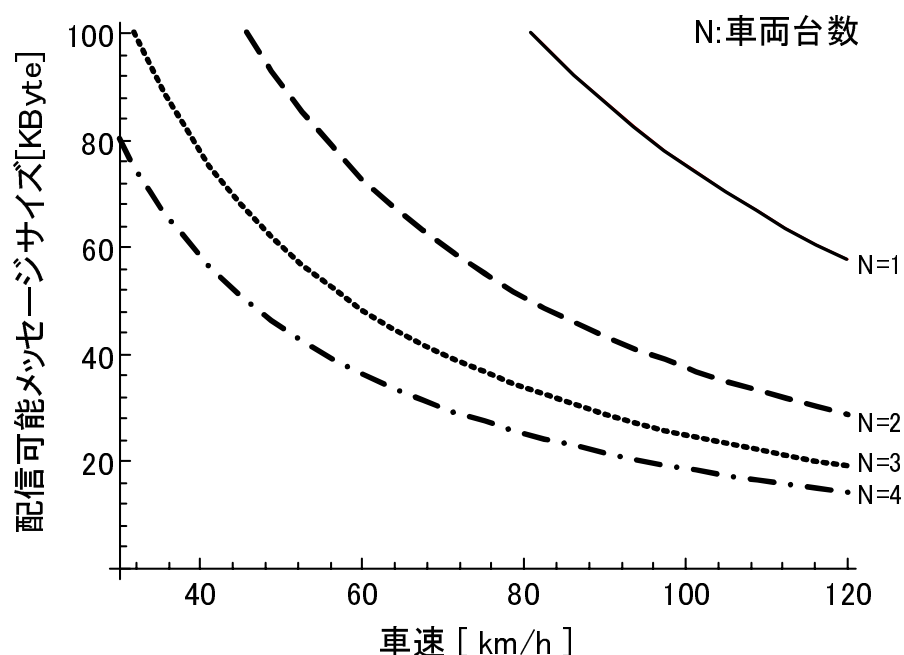
図 3.7: 1 台あたりの通信可能データサイズと車速の関係(通信エリア 20[m] の場合)
