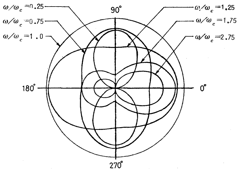
(a) H 波入射
