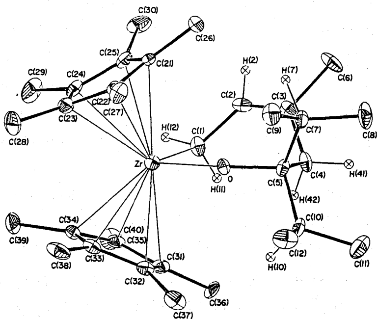
Fig. 2-6. Molecular structure of (\eta^5\text{-C}_5\text{Me}_5)_2\text{ZrOC}(i\text{-Pr})_2\text{CH}_2\text{CMe}=\text{CHCH}_2 ( 7 ).
