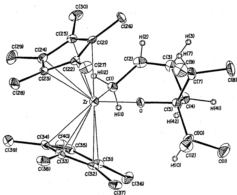
Fig. 2-5. Molecular structure of (\eta^5\text{-C}_5\text{Me}_5)_2\text{ZrOC}(i\text{-Pr})_2\text{CH}_2\text{CH}=\text{CHCH}_2 ( 6 ).
