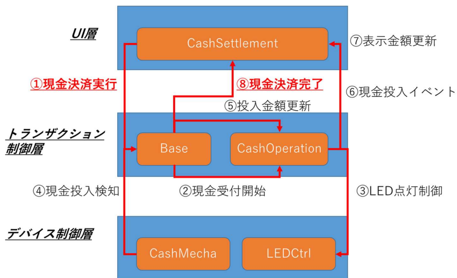
図 23 現金決済処理時のインタフェース例
