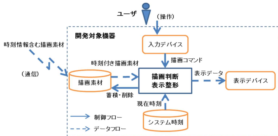
図 4 開発対象機器の構成
