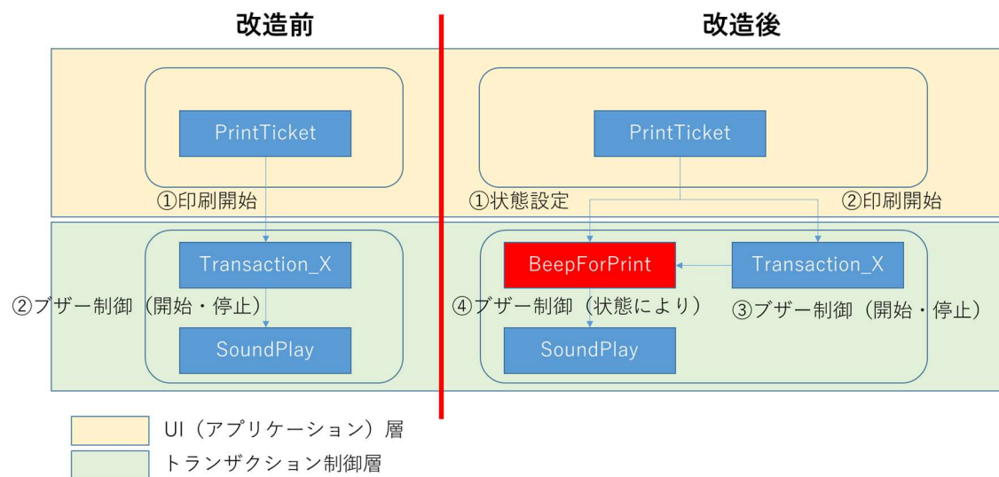
図 26 改造前後のソフトウェア構造
