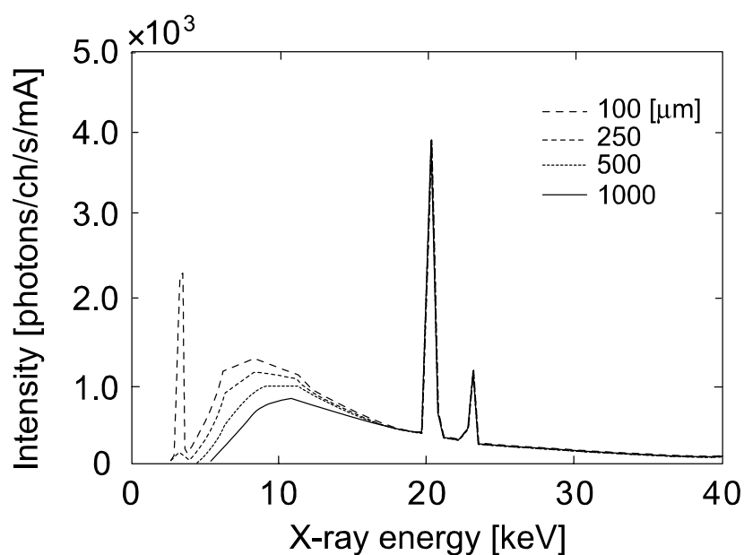
図 3.3.3 培地層を通過して細胞に到達する X 線マイクロビームのエネルギースペクトルの計算結果(培地層の厚みが 100, 250, 500, 1000 μm のときの結果を示した)
