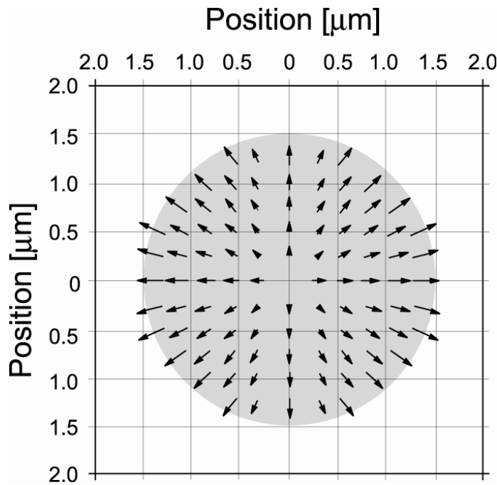
図 A.2.3 レーザー光によって発生する光圧の大きさと方向の関係.
