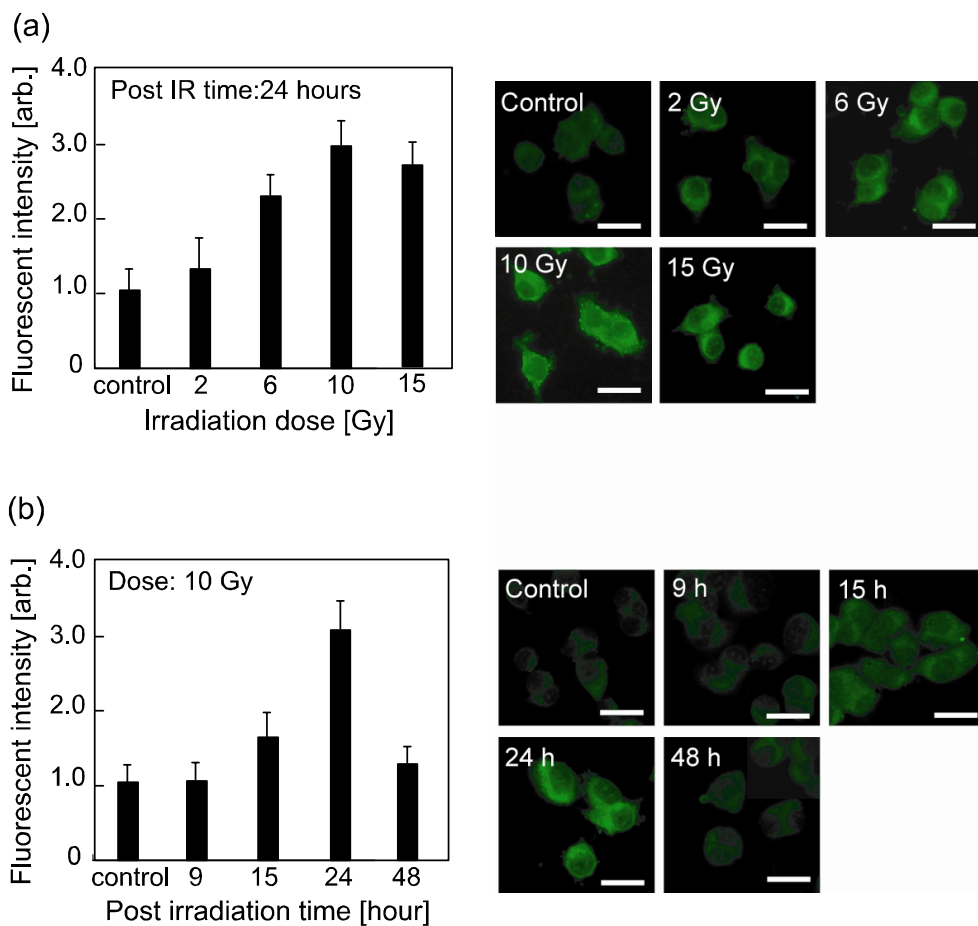
図 5.2.4 (a) \gamma 線照射線量と IL-6 の蛍光量との関係( \gamma 線照射 24 時間後に測定した). (b) \gamma 線照射後の時間と IL-6 の蛍光量との関係( \gamma 線照射量は 10 Gy とした). 誤差棒は標準偏差を, スケールバーは 20 \mu\text{m} を示している.
