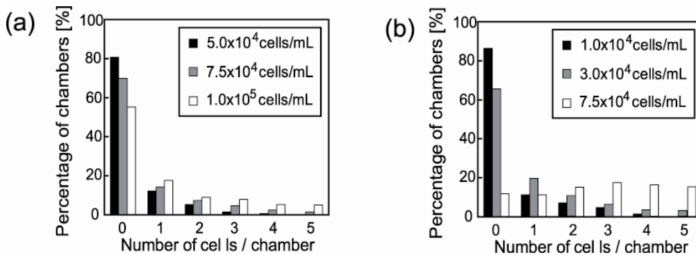
図 4.3.3 (a) 50 \mu\text{m} サイズと(b)100 \mu\text{m} サイズの McAC 上に異なる細胞密度で細胞を蒔種した時の, 各マイクロチャンバーに格納される細胞数とその割合の関係. 測定結果は 3 度の独立した蒔種におけるデータの平均値を示している.
