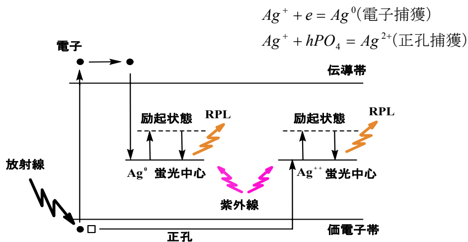
図 2.3.2 RPL ガラス線量計の蛍光発生過程
