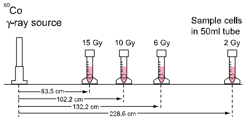
図 5.2.3 \gamma 線照射実験のレイアウト. それぞれの線量に対応した線源からの距離 (2008 年 10 月 14 日時点)を示した.
