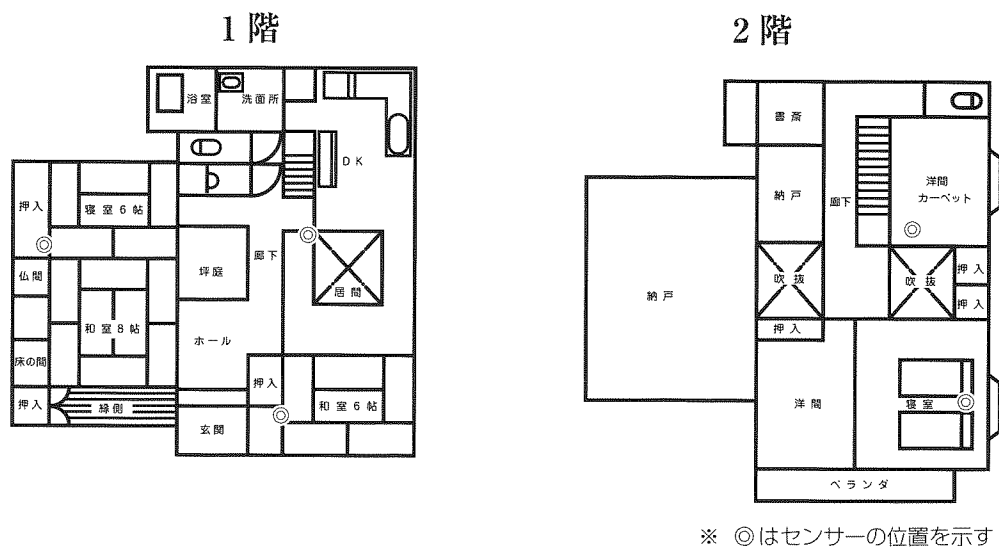
図1. 猪川町住宅見取図
