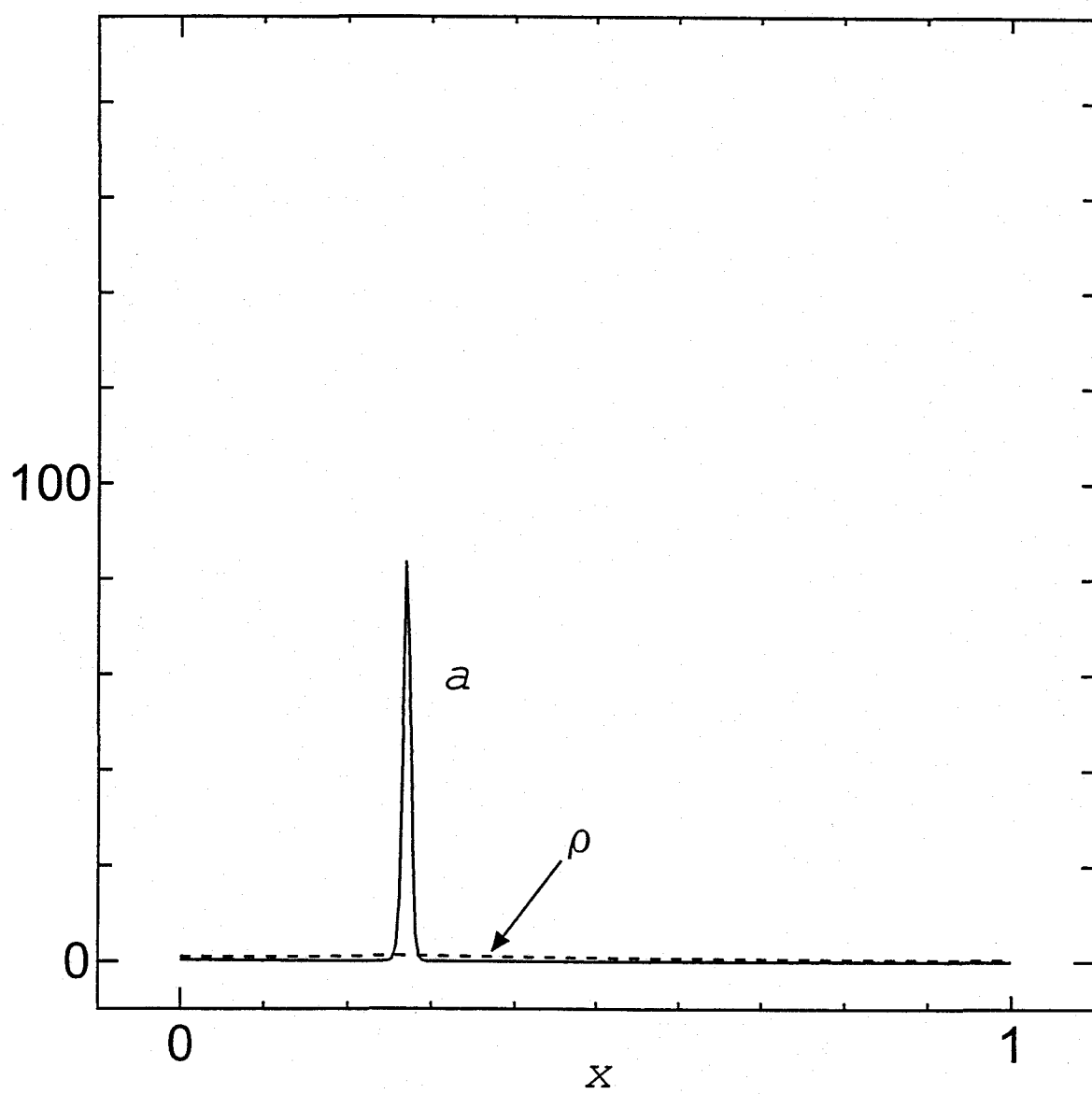
図 6.2 (d) t = 0.1
