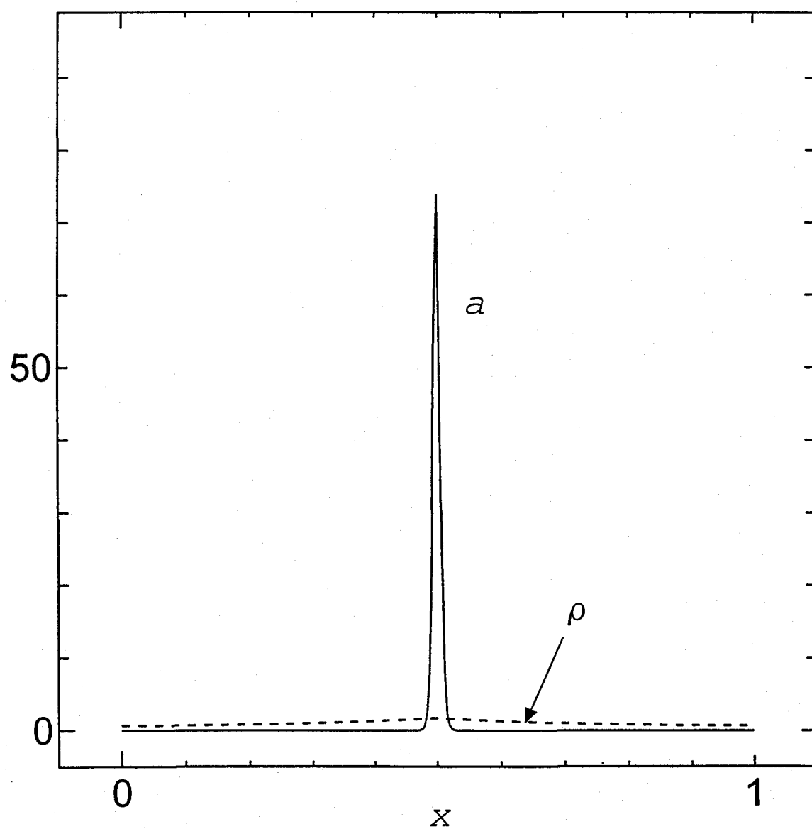
図 6.1 (d) t = 7
