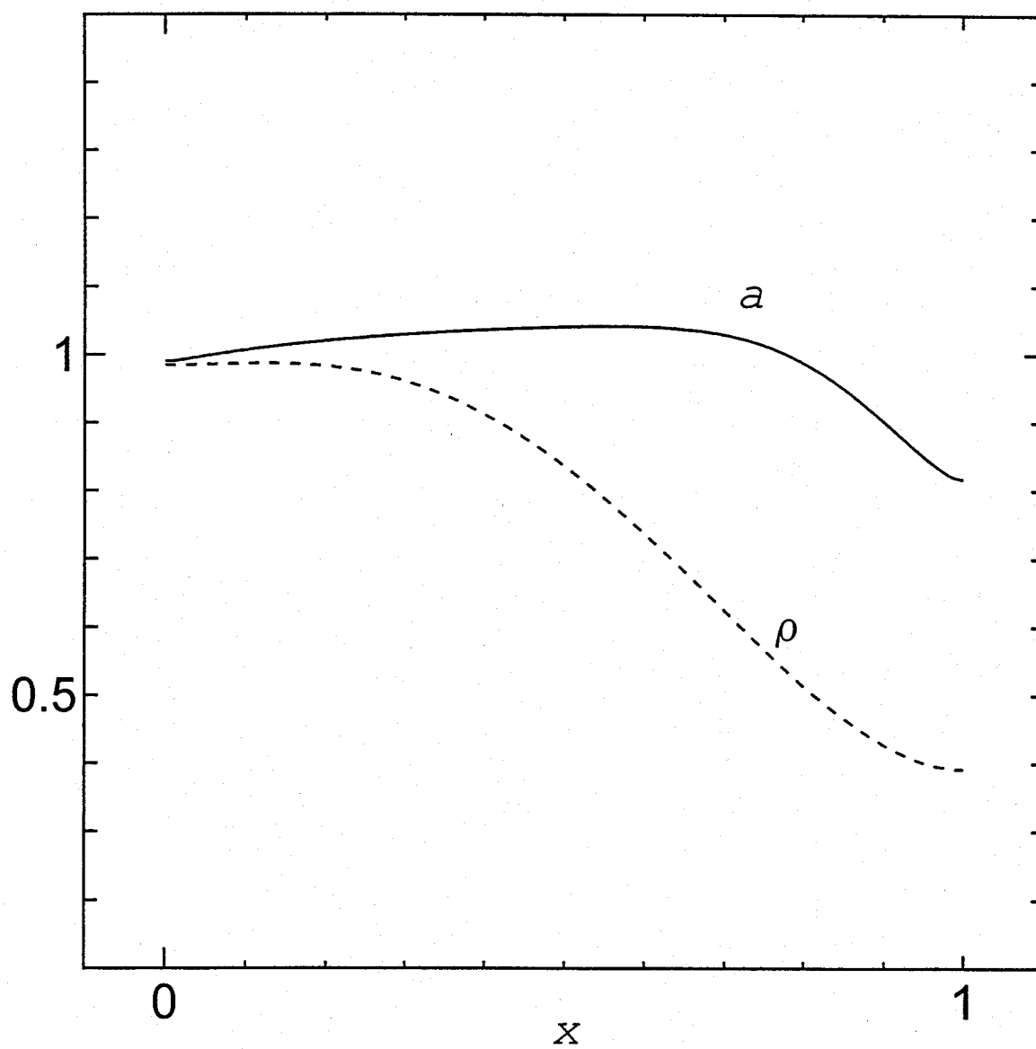
図 6.2 (b) t = 0.001
