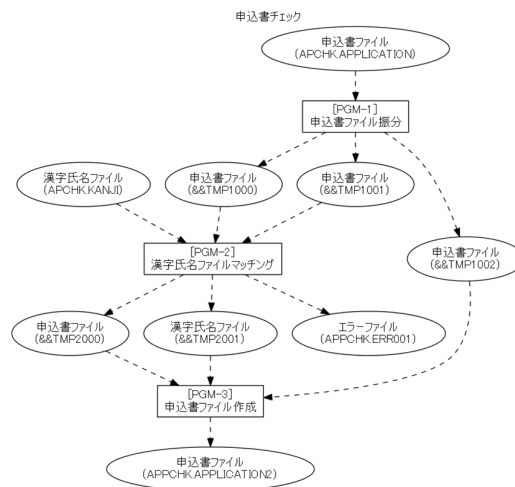
図 3.5 既存手法で作成した申込書チェック機能のデータフロー図
