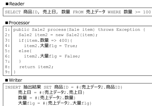
図 4.4 バッチフレームワークによる実装例 (Filter)
