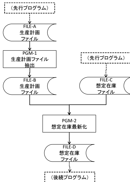
図 3.1 既存手法によるデータフロー図の例
