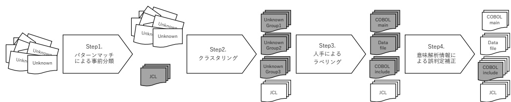
図 2.1 AutoSort の手順
