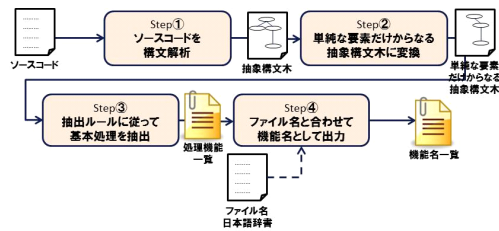
図 3.3 提案手法の概略
