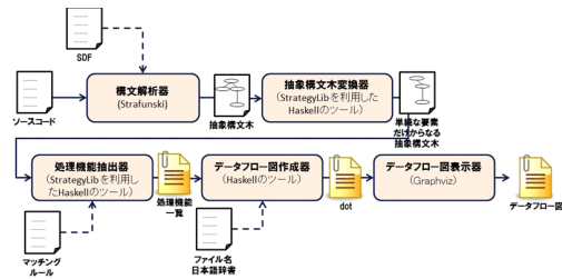
図 3.4 試作した処理機能抽出ツールの概要
