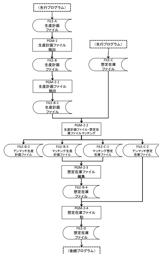
図 3.2 処理機能を抽出したデータフロー図の例
