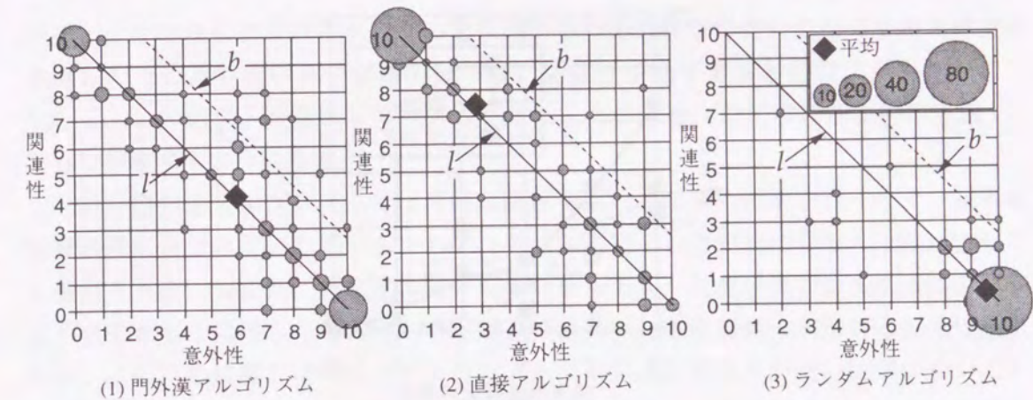
図 2.7: 全評価結果の散布図
