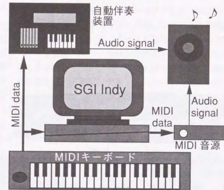
図6.3: 試作器による演奏環境の全体構成
