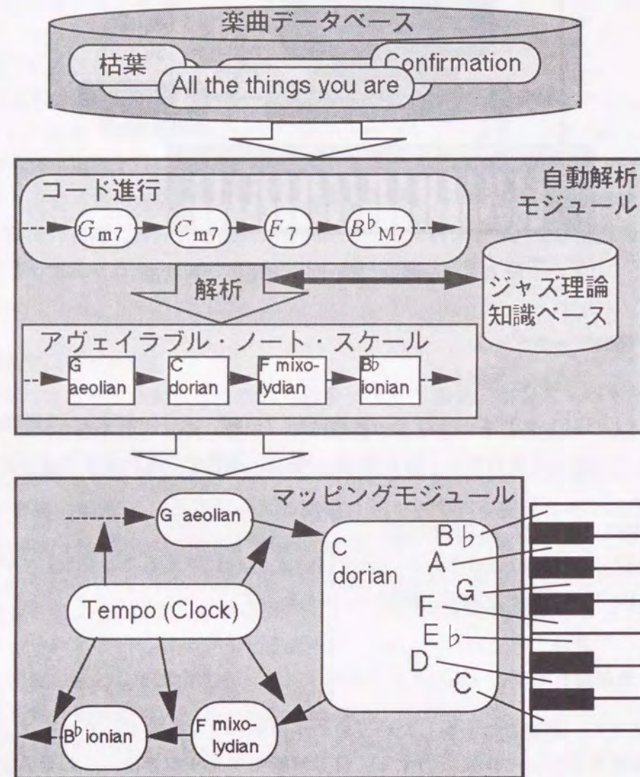
図 6.4: 試作器のソフトウェアモジュール構成
