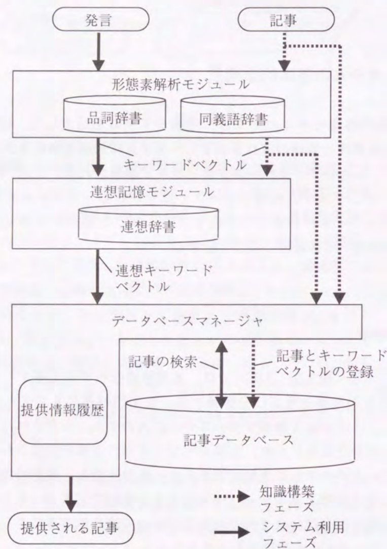
図 2.3: 実験システムのソフトウェア構成と処理の流れ
