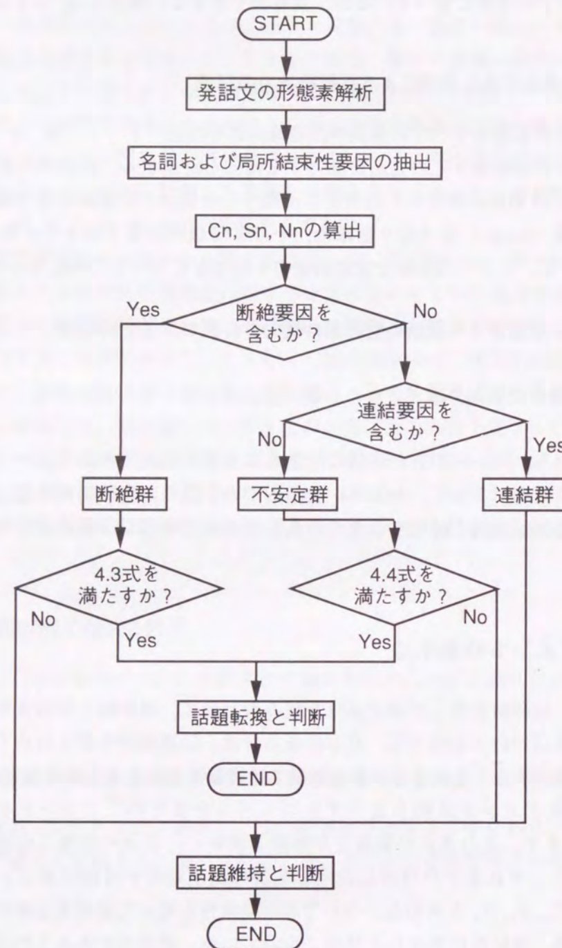
図 4.3: セグメント分割の処理の流れ
