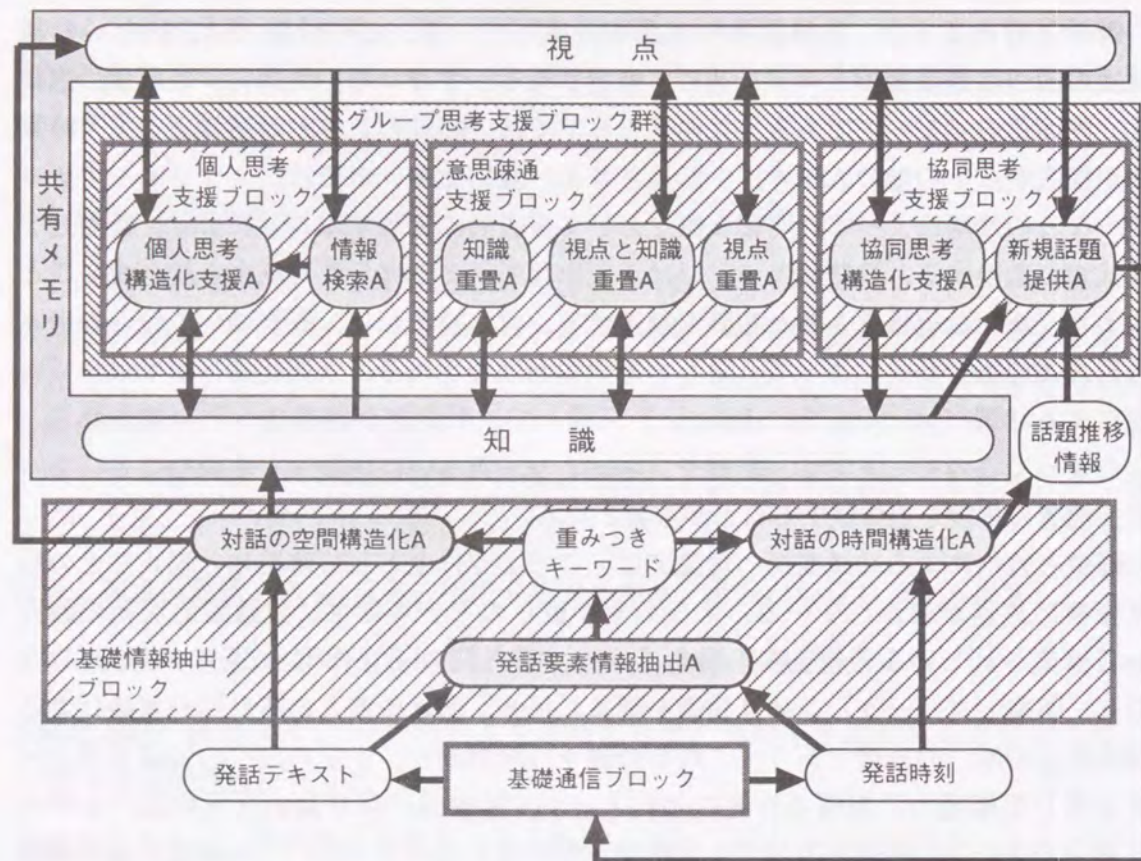
図 5.2: AIDE を構成する機能ブロックとエージェント群
