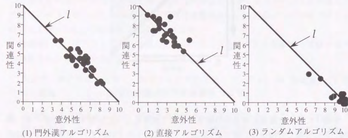
図 2.5: 被験者ごとの評価値の平均の分布
