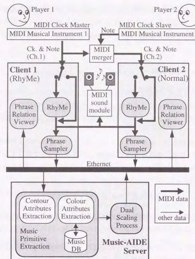
図 7.1: Music-AIDE システム構成図
