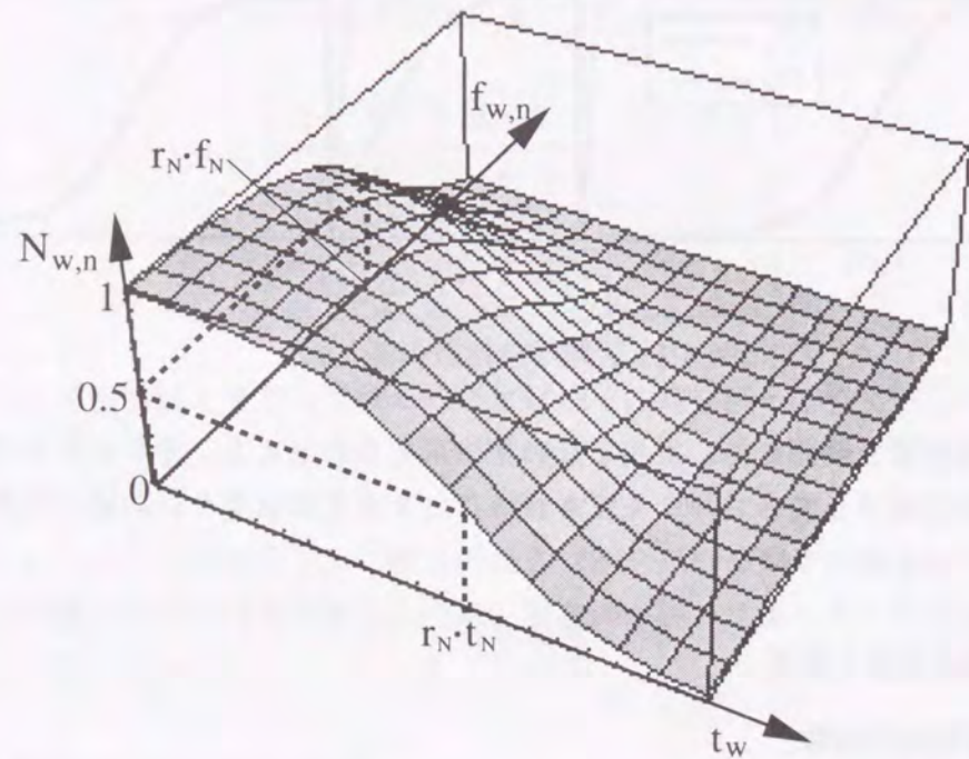
図 4.2: 名詞の話題維持寄与指数の変化の様子
