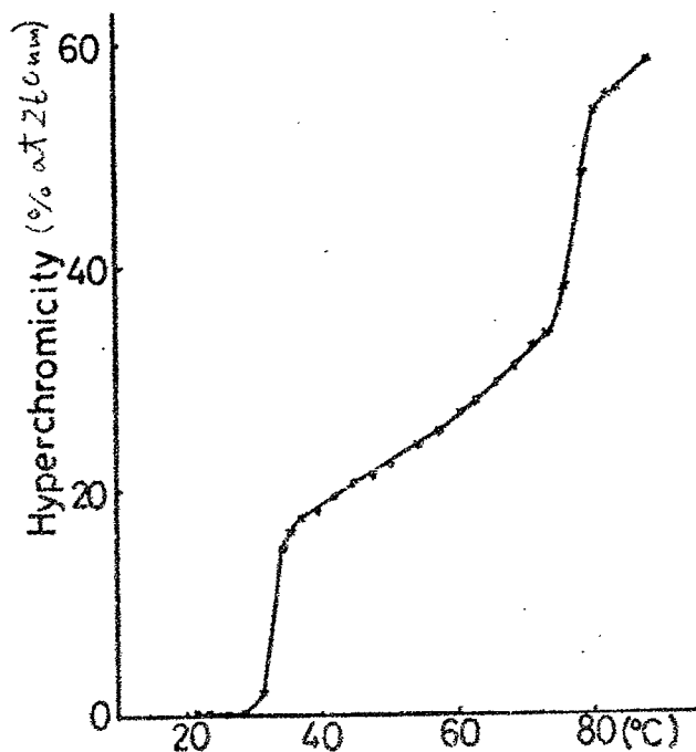
Fig 10(b) poly (Az) の temperature.- absorbance profile (PH 5.0)
