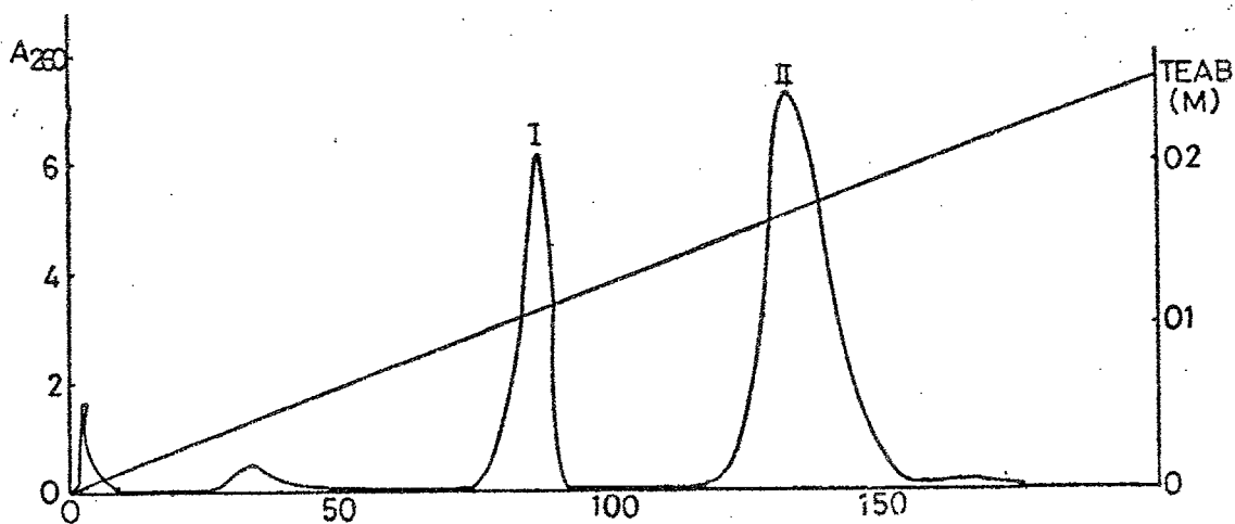
Fig 3 DEAE Sephadex A-25 (bicarbonate) に J3 AzDP の分離
