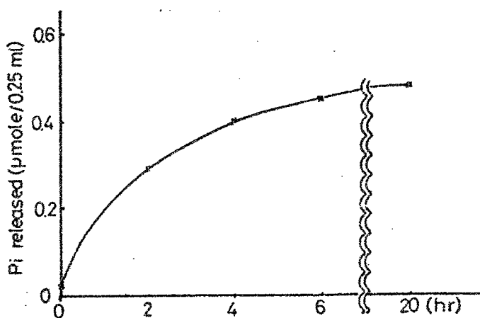
Fig 4 poly(Az) 合成の Time course
