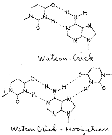
Fig 14: (A)-(U) complexの構造
