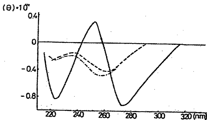
Fig 9-a CD spectra of poly(Aa) taken at 20°(—), 46°(---) and 66°(-.-.-).
