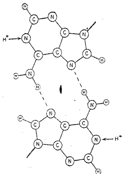
Fig 8 "acid form" の構造
