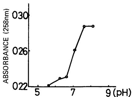
Fig. 4. Acid titration of poly(Aa).
