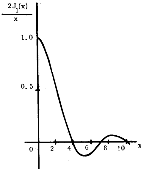
Fig. 3-2 平均化の重み関数 \frac{2J_1(2\pi acA)}{2\pi acA} の一般的形状
