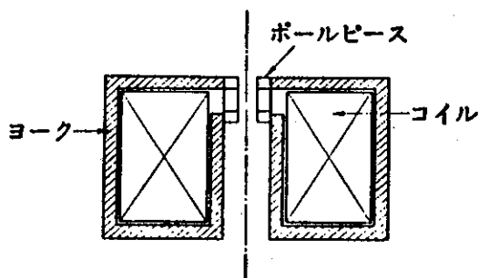
Fig. 1-8 磁界型電子レンズ
