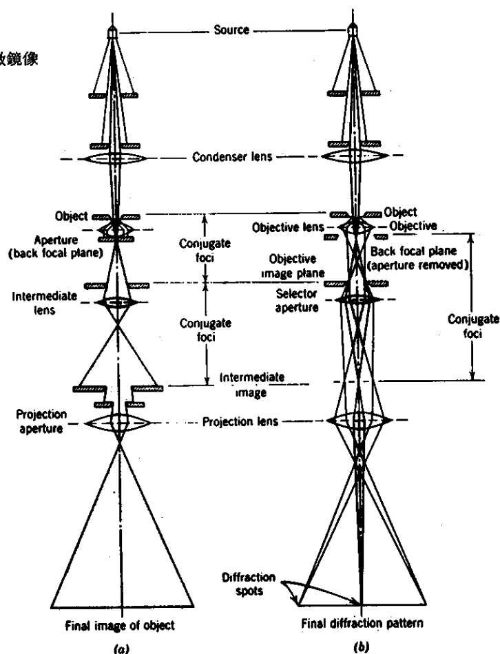
Fig. 1-13 顕微鏡像(a)と制限視野回折像(b)を得る場合の光線図 (from Heidenreich 1964)
