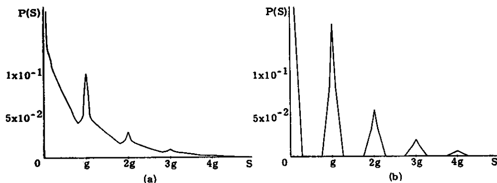
Fig. 4-5 雑音を含む周期物体の処理像のパワースペクトル
