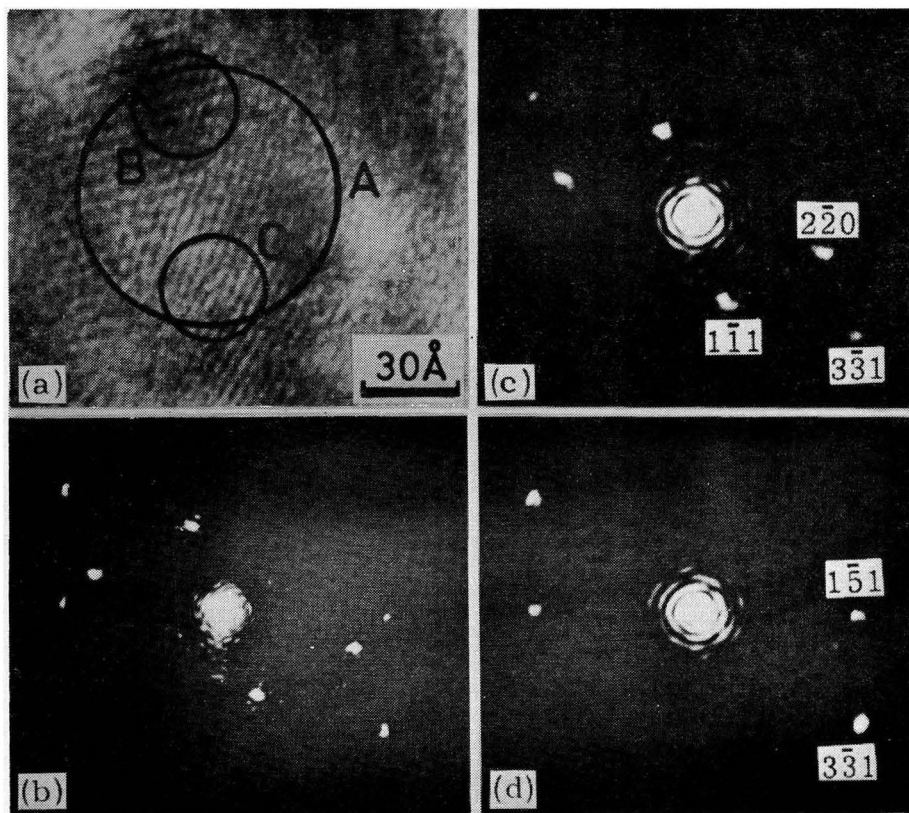
Fig. 2-7 微結晶に含まれる2つの結晶粒の光回折法による識別
