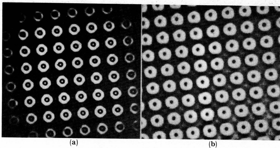
Fig. 3-11 格子像のモデル (Fig. 3-9 (a)) のフィルターグレーティングによる処理 (a) 0.5 g\phi の穴径のフィルターで処理したもの (b) 0.075 g\phi の穴径のフィルターで処理したもの
