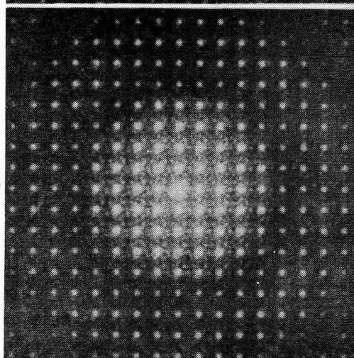
Fig. 3-8 (b) フィルターグレーティングの光回折像 フィルターの穴径は
