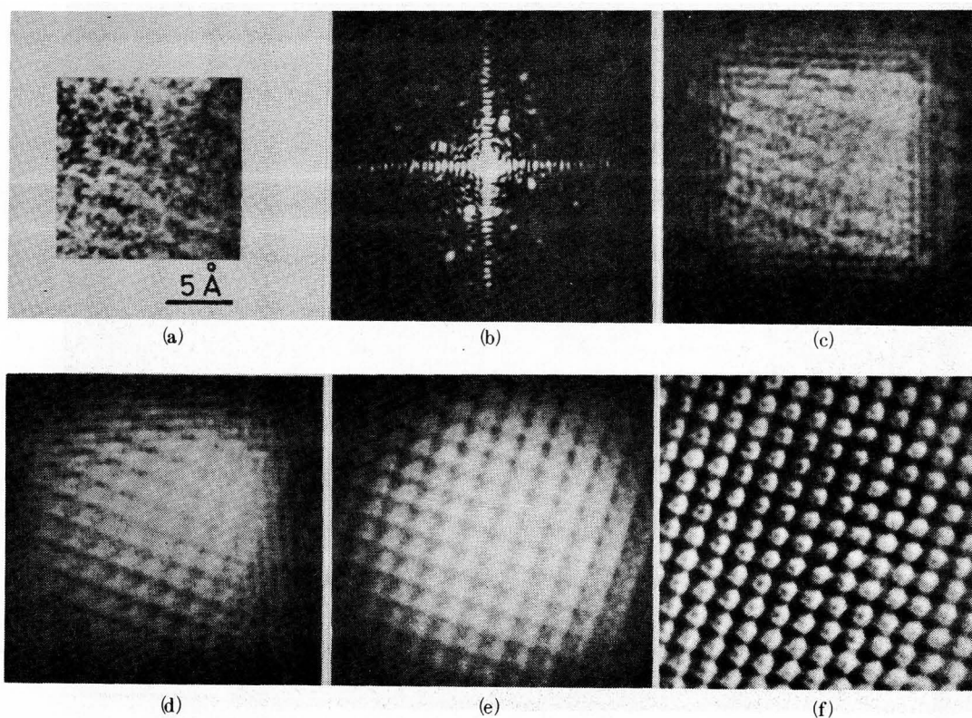
Fig. 3-14 金格子像の処理
