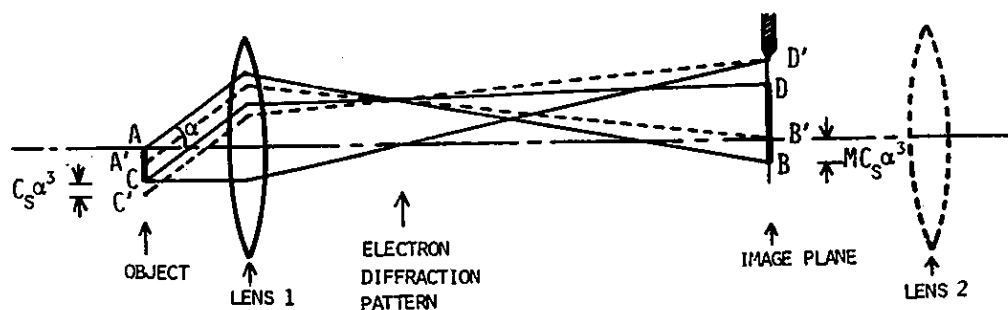
Fig. 1-18 制限視野回折における対物レンズ (LENS I) の球面収差のためのビームのまわり込みと視野の関係
