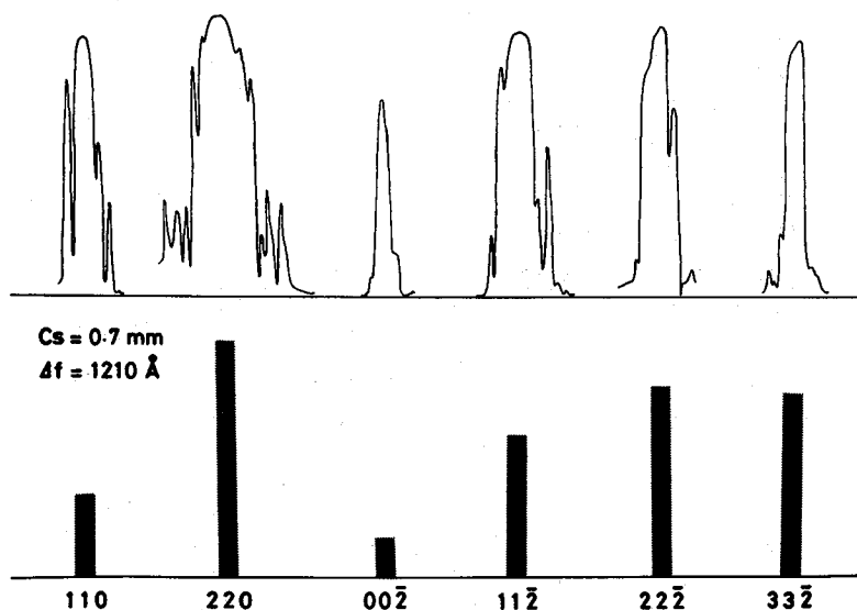
Fig. 2-11 ラボラドライト長石の格子像からの光回折強度 実験値と計算値との比較(1)
