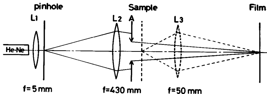
Fig. 2-2 光回折光学系
