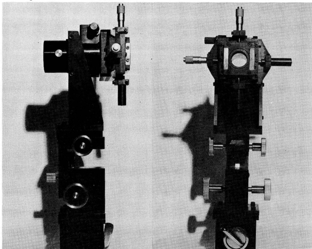
Fig. 3-6 フィルターホルダー
