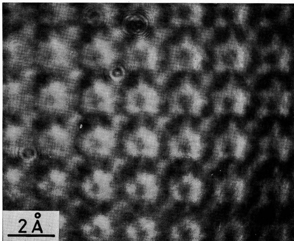
Fig. 3-17 金の処理像
