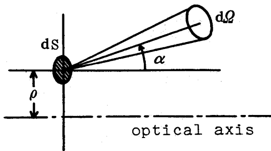
Fig. 1-2 座 標 系
