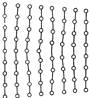
Fig. 2-17 格子湾曲
