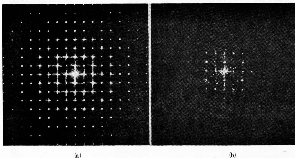
Fig. 3-18 格子像のモデルの光回折像
