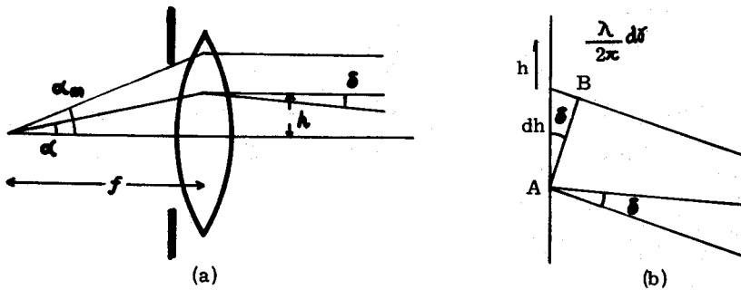
Fig. 1-15 収差による位相のおくれ (本文参照)
