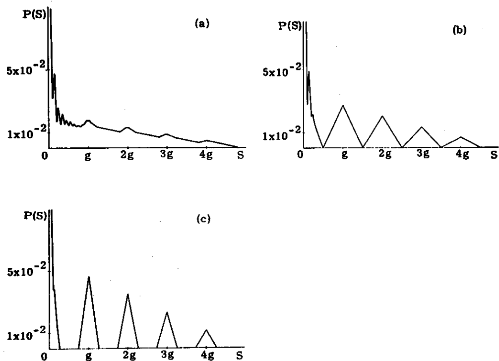
Fig. 4-3 疑似格子像のパワースペクトルの計算
