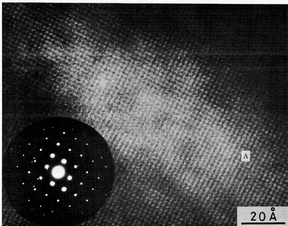
Fig. 3-13 57波を用いて結像された金(001)面の結晶格子像 Aの部分の処理がFig. 3-14に示される。
