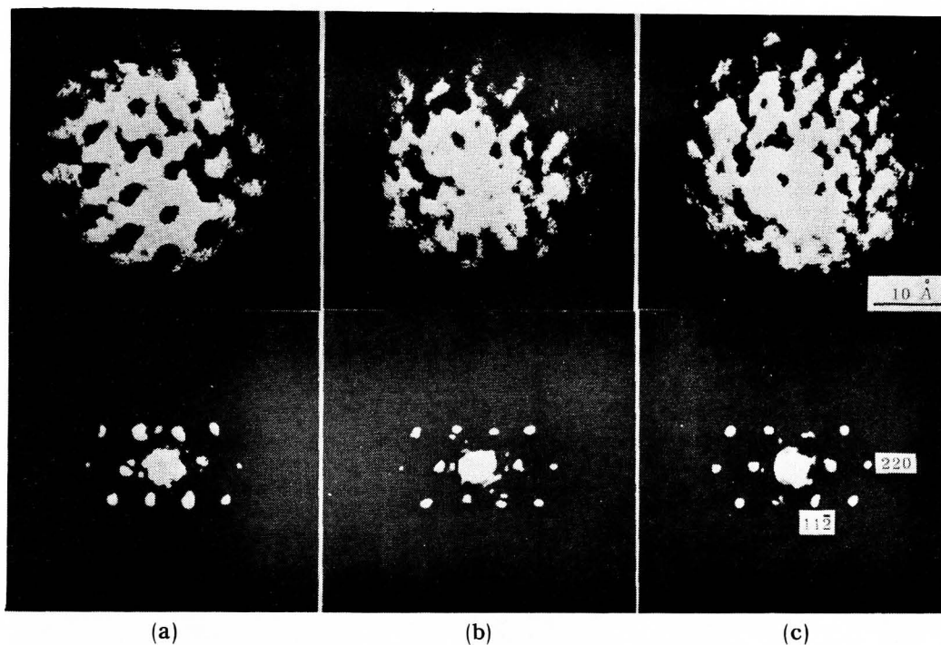
Fig. 2-14 転位の周りの歪んだ結晶格子とその光回折像
