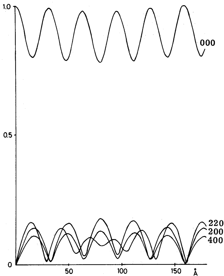
Fig. 3-20 動力学的に計算された金結晶からの回折波の振巾の厚さ依存性 (電子線は \langle 001 \rangle 軸と平行な入射を仮定している。)
