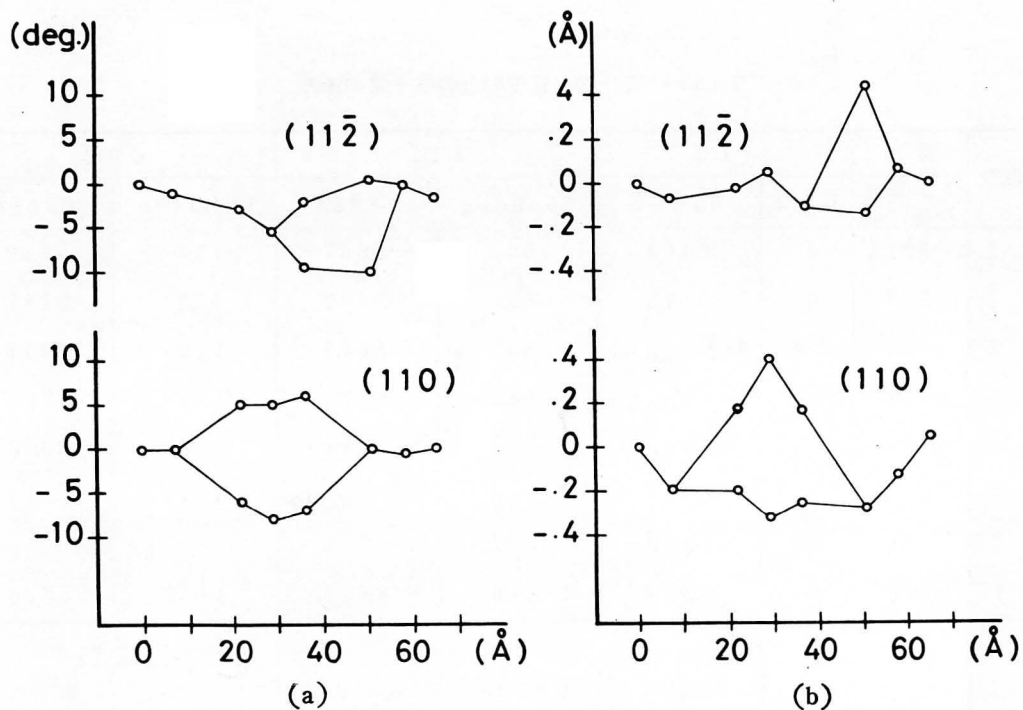
Fig. 2-15 転位付近の像からの光回折斑点の振舞い (a) 面間角の変化 (b) 面間隔の変化
