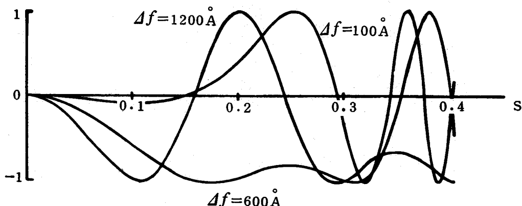
Fig. 1-16 弱い位相物体に対するコントラスト伝達関数
