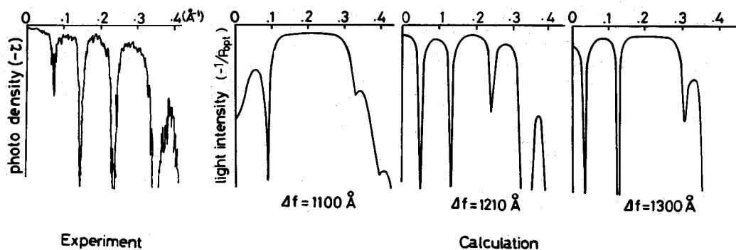
Fig. 2-10 ユニットセルからの光回折強度実験値と計算値との比較
