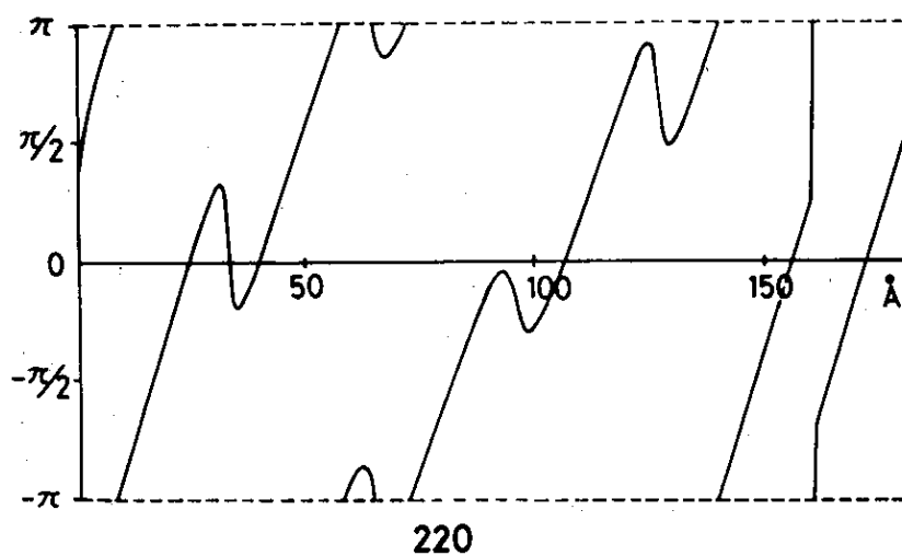
Fig. 3-21 動力学的に計算された金結晶からの回折波の位相の 厚さ依存性
