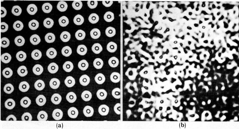
Fig. 3-19 円形絞りによる格子像の処理
