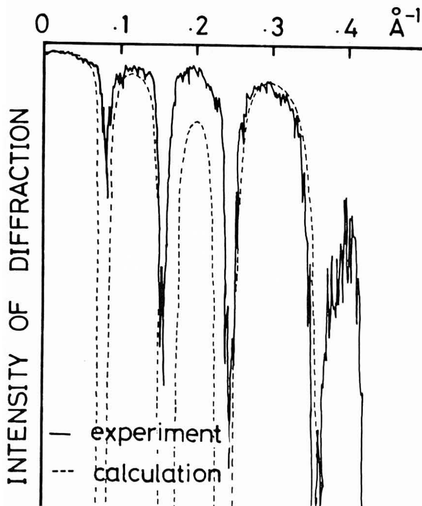
Fig. 2-9 ユニットセルの光回折強度 ( -\tau ) と結晶構造因子 -|F(s)|^2 との比較
