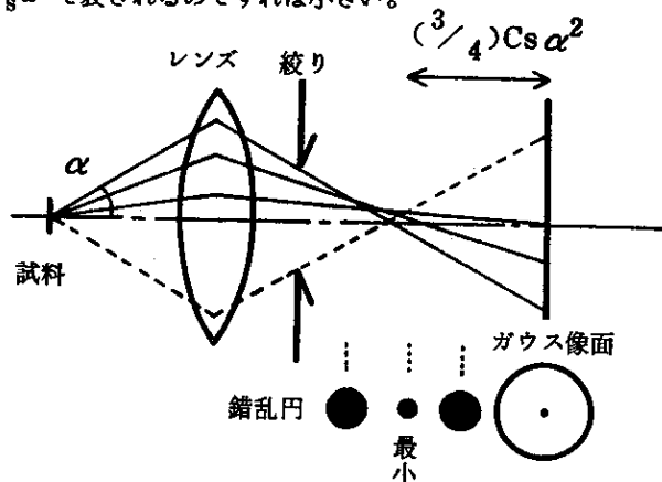
Fig. 2-1 球面収差による錯乱円は \Delta f = (8/4)C_s \alpha_m^2 のとき半径 (1/4)C_s \alpha_m^3 で最小となる。
