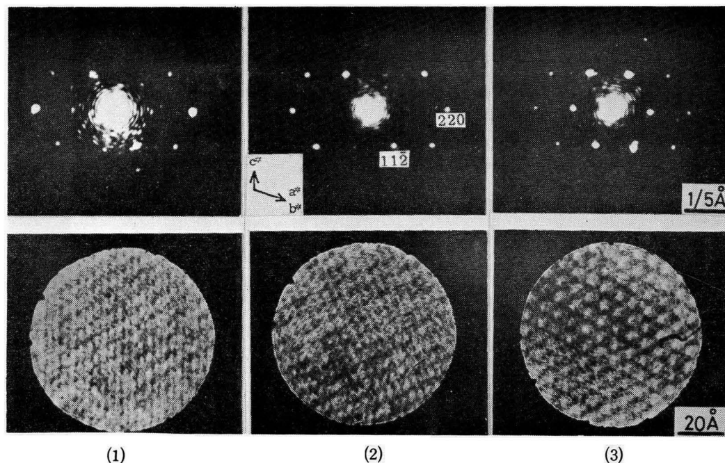
Fig. 2-4 ラボラドライト長石の格子像からの微小領域制限視野回折 (1)~(3)がそれぞれ Fig. 2-3 の円 1~3 内の回折像と拡大像 に相当する
