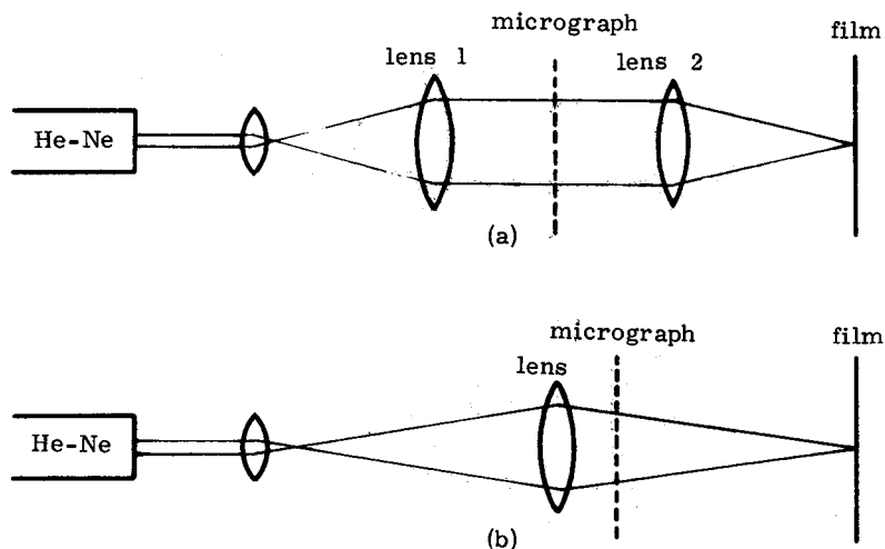
Fig. 1-21 光回折光学系
