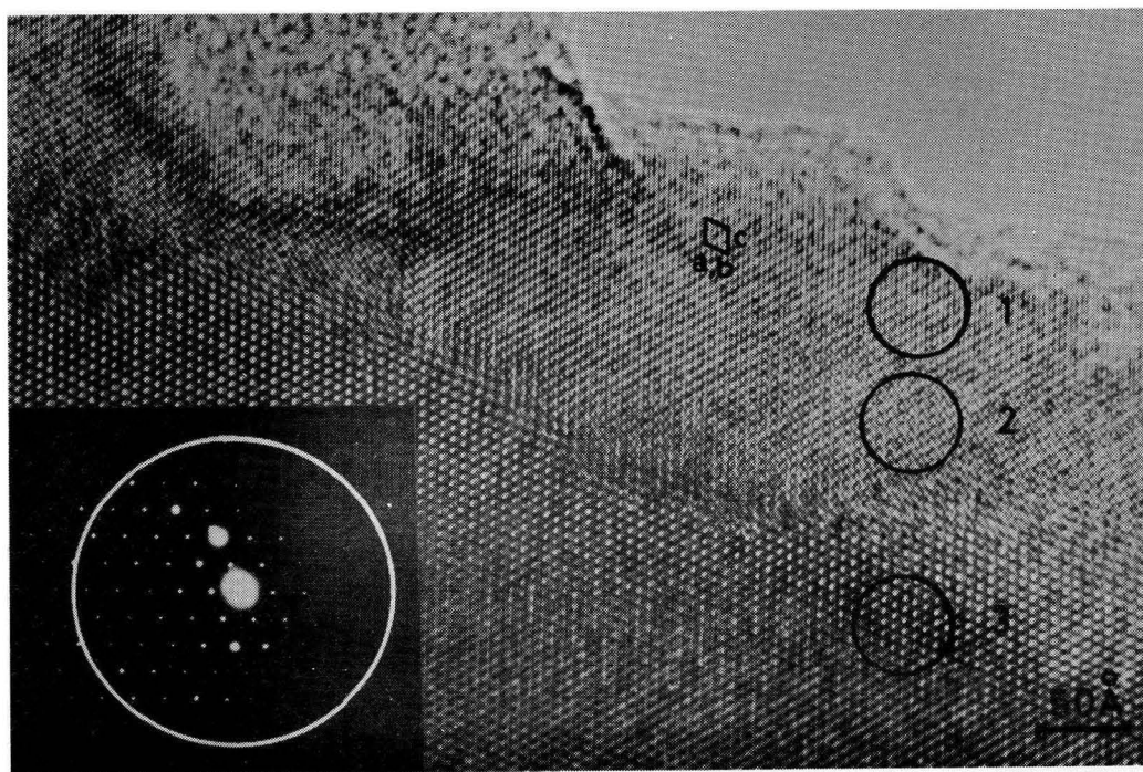
Fig. 2-3 ラボラドライト長石の格子像
