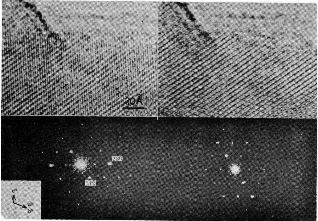
Fig. 2-5 異なる焦点外れ量で撮影された同一視野の格子像とその光回折
