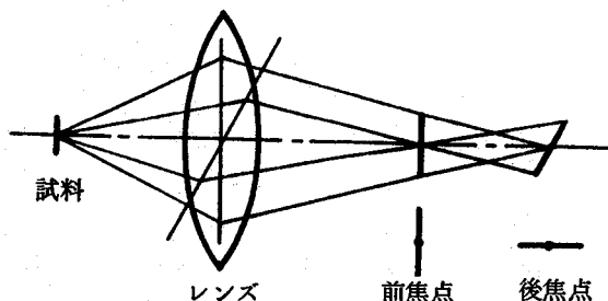
Fig. 1-12 非点収差 (非対称収差)
