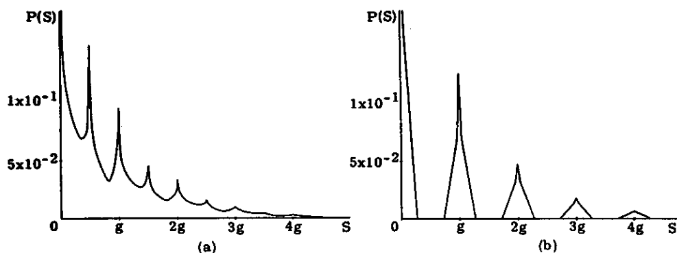
Fig. 4-6 雑音を含む周期物体の処理像のパワースペクトル
