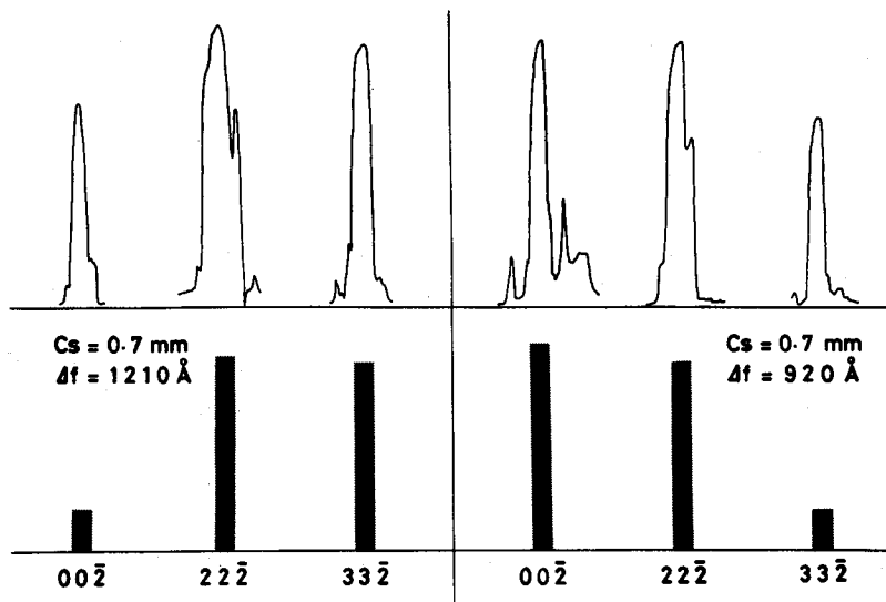
Fig. 2-12 ラボラドライト長石の格子像からの光回折強度 実験値と計算値との比較(2)
