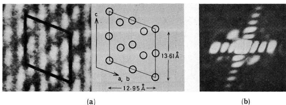
Fig. 2-8 ユニットセルからの回折像
