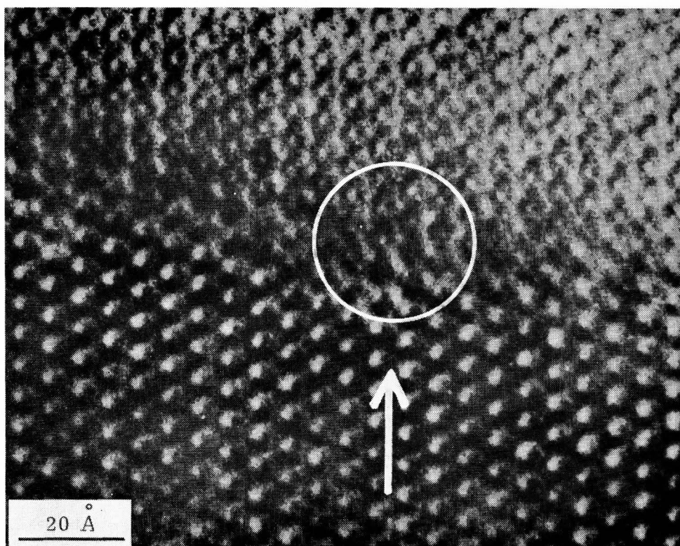
Fig. 2-13 転位を含むラポラドライト格子像 矢印の向きに丸印の大きさの視野を走査して光回折を行う。
