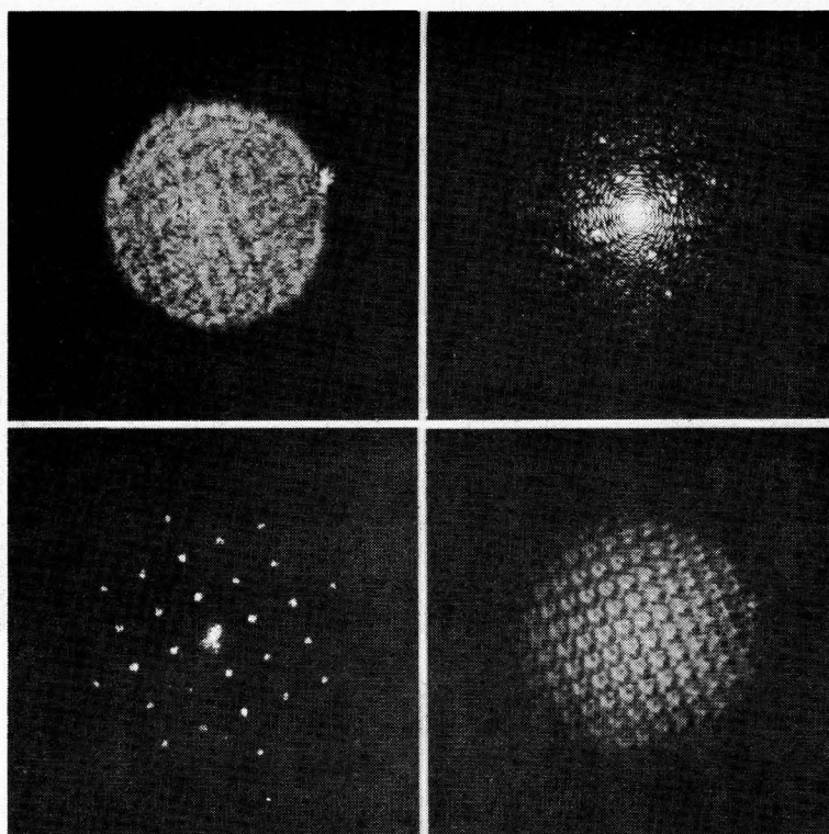
Fig. 3-16 Au(001)格子像の色収差補正 (a) 被処理像 (c) フィルター挿入後の回折像 (b) (a)の光回折像 (d) 処理像
