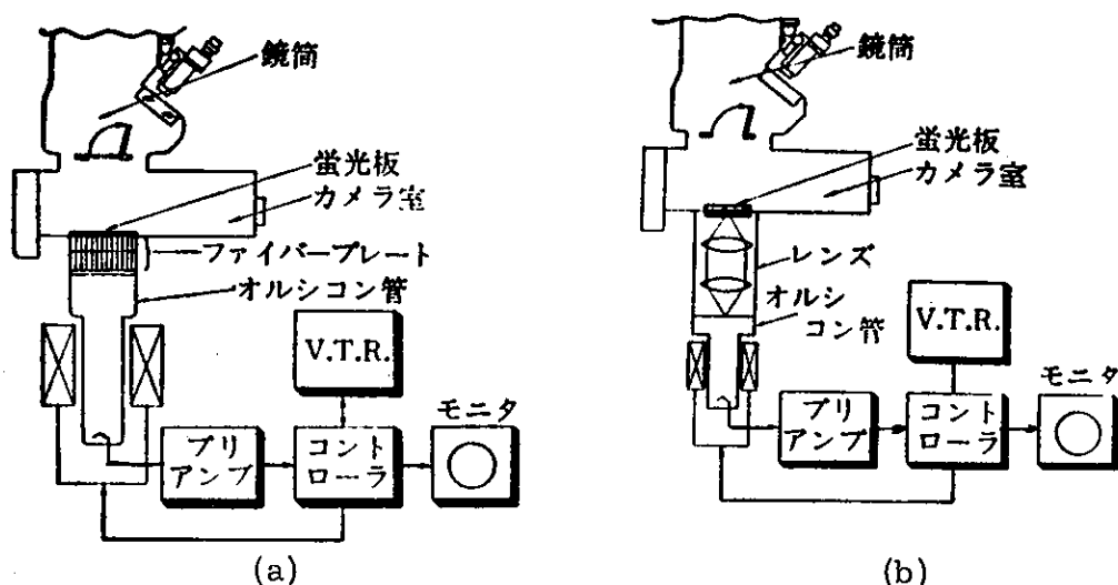
Fig. 1-7 間接方式のTV装置
