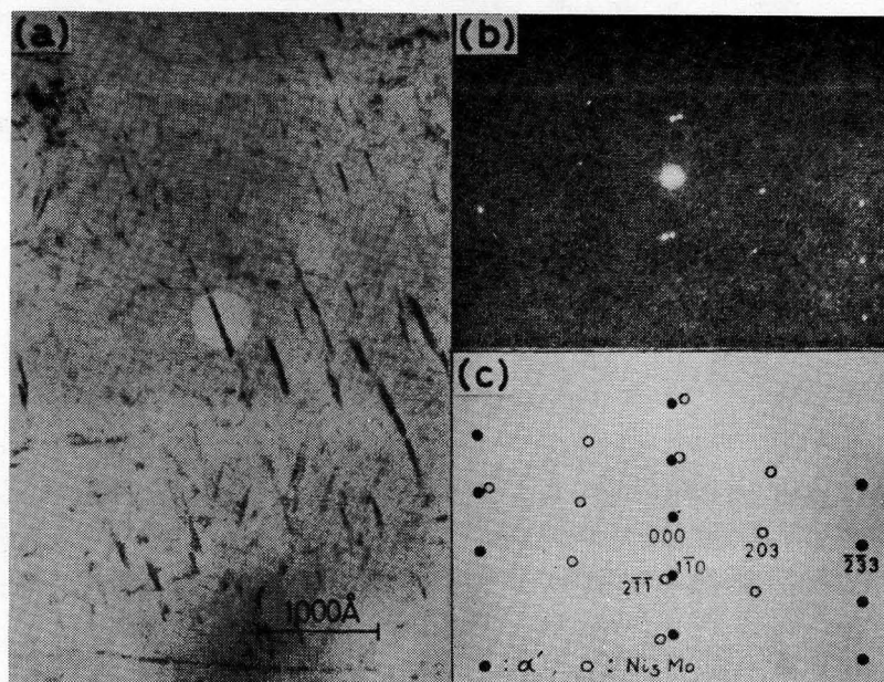
Fig. 1-19 650kV超高電圧電子顕微鏡による制限視野回折
