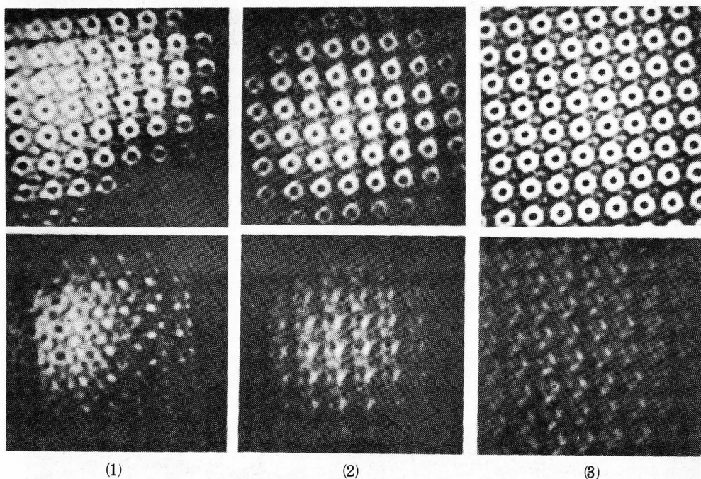
Fig. 3-12 モデル像の処理
