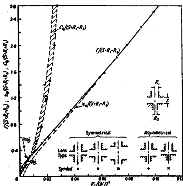
Fig. 1 - 10 磁界型レンズの焦点距離 f 、無限遠 へ像を作るための試料位置 Z_0 、球 面収差係数 C_s と起磁力との関係 (from Liebmann 1955 b)
