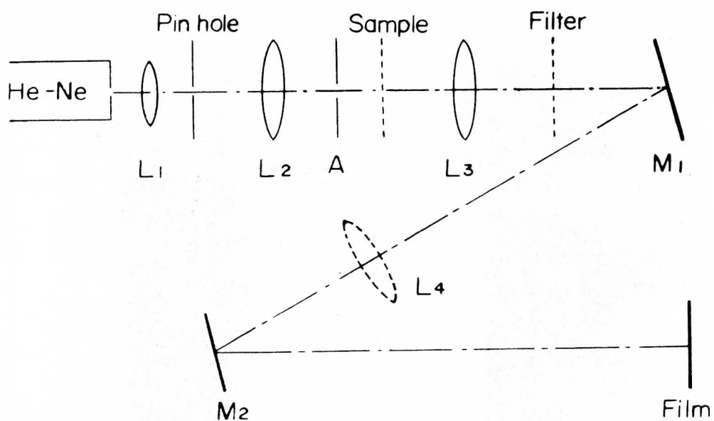
Fig. 3-4 処理光学系の光路図
