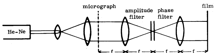
Fig. 1-22 インバース・フィルターリング光学系
