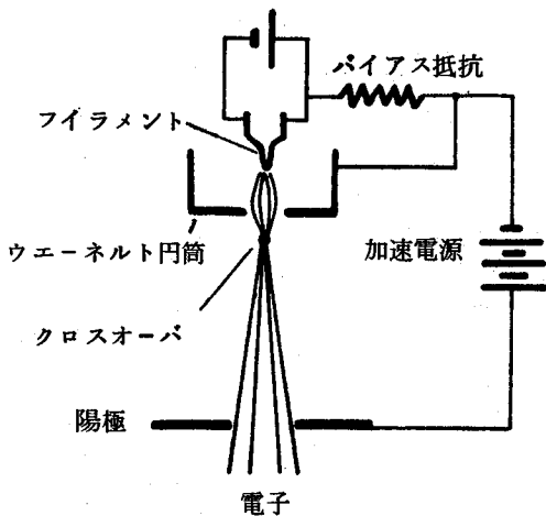
Fig. 1-3 電子銃
