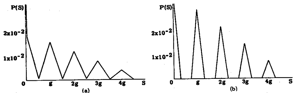
Fig. 4-4 視野を 100/g に広げた場合の疑似格子像のパワースペクトル
