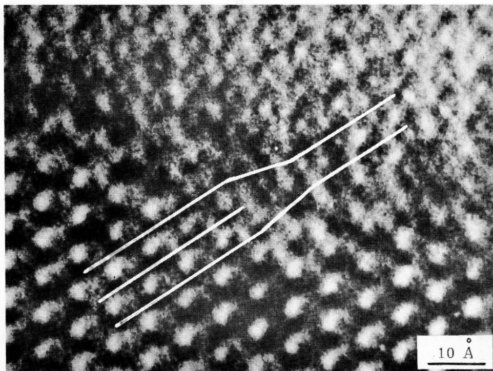
Fig. 2-16 転位 の 方 向
