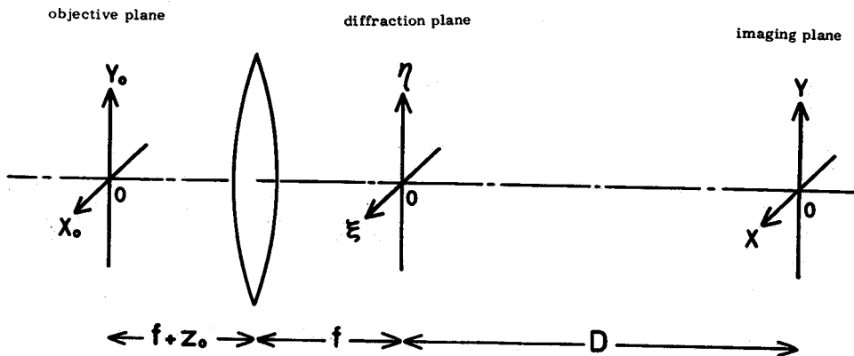
Fig. 3-1 座標系
