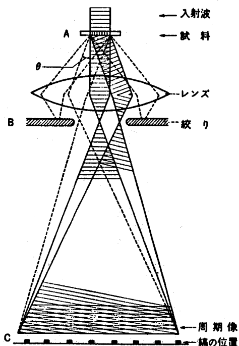
Fig. 1-14 結晶格子像の撮影
