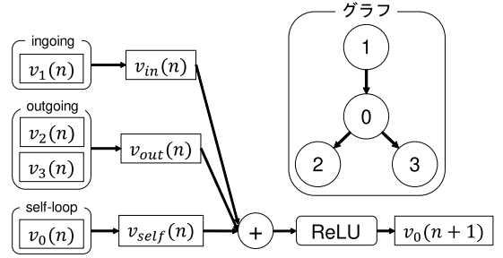
図3 GCN の畳み込み層の例
