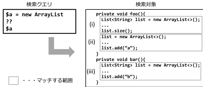
図2 “??” がマッチする範囲の例. (i), (ii), (iii) の3つのコード片にマッチする.
