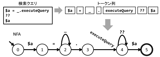
図 3 検索クエリからの非決定性有限オートマトンの構築
