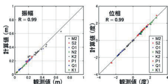
図3：主要8分潮の再現性
