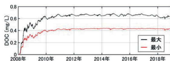
図6：紀伊水道の外洋起源DOC濃度の変動
