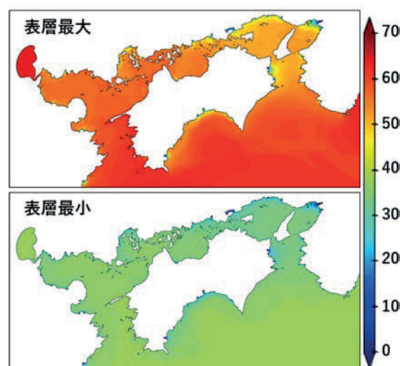
図5：外洋起源DOC (mol/L)の表層分布
