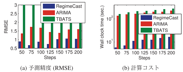
図 11 モーションイベントストリーム (exercise) に対する l_s ステップ先の (a) 予測精度と (b) 計算コストの比較
