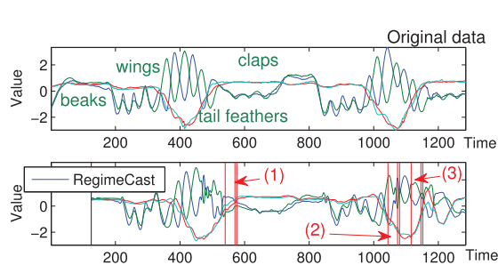
(a) オリジナルデータ (上段) と REGIMECAST の予測結果 (下段)
