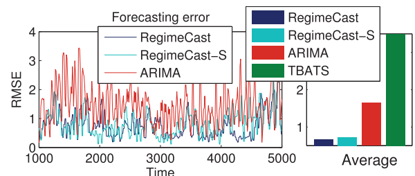
(a) 各時刻における予測値のエラー値 (左) と平均値 (右)
