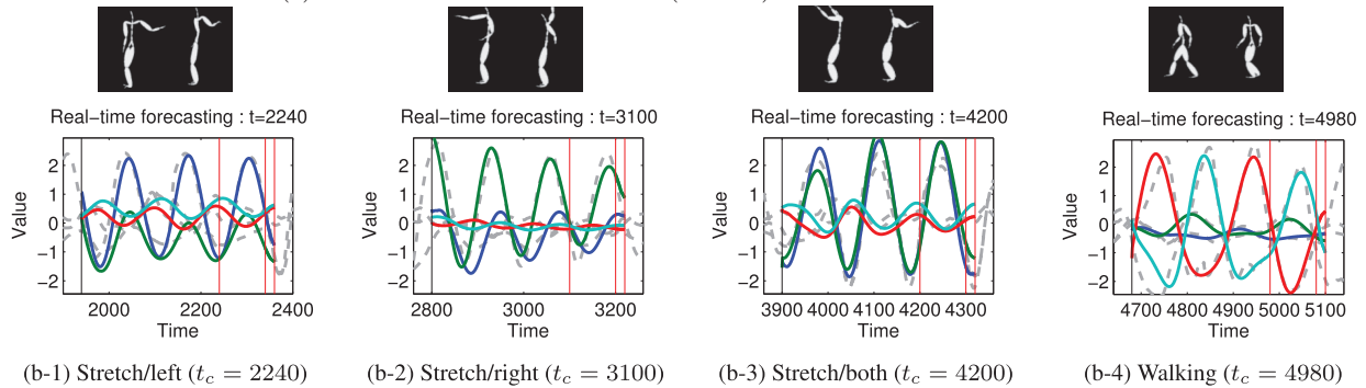
図 5 モーションストリーム (exercise) に対する REGIMECAST の予測結果の様子 ( c^{(1,2)} = 27, 14 )
