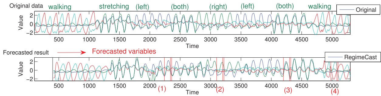
(a) オリジナルストリーム (上段) と (100:120)-ステップ先の予測結果 (下段)
