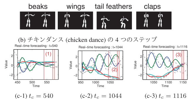
図 6 モーションストリーム (chicken dance) に対する REGIMECAST の予測結果の様子 ( c^{(1,2)} = 5, 9 )
