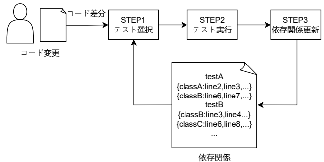
図 1 提案手法全体図
