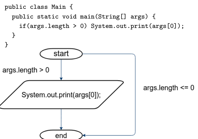
図 1 制御フローグラフの例
