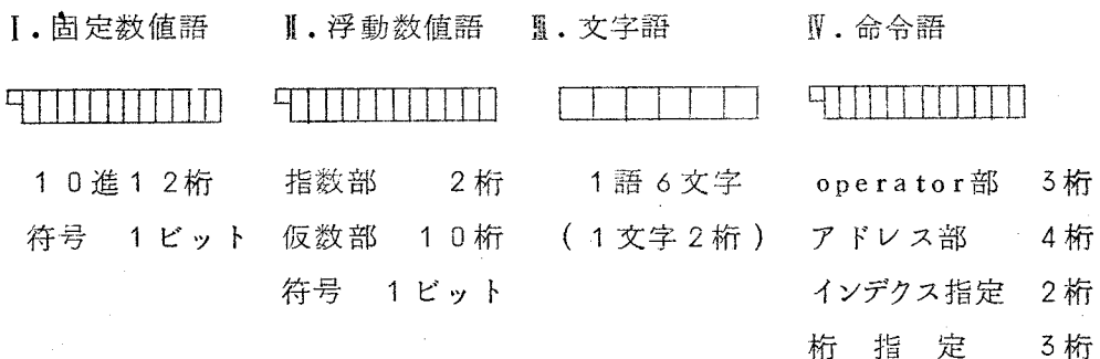
図 6.1 NEAC 2206 の命令
