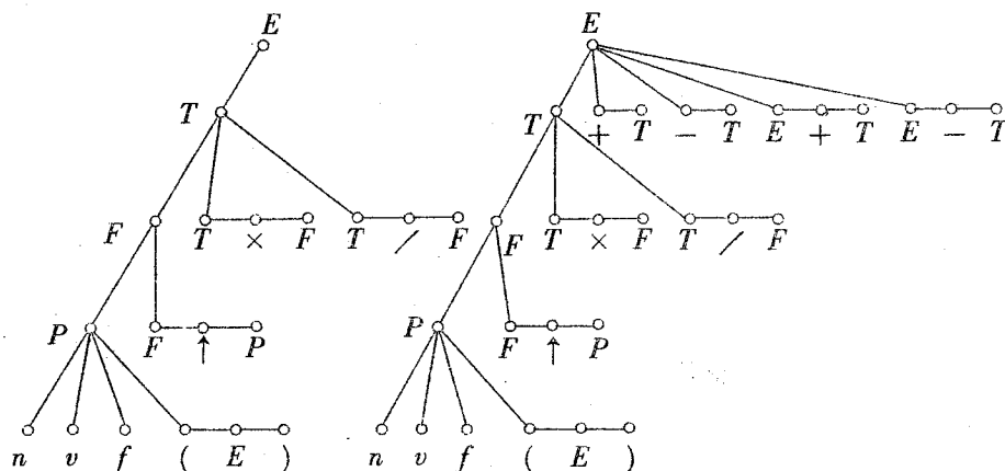
図 4 . 8 II c) の型の書換規則の付加
