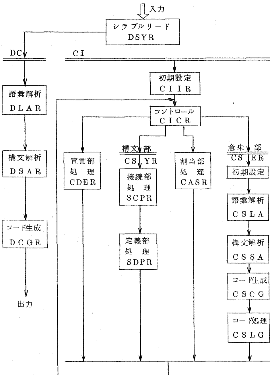
図 5 . 2 DCS 処理フロー
