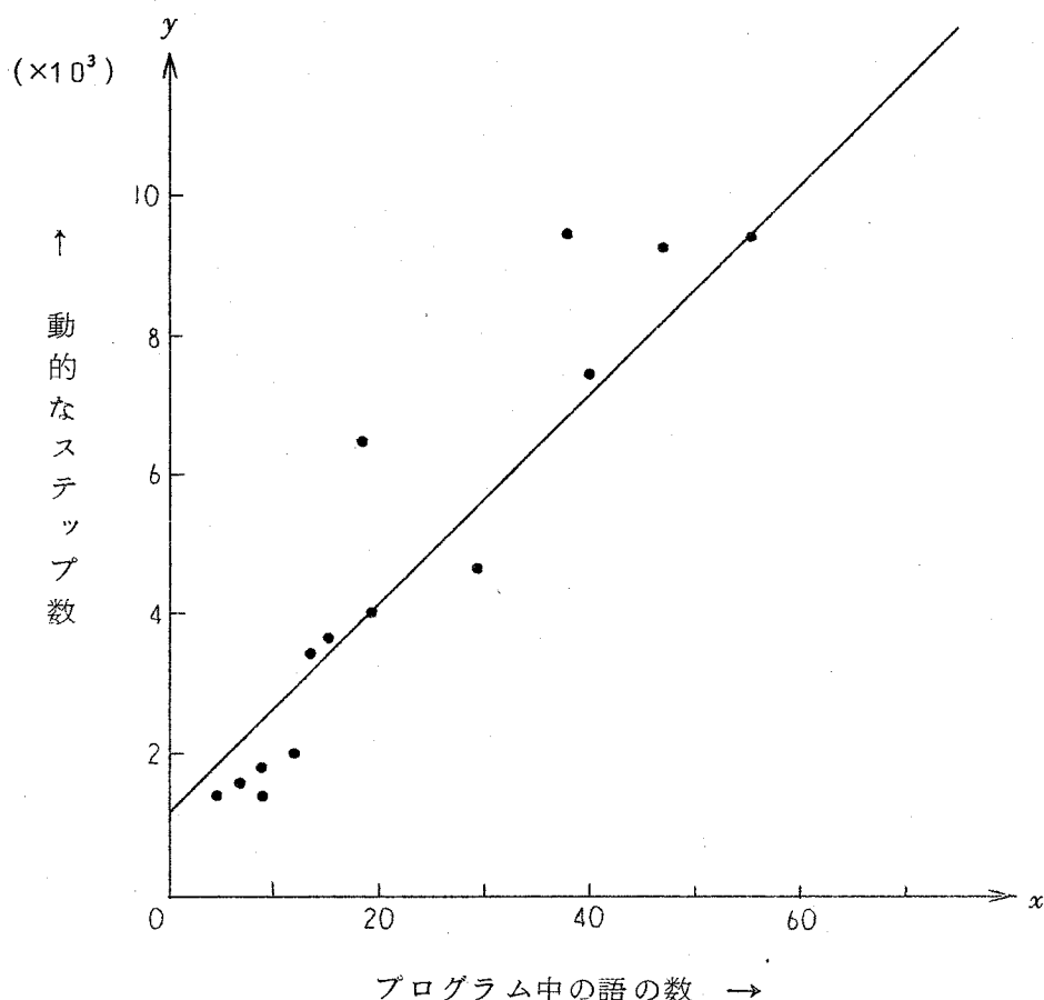
図 6.2 DC における入力語数と動的なステップ数の関係
