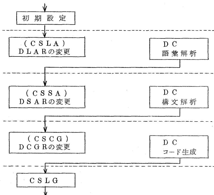
図5.7 CIの意味部処理ルーチン
