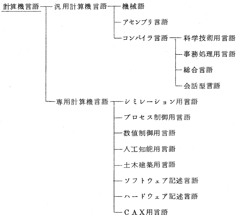
図 1 . 1 計算機言語の種類
