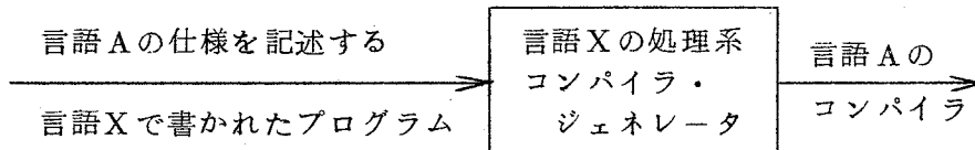
図 2.2 コンパイラ・ジェネレータ
