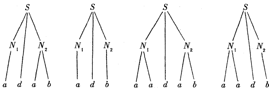
図 4.4 式 (4.4) の L(G) に対する導出樹
