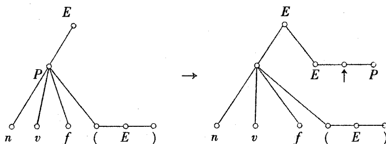
図 4 . 7 II a) 型の書換規則の付加
