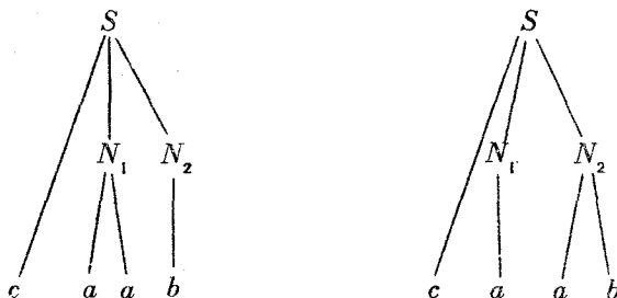
図 4.5 caab に対する二つの導出樹
