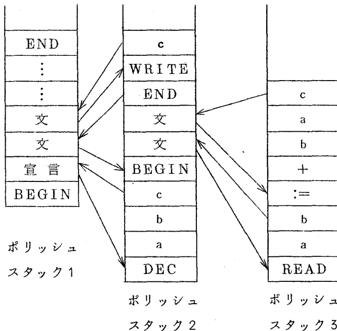
図 5. 3 ストリーム・ポリッシュデータの例
