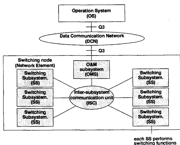
図 50 システム構成例
