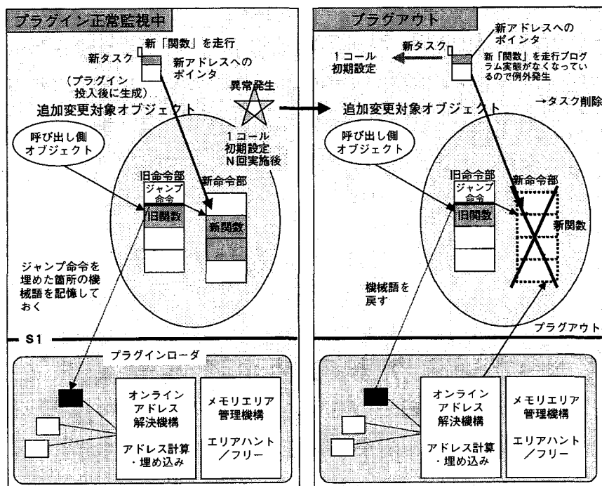
図 30 プラグアウト機構
