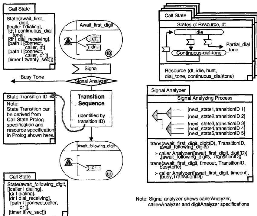
図 72 SDL/PE と実行可能な宣言の仕様記述例
