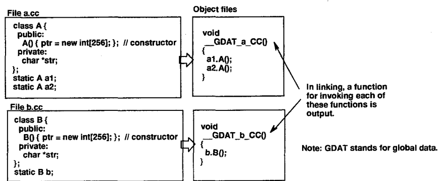
図 28 大域オブジェクトのコンストラクタ起動方式
