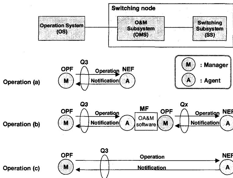
図 62 マネージャとエージェントとの関係
