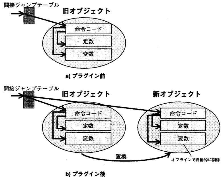
図 21 新オブジェクト追加時の手法（間接ジャンプ方式）
