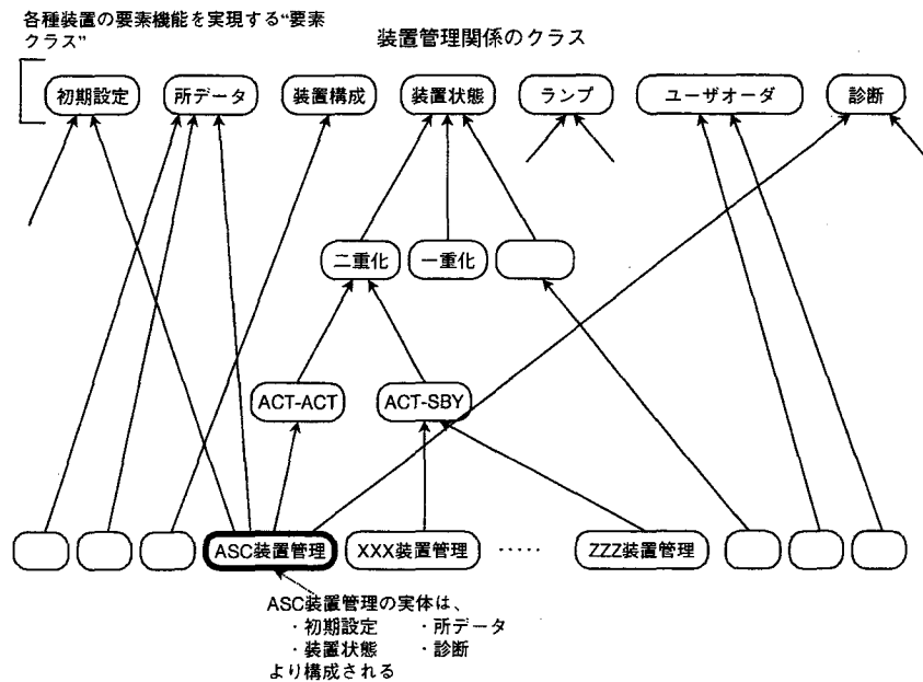
図 14 装置管理クラスの継承関係
