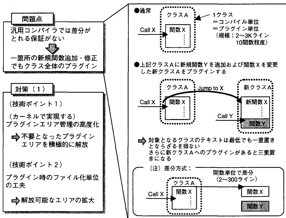
図 39 メモリ使用効率向上対策の必要性
