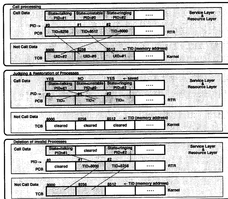
図 58 分散環境での呼救済手法
