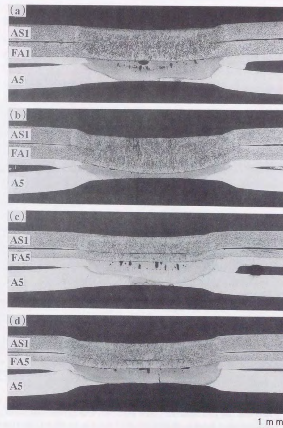
Fig. 6.42 Macrostructures of galvanized steel-aluminum clad steel-aluminum (AS1-FA1-A5, AS1-FA5-A5) spot weld joints: (a) AS1-FA1-A5 11.1kA-0.2s, (b) AS1-FA1-A5 13.9kA-0.2s, (c) AS1-FA5-A5 11.0kA-0.2s, (d) AS1-FA5-A5 14.1kA-0.2s.
