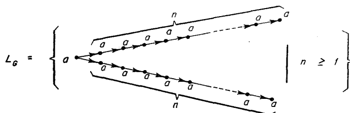
図 2. このウェーブは ncfw L ではない。
