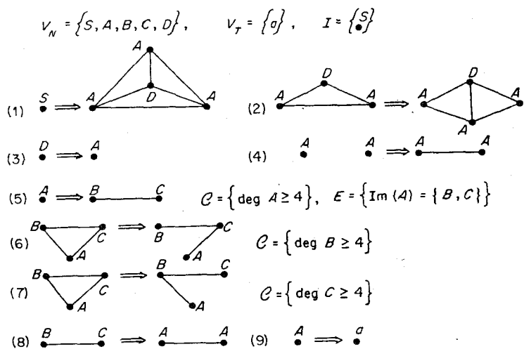
図 14. この \text{anmc swg} はすべての 3-コネクティッドグラフを生成する。
