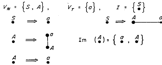
図 7. この \text{anlwg} はすべての完全ウェーブ K_p ( p \geq 1 ) を生成する。
