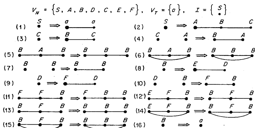
図 3. すべての分離不可能なウェーブを生成する \text{ncswg} の例。
