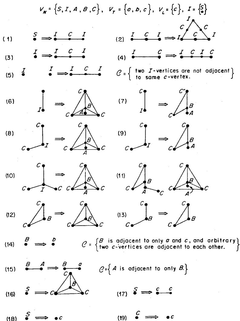
図 11. この適用条件を持つ nmc\ swg はすべてのライングラフを間接生成する。
