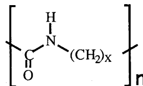
poly(lactam)
