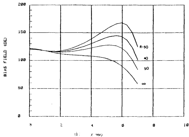
第6-17図 各条件における半円弧状永久磁石からの磁界分布
