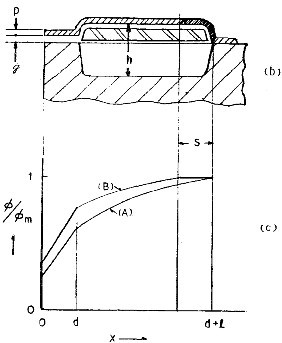
第5-10図 薄膜磁気ヘッドの構造と飽和モデル
