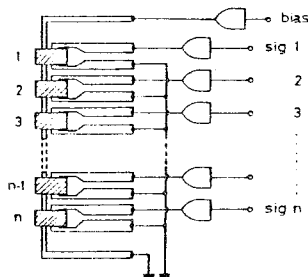
第4-16図 共通バイアス方式構成原理図
