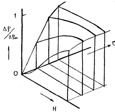
第 6-18 図 磁界と応力による強磁性体の抵抗変化
